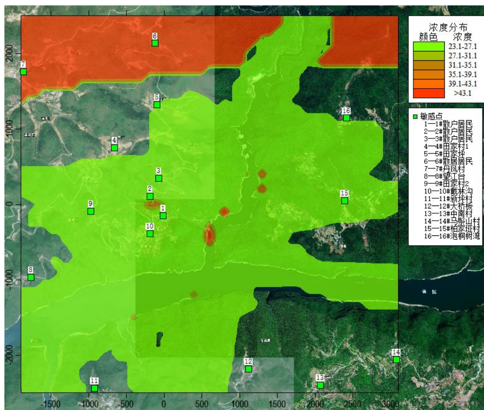
图 4.2-7 PM 2.5 叠加后保证率日平均质量浓度分布图（单位：μg/m 3 ）
