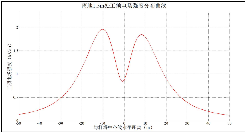
图 3-13 220kV 单回架空线路
