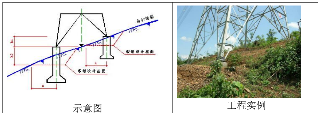
图5-1 铁塔全方位长短腿与不等高基础示意图及工程实例
