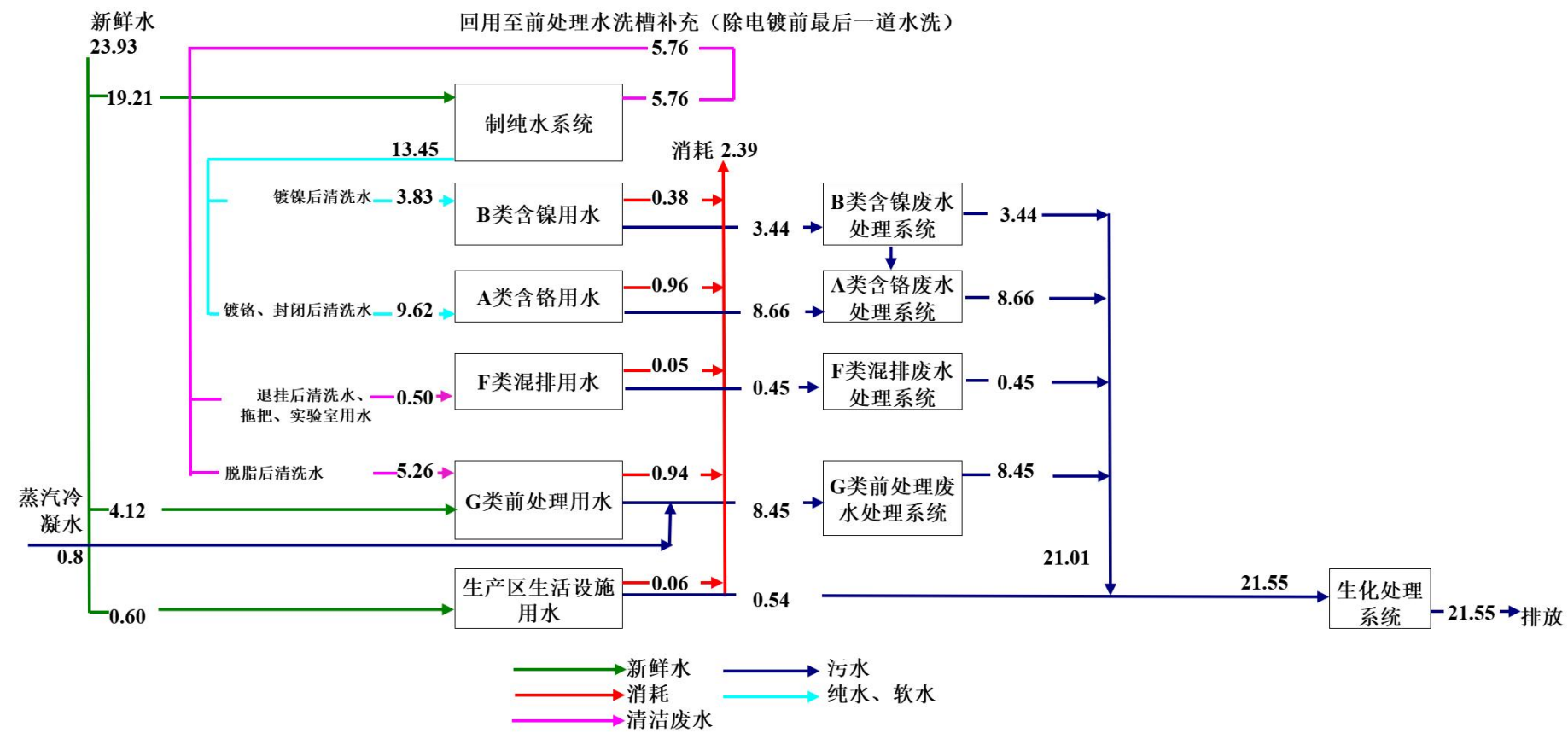
图 3.5-1 装饰铬表面处理生产线水平平衡图
