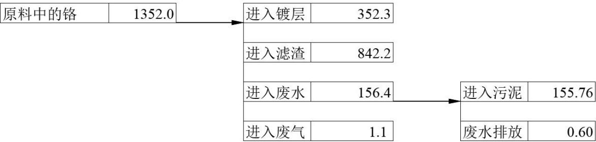
图 3.4-2 铬平衡图（单位：kg/a）
