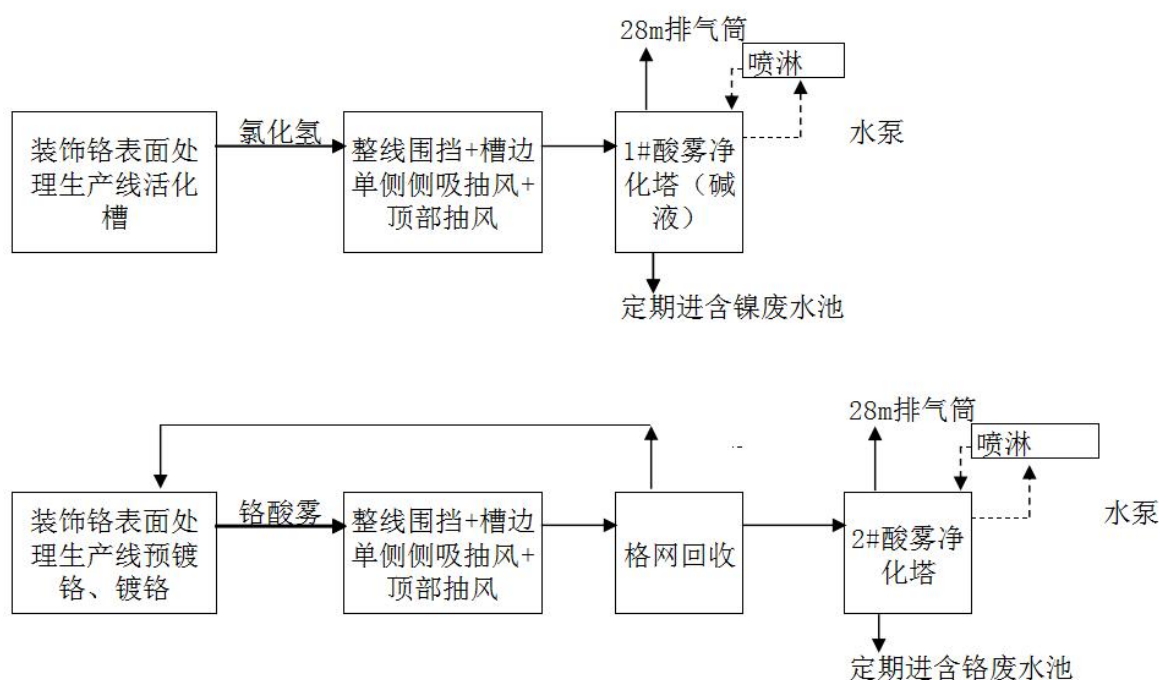
图 7.1-1 废气净化装置处理流程图
