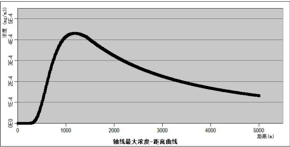
图 6.5-1 氯化氢轴线最大浓度分布图
