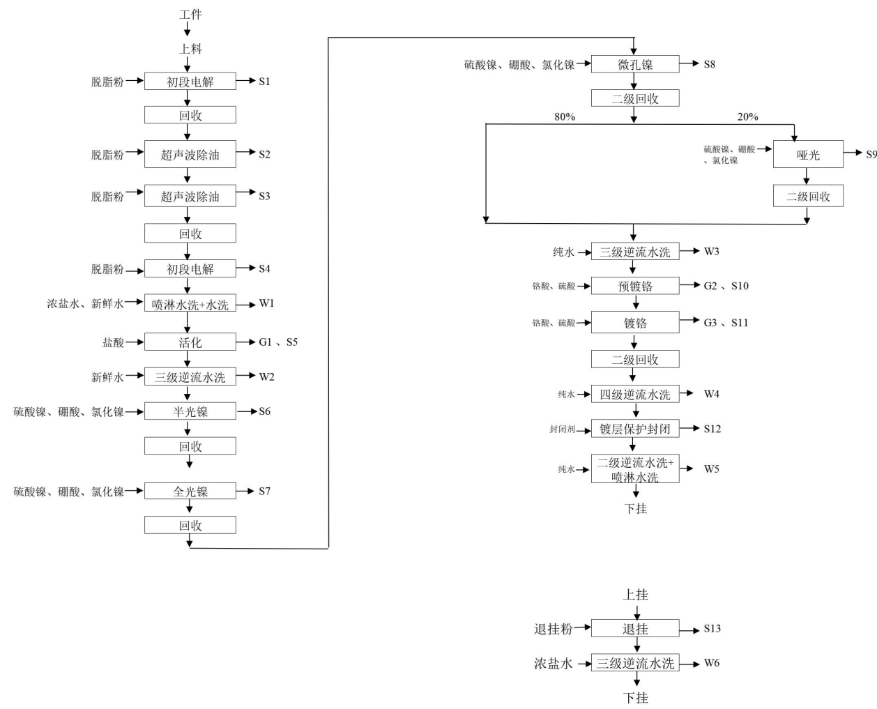
图 3.3-1 装饰铬表面处理生产线工艺流程及产污环节图
