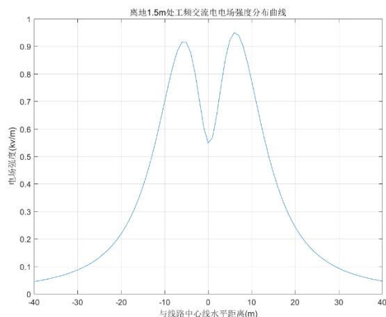
导线对地高度 10m 时地面 1.5m 电场强度水平分布图（kV/m） 导线对地高度 10m 时地面 1.5m 磁感应强度水平分布图（ \mu\text{T} ）
