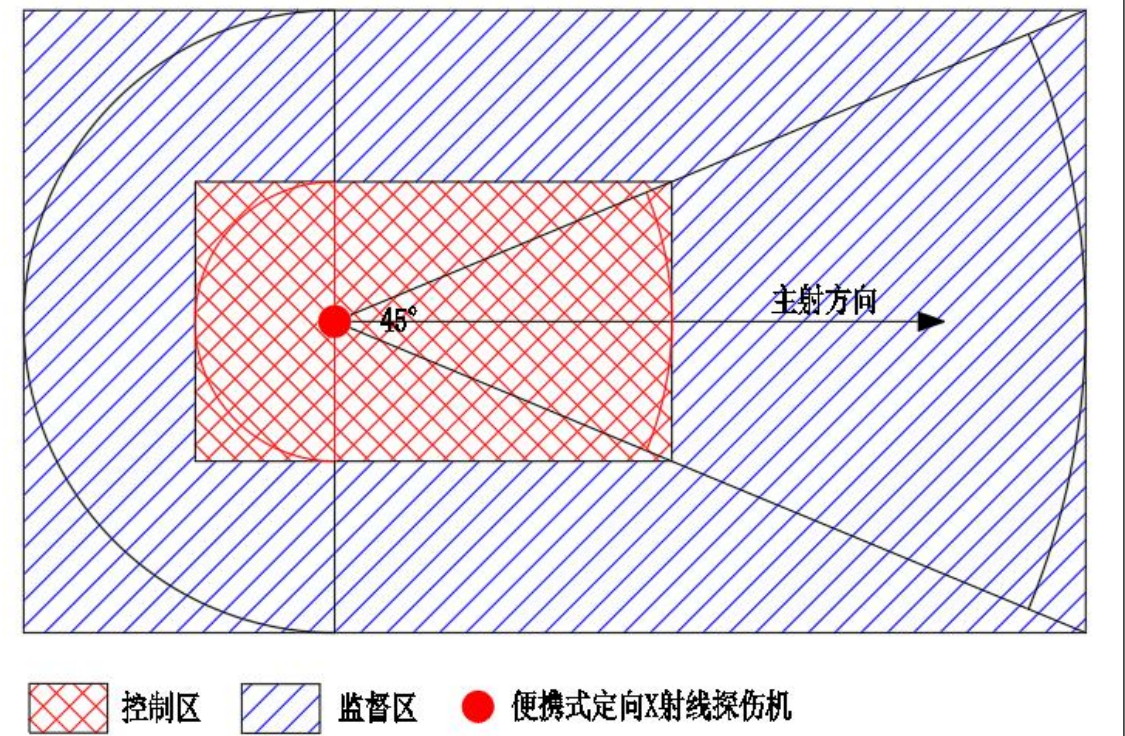
图 10-1 便携式定向 X 射线探伤机探伤现场地面控制区和监督区示意图
