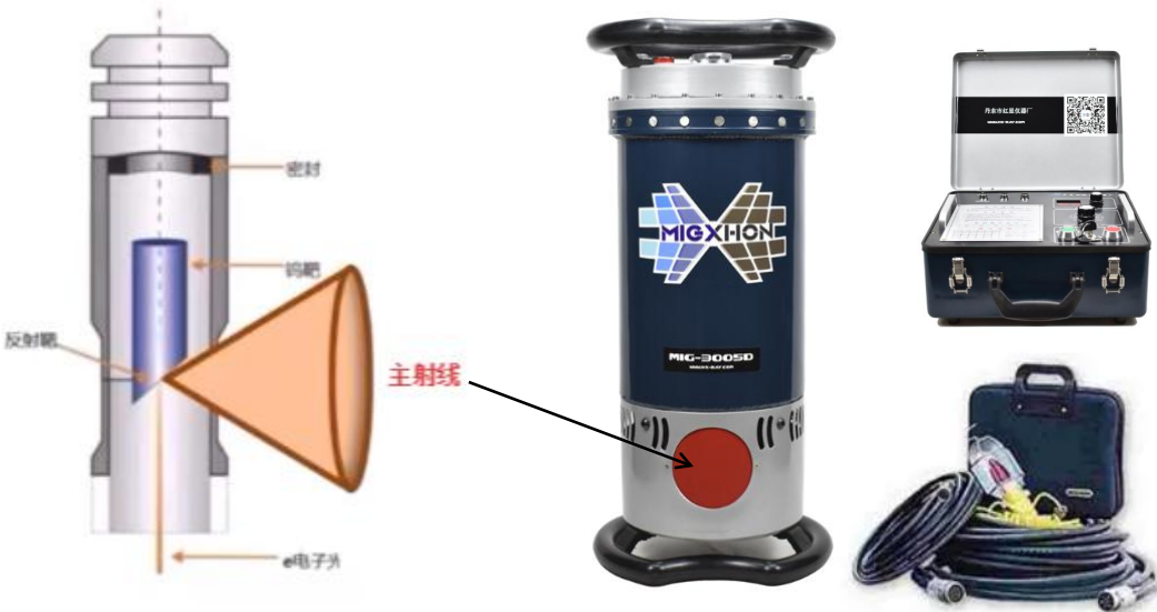
图 9-1 典型便携式 X 射线探伤机照片（左图为射线示意图）
