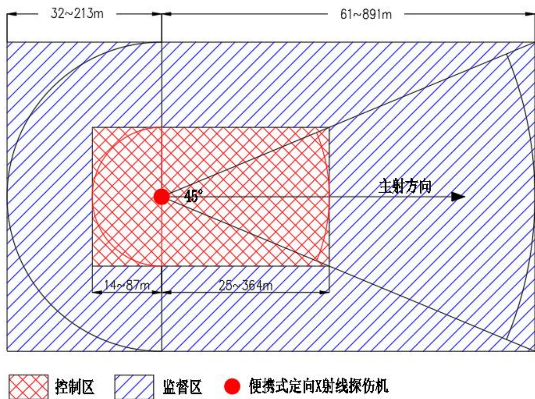
图 11-1 便携式定向 X 射线探伤机控制区、监督区划分示意图
