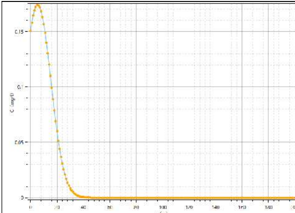
图 6.3.5-5 下游轴向铜浓度变化曲线（100d）
