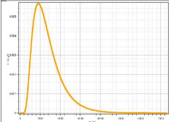
图 6.3.5-15 铜浓度随时间变化曲线 (x=60m)
