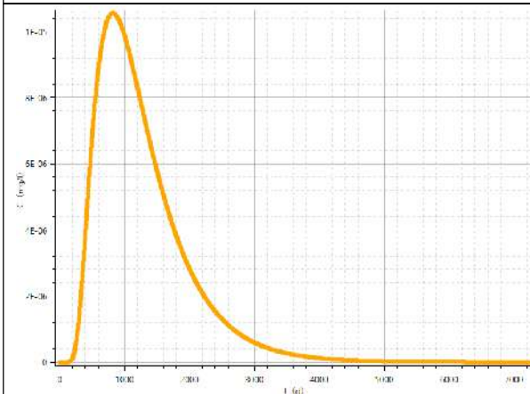
图 6.3.5-27 铜浓度随时间变化曲线（x=60m）
