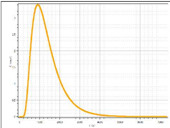
图 6.3.5-11 COD Mn 浓度随时间变化曲线 (x=60m)
