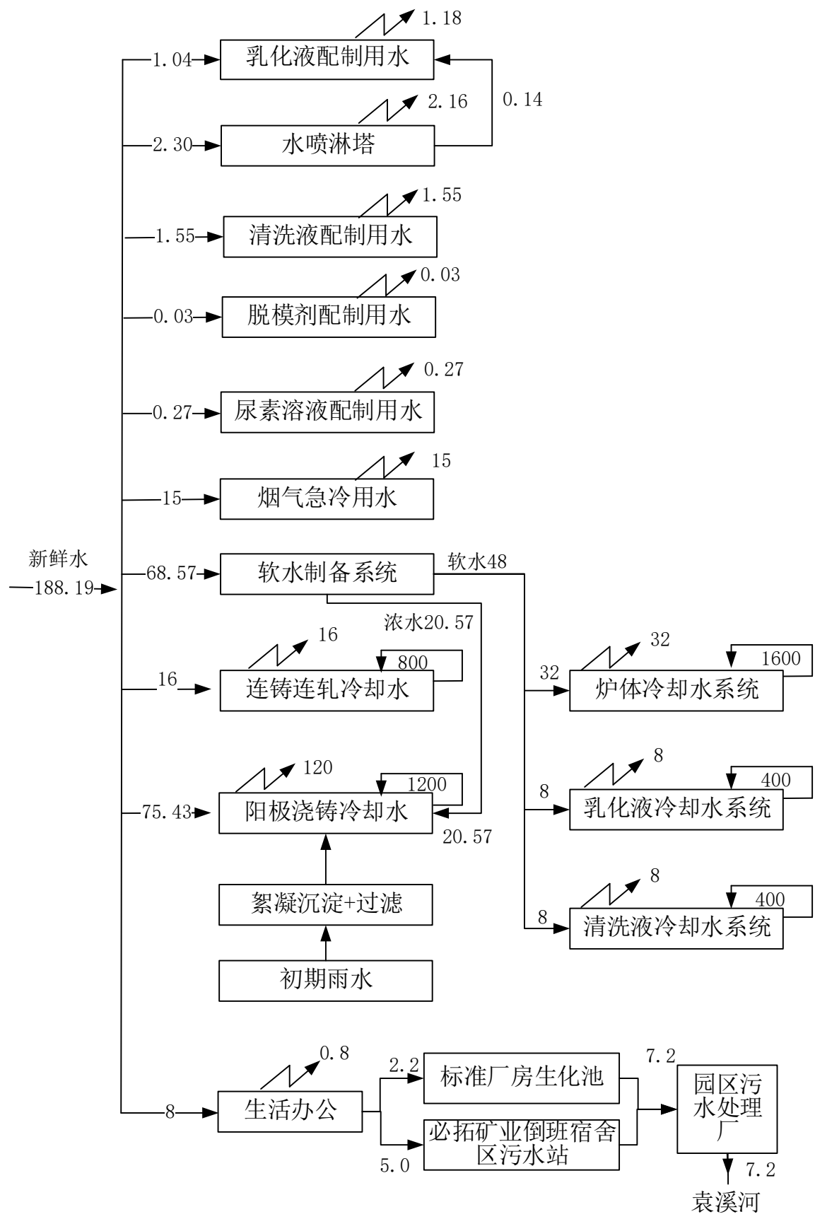
图3.2.5-1 本项目全厂水平衡图 (单位: \text{m}^3/\text{d} )
