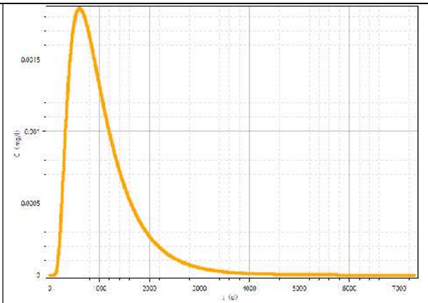
图 6.3.5-8 铜浓度随时间变化曲线 (y=15m)
