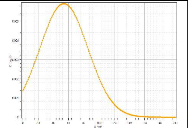
图 6.3.5-14 下游轴向铜浓度变化曲线 (1000d)
