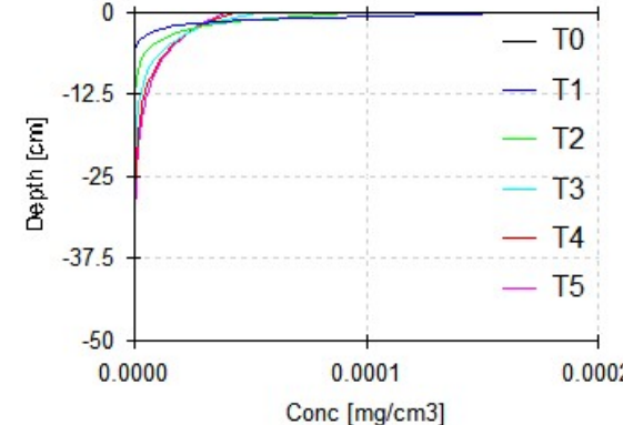
图 6.6.3-4 土壤中石油类浓度垂向深度变化图
