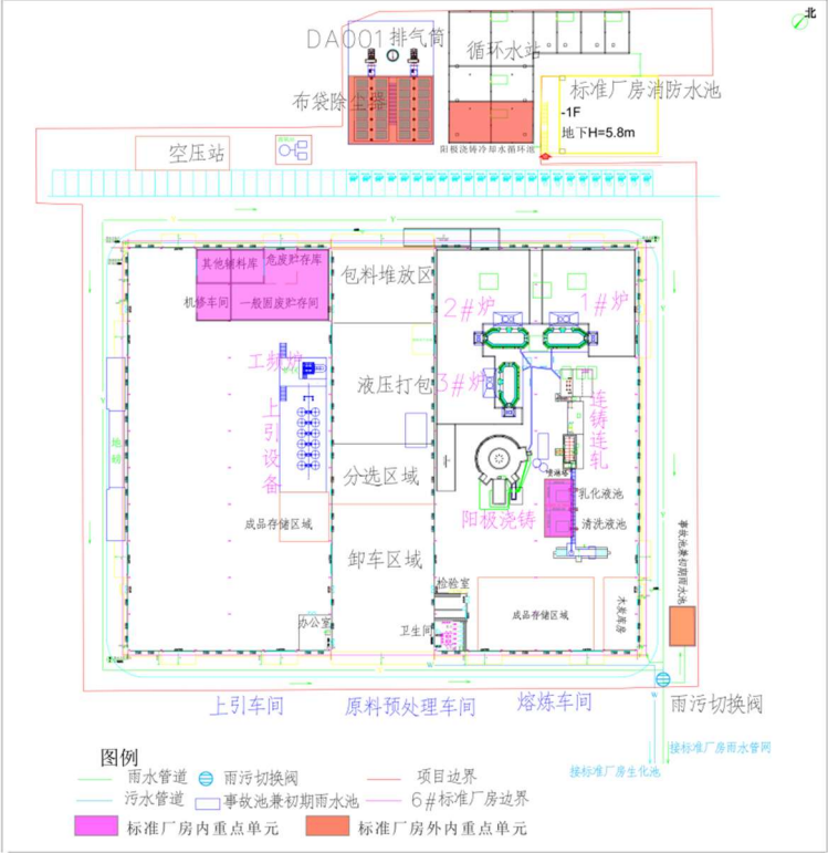
图 10.3.2-1 项目重点单元划分示意图
