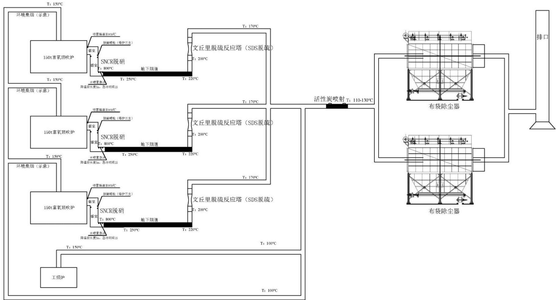
图 8.1-1 熔炼炉、工频炉废气处理走向示意图
