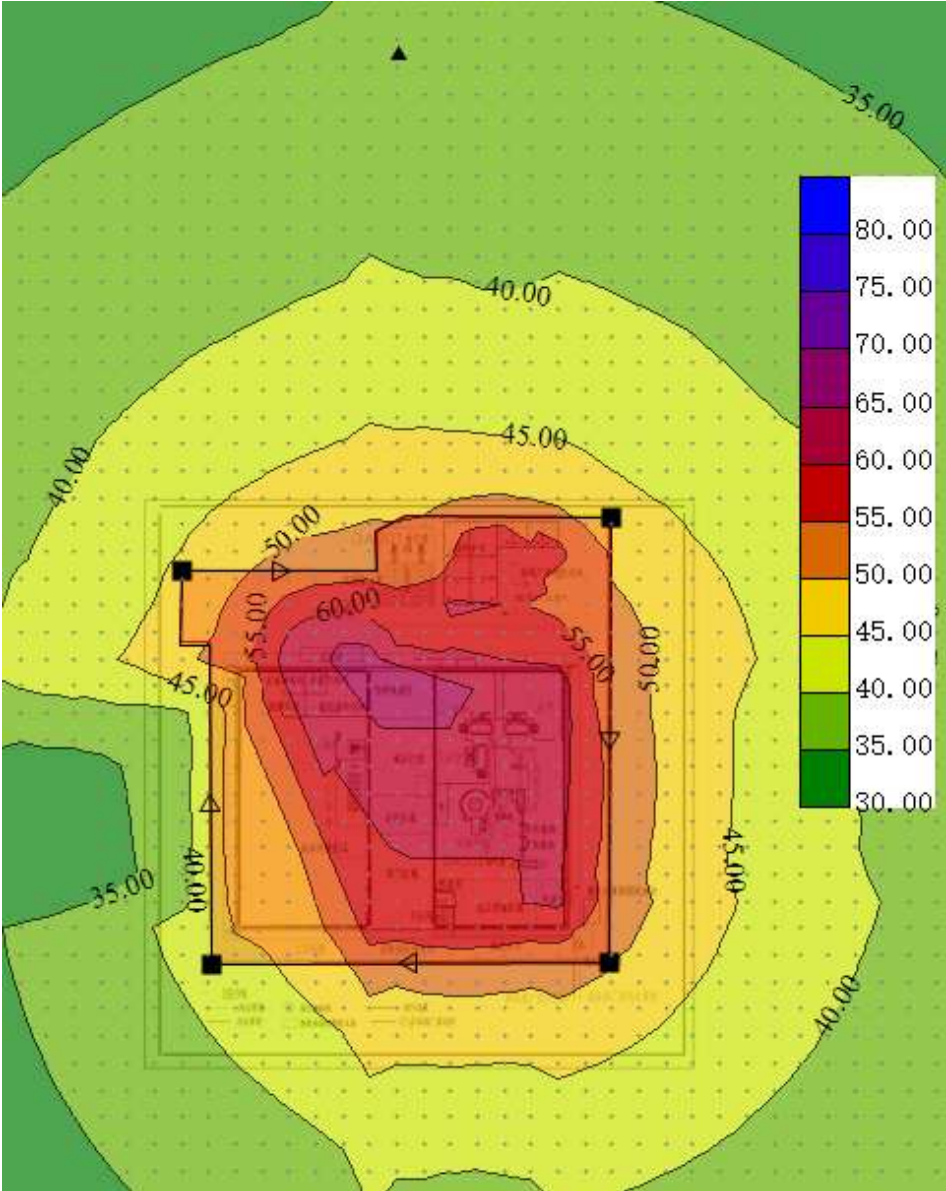
图 6.4.4-1 噪声贡献值等值线分布图
