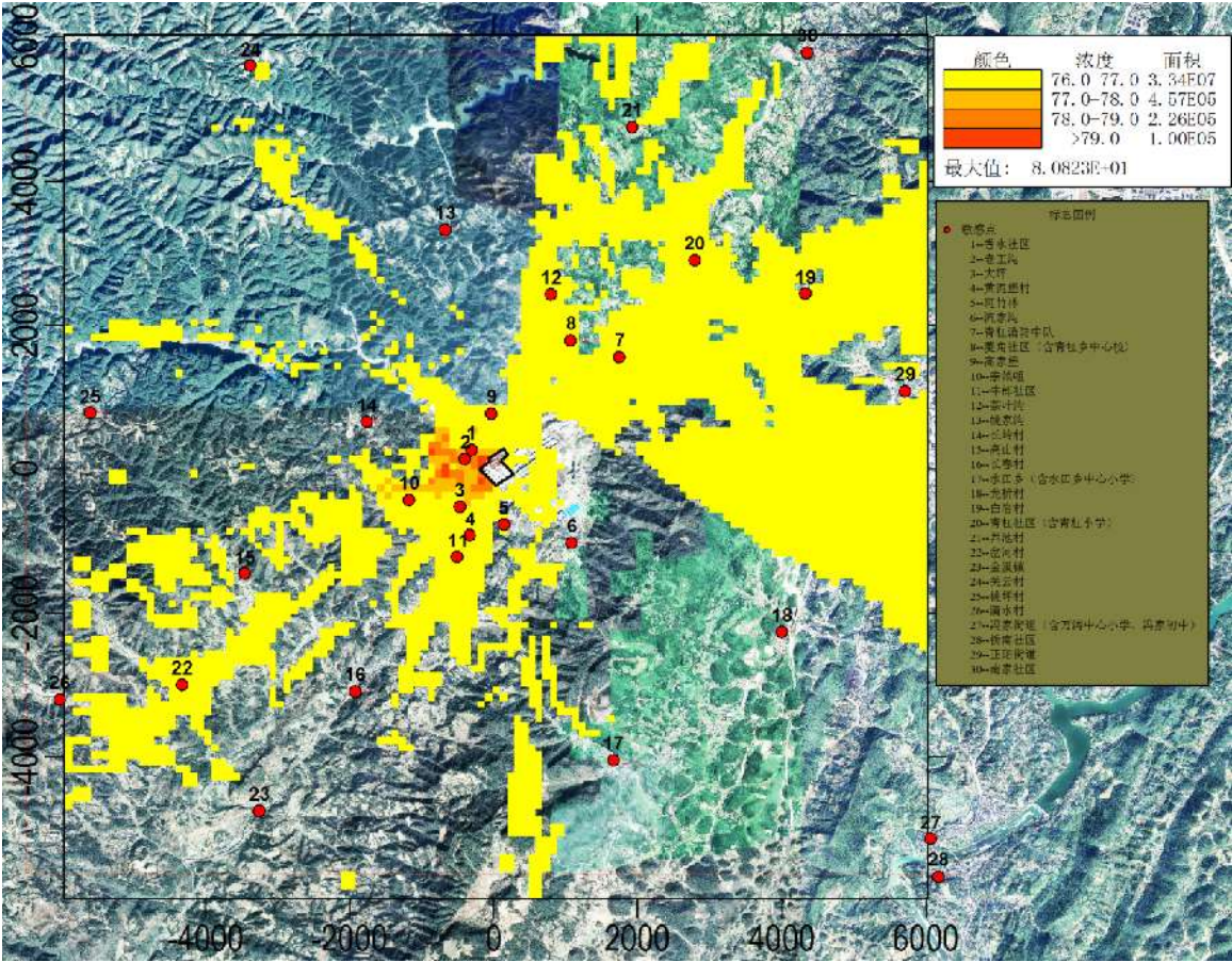
图 6.1.7-1 PM 10 日均叠加浓度分布图
