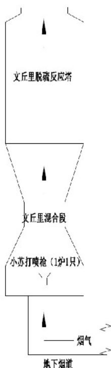
图 8.1.2-1 文丘里脱硫塔示意图
