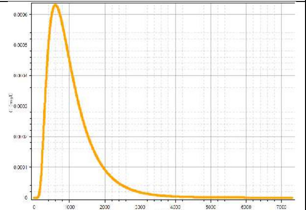
图 6.3.5-16 铜浓度随时间变化曲线 (y=15m)
