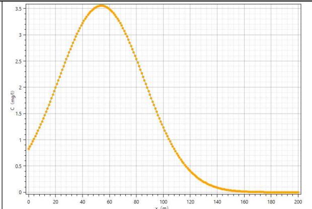
图 6.3.5-10 下游轴向 COD Mn 浓度变化曲线 (1000d)
