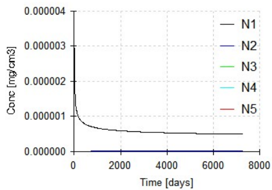
图 6.6.3-1 土壤中铜浓度随时间变化图
