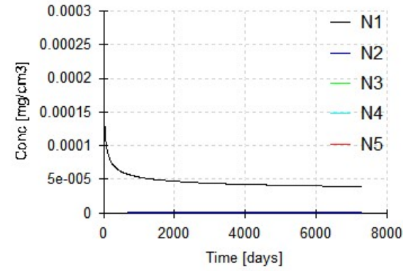
图 6.6.3-3 土壤中石油类浓度随时间变化图
