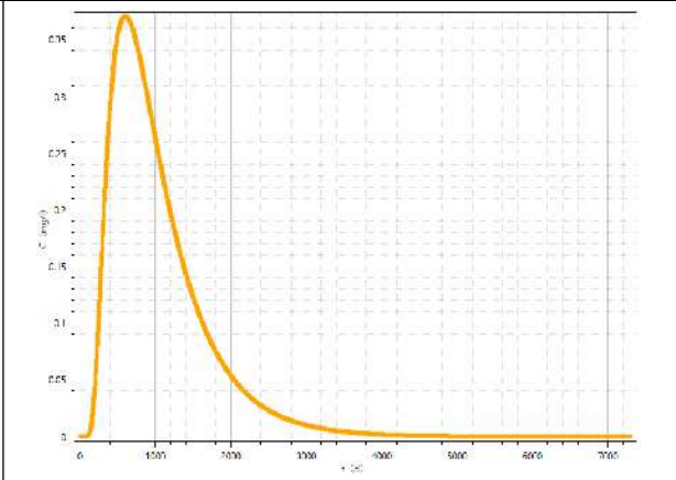
图 6.3.5-4 COD Mn 浓度随时间变化曲线（y=15m）
