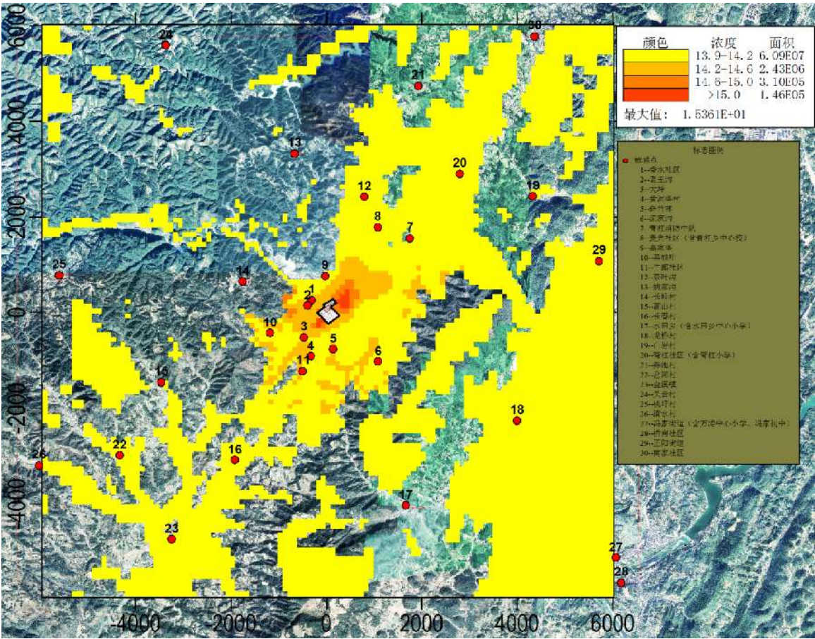
图 5.1.7-8 NO 2 年均叠加浓度分布图
