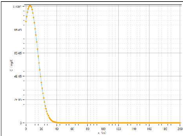
图 6.3.5-25 下游轴向铜浓度变化曲线（100d）
