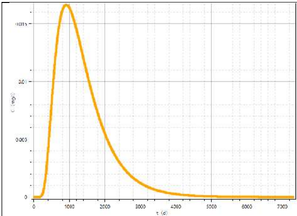
图 6.3.5-7 铜浓度随时间变化曲线 (x=65m)
