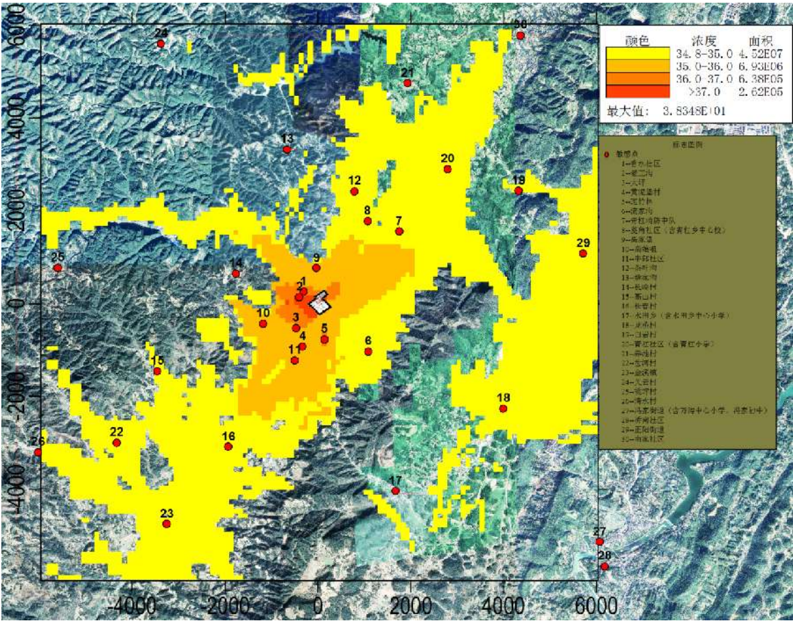
图 6.1.7-2 PM 10 年均叠加浓度分布图
