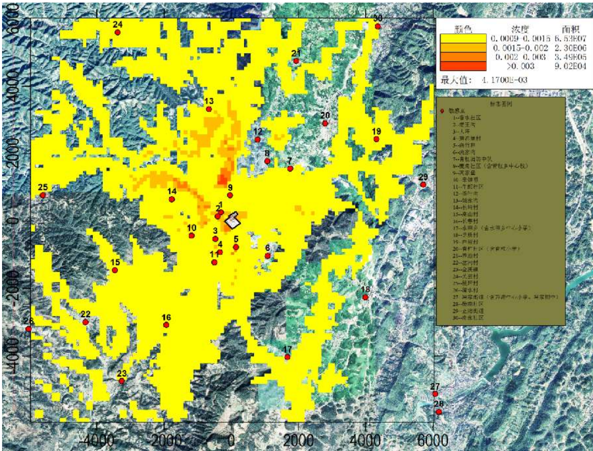
图 6.1.7-11 砷及其化合物日均叠加浓度分布图
