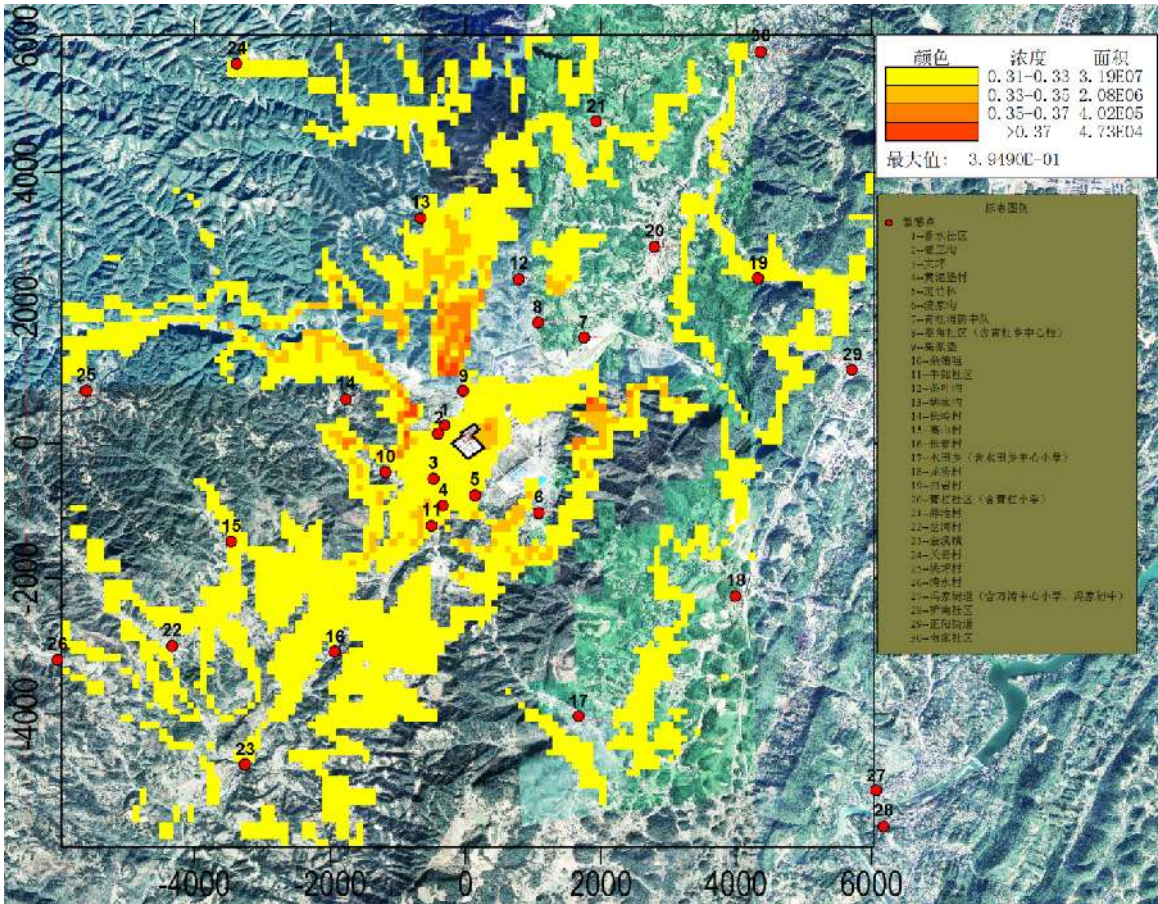
图 6.1.7-12 二噁英日均叠加浓度分布图
