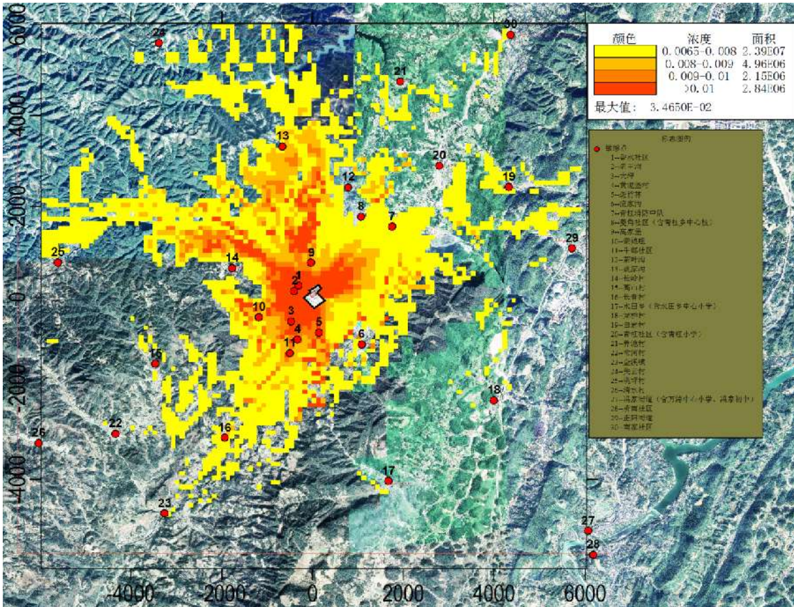
图 6.1.7-9 铅及其化合物日均叠加浓度分布图
