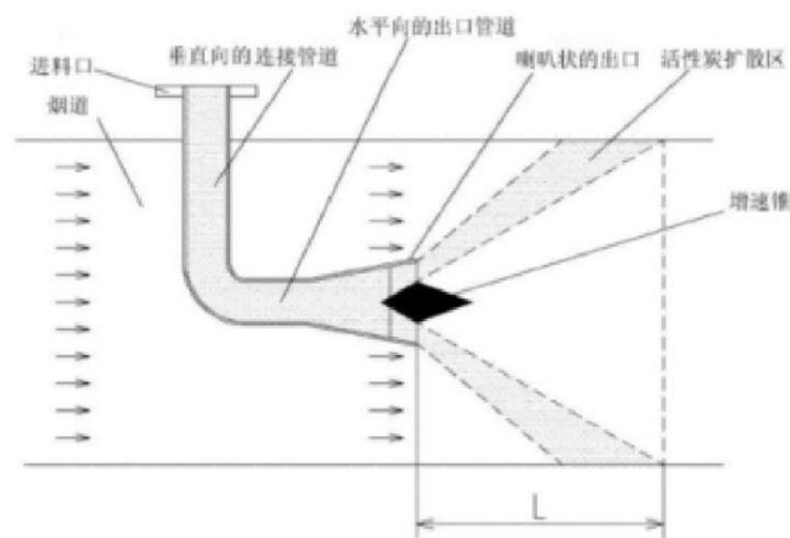
图 8.1.4-2 活性炭喷射装置结构示意图
