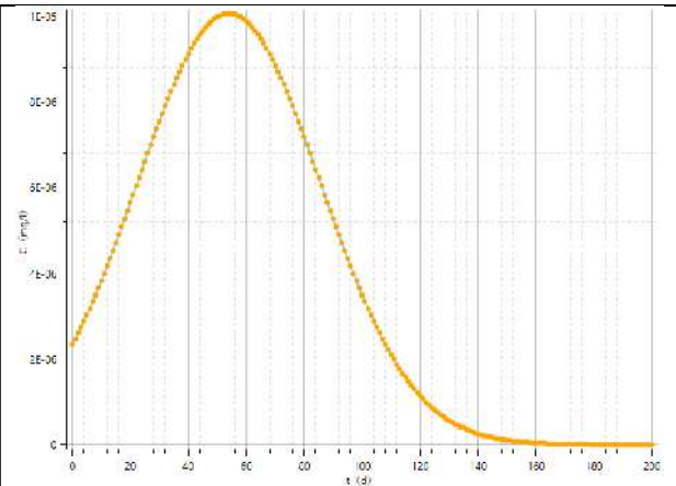
图 6.3.5-26 下游轴向铜浓度变化曲线（1000d）
