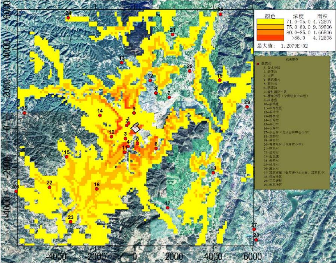
图 6.1.7-14 氨小时叠加浓度分布图
