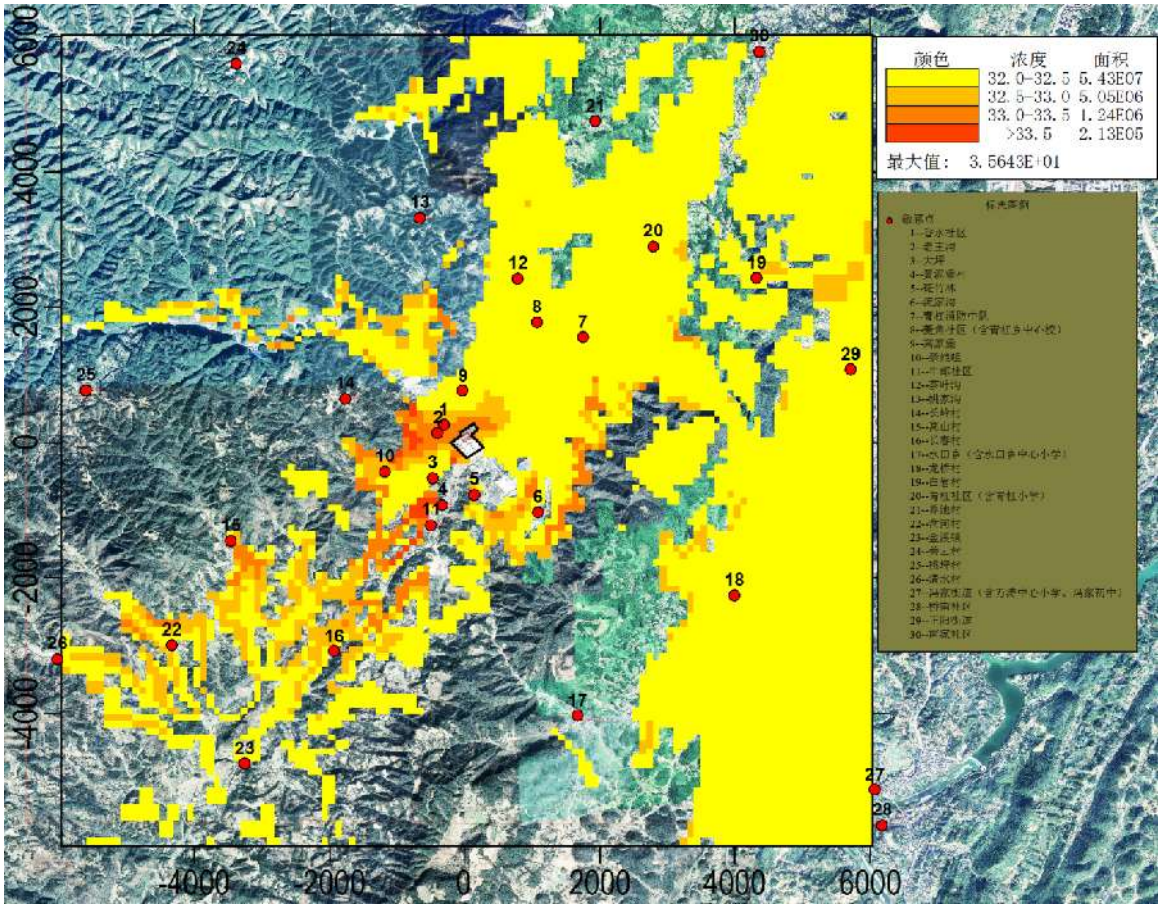
图 5.1.7-7 NO 2 日均叠加浓度分布图
