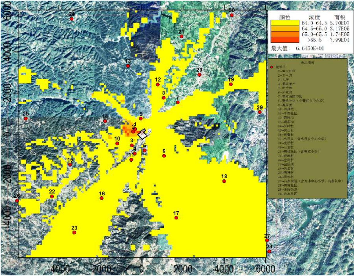
图 6.1.7-3 PM 2.5 日均叠加浓度分布图
