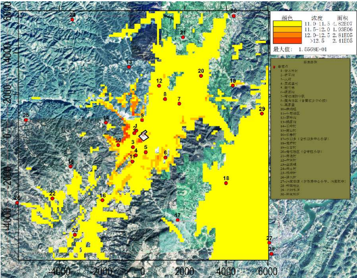
图 6.1.7-5 SO 2 日均叠加浓度分布图
