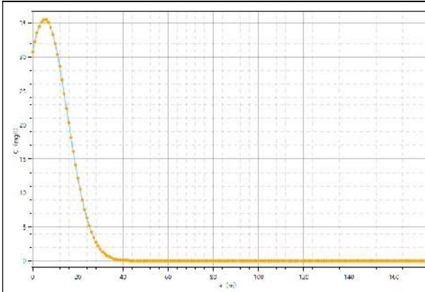
图 6.3.5-9 下游轴向 COD Mn 浓度变化曲线 (100d)
