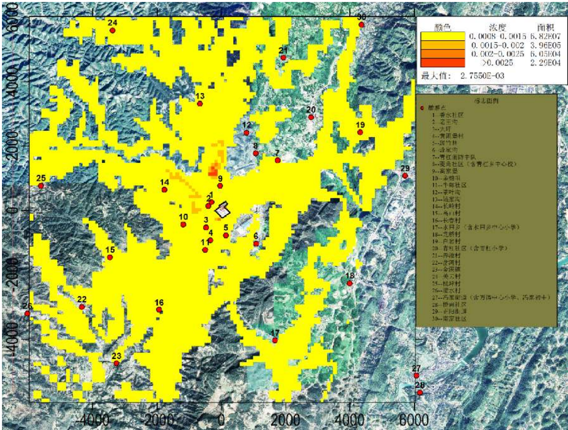
图 6.1.7-10 镉及其化合物日均叠加浓度分布图
