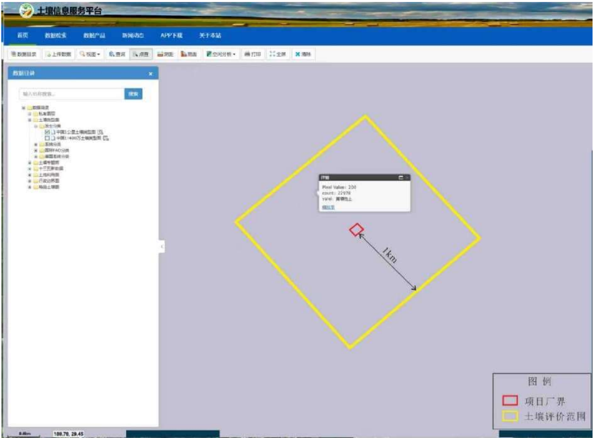
图 4.5.2-1 项目所在区域土壤类型分布图
