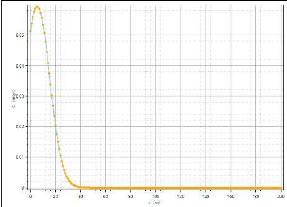
图 6.3.5-13 下游轴向铜浓度变化曲线 (100d)
