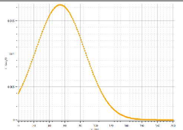
图 6.3.5-6 下游轴向铜浓度变化曲线（1000d）
