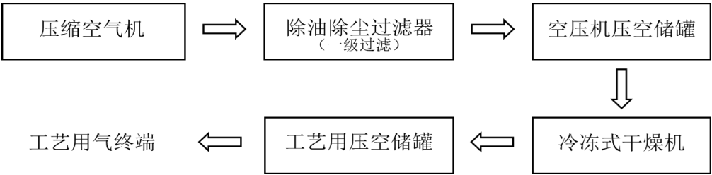
图 3.10-1 压缩空气系统工艺流程图
