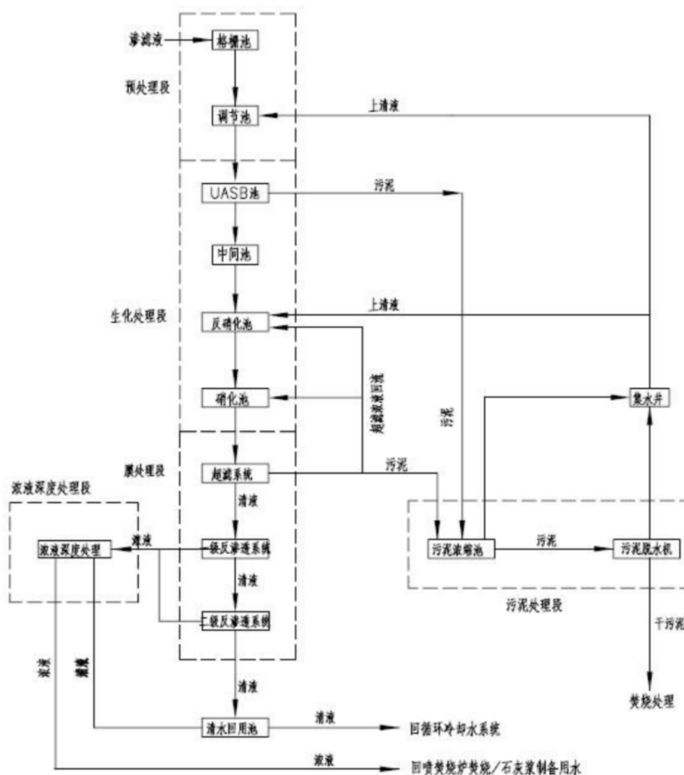
图 2.4-1 污水处理站（综合废水处理站）工艺流程图
