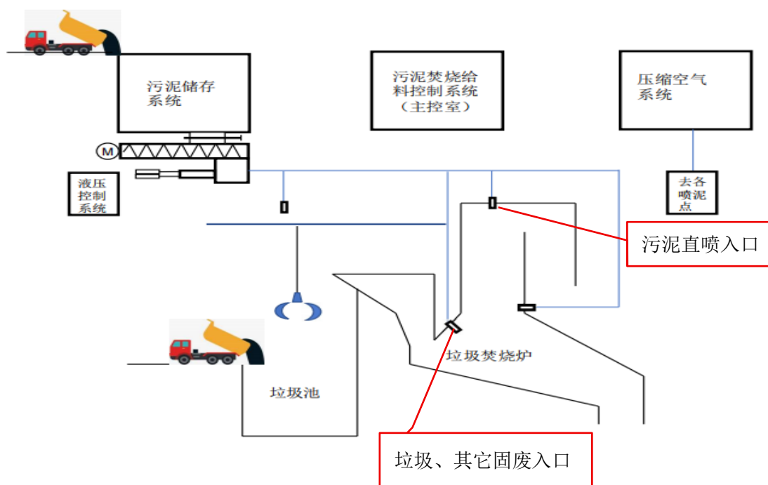
图 3.11-3 污泥直喷系统示意图
