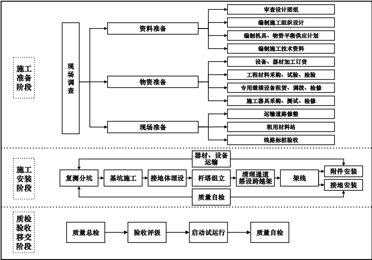
图3.1-3 本项目线路施工工艺流程图
