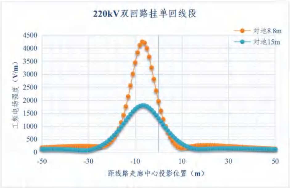
图 6.1-13 220kV 双回路挂单回线路导线对地不同高度时地面 1.5m 处工频电场强度变化趋势
