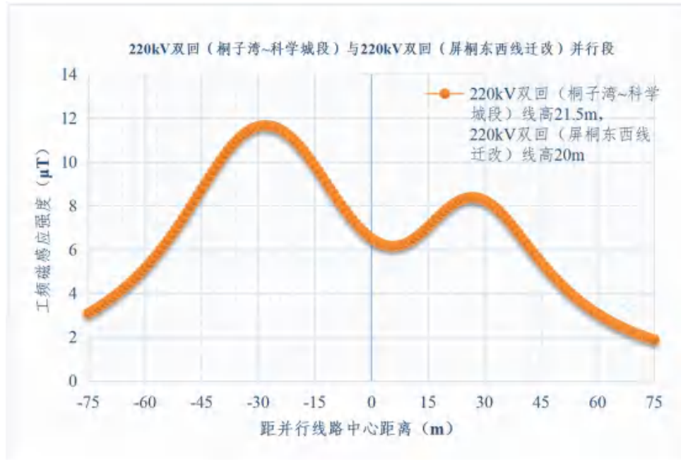
图6.1-46 220kV 双回（桐子湾~科学城段）与220kV 双回（屏桐东西线迁改）并行段地面1.5m 处产生工频磁感应强度变化趋势
