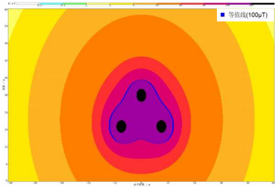
图 6.1-36 500kV 单回架空线路导线对地高度 19m 工频磁感应强度空间分布图
