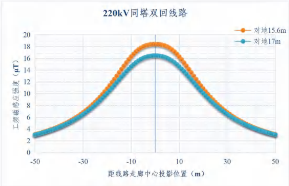
图 6.1-22 220kV 同塔双回线路（桐子湾~科学城段）不同对地高度时地面 1.5m 处工频磁感应强度变化趋势
