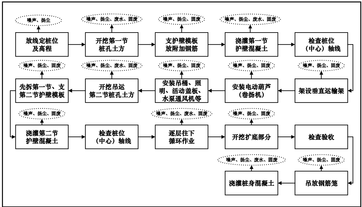
图 3.1-4 挖孔基础施工流程图
