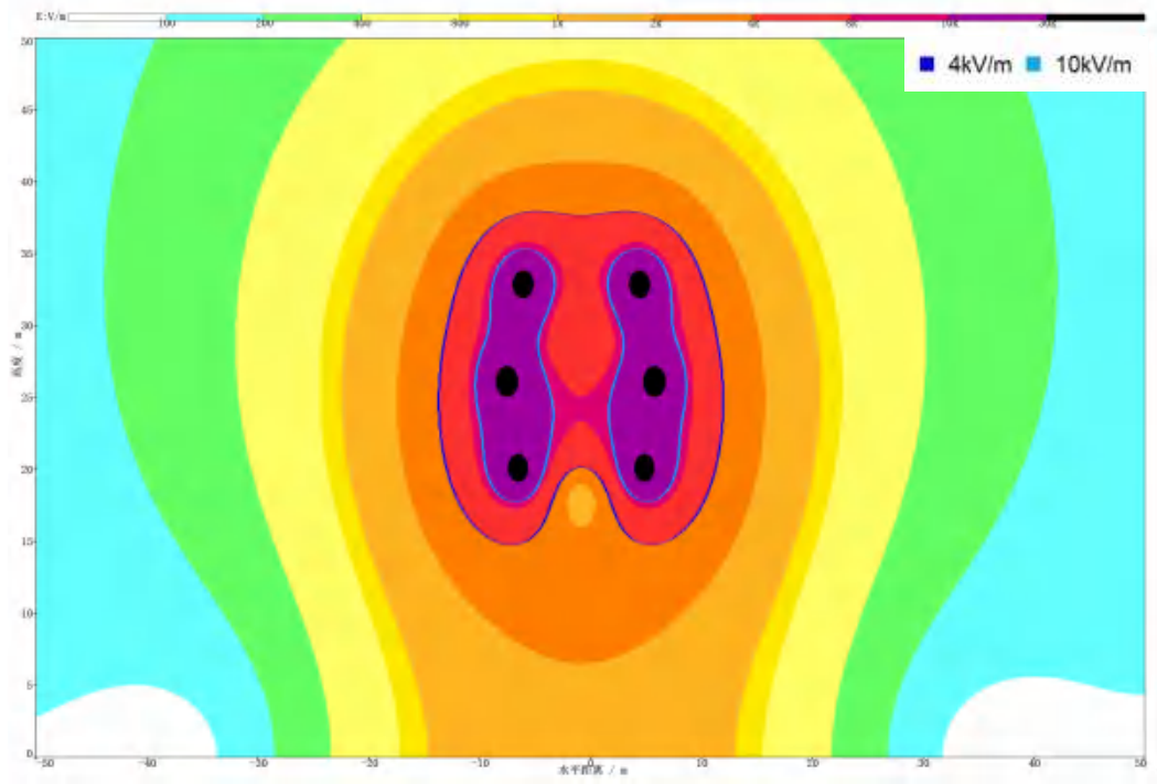
图 6.1-27 220kV 同塔双回（220kV 屏桐东西线迁改段）导线对地高度 20m 工频电场强度空间分布图
