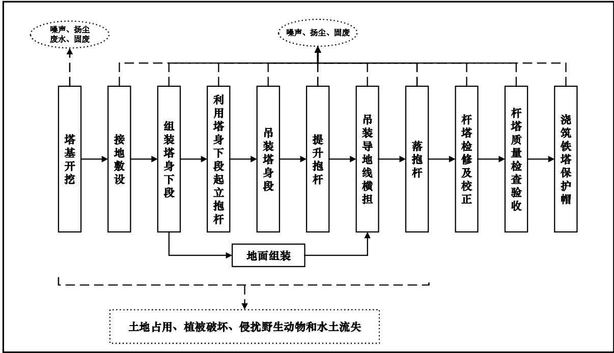
图3.1-7 铁塔组立施工流程图
