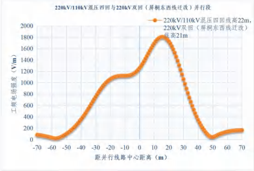
图 6.1-48 220kV/110kV 混压四回与 220kV 双回（屏桐东西线迁改）并行段 地面 1.5m 处工频电场强度变化趋势
