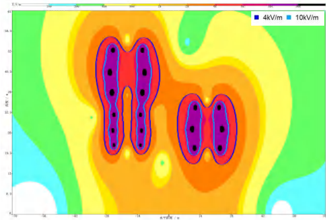
图 6.1-50 220kV/110kV 混压四回与 220kV 双回（屏桐东西线迁改）并行段工频电场强度空间分布图
