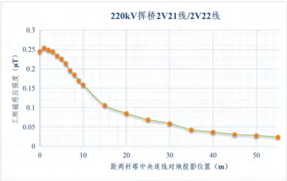
图 6.1-5 220kV 挥桥 2V21 线/2V22 线双回线路工频磁感应强度随距离的变化趋势
