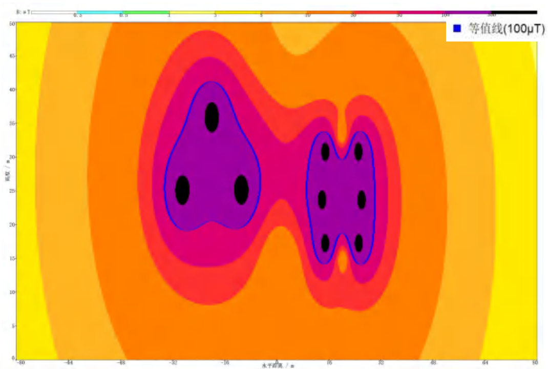
图 6.1-40 500kV 单回架空线路与 220kV 同塔双回架空线路并行段工频磁感应强度空间分布图
