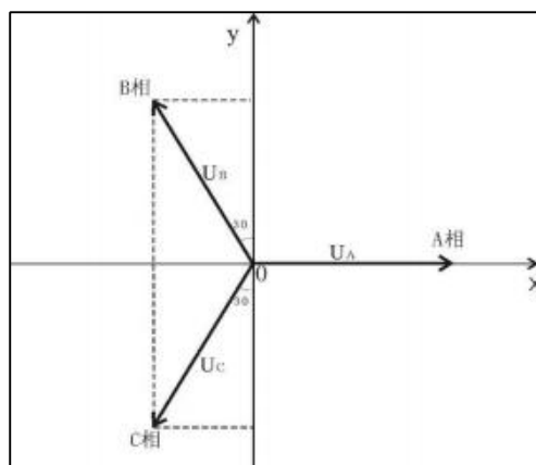
图 6.1-10 对地电压计算图
