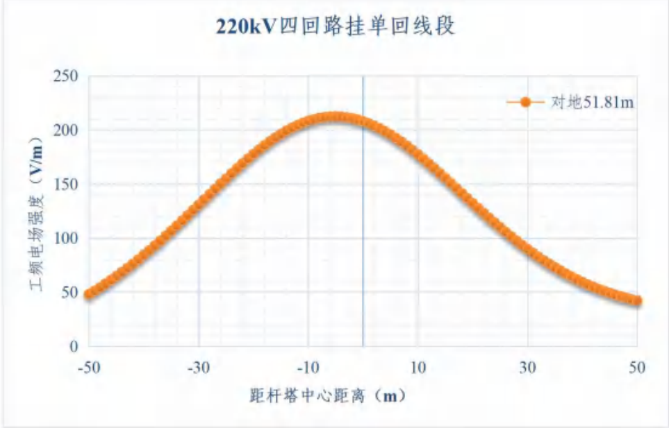
图 6.1-17 220kV 四回路挂单回线路导线对地 51.8m 地面 1.5m 处工频电场强度变化趋势
