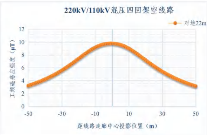
图6.1-30 220kV/110kV 混压四回架空线路导线对地高度22m 时地面1.5m 处 工频磁感应强度变化趋势
