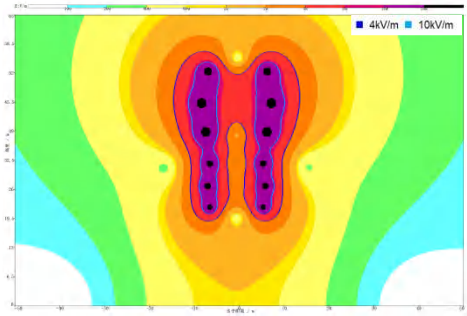
图 6.1-31 220kV/110kV 混压四回架空路导线对地高度 22m 工频电场强度空间分布图
