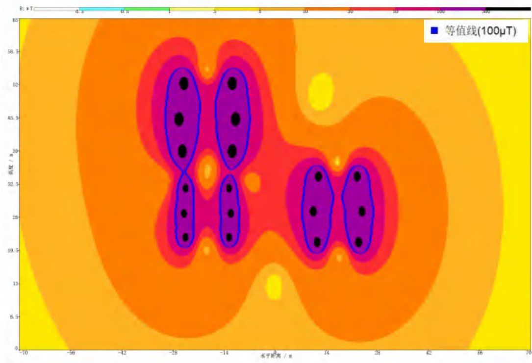
图 6.1-51 220kV/110kV 混压四回与 220kV 双回（屏桐东西线迁改）并行段工频磁感应强度空间分布图
