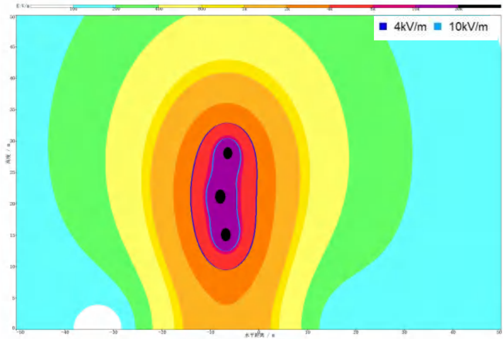
图 6.1-15 220-GB21S-JC4 塔型导线对地 15m 工频电场强度空间分布图
