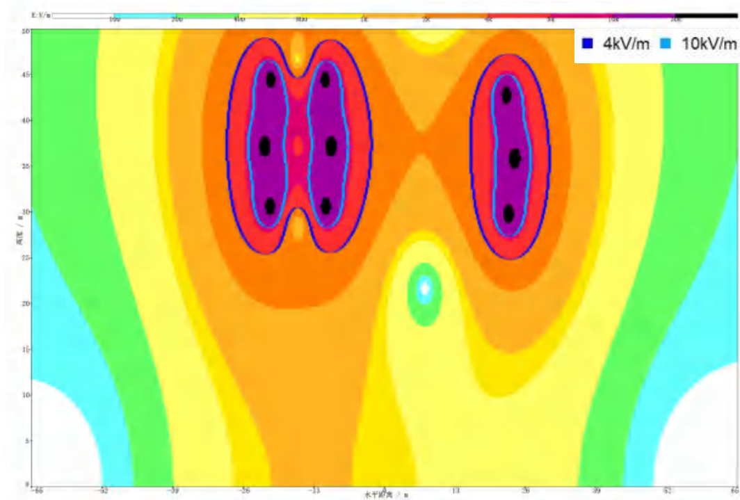
图 6.1-43 220kV 双回（桐子湾~科学城段）与 220kV 双回路挂单回线并行段工频电场强度空间分布图
