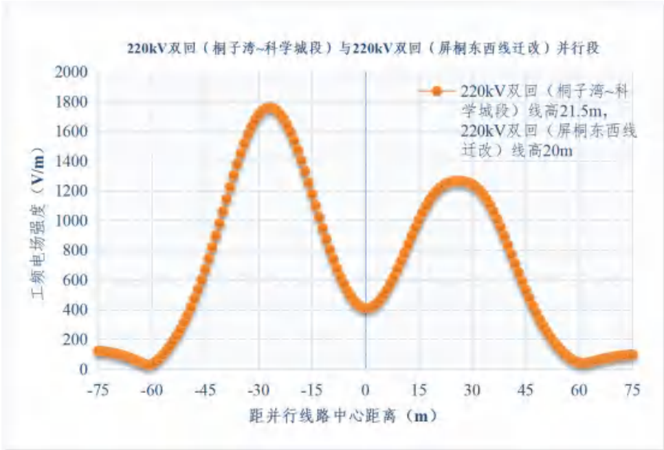
图 6.1-45 220kV 双回（桐子湾~科学城段）与 220kV 双回（屏桐东西线迁改）并行段 地面 1.5m 处工频电场强度变化趋势
