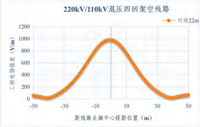
图 6.1-29 220kV/110kV 混压四回架空线路导线对地高度 22m 时地面 1.5m 处 工频电场强度变化趋势
