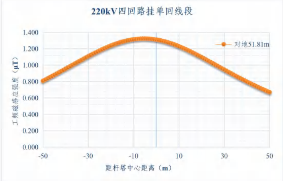
图 6.1-18 220kV 四回路挂单回线路导线对地 51.8m 地面 1.5m 处工频磁感应强度变化趋势
