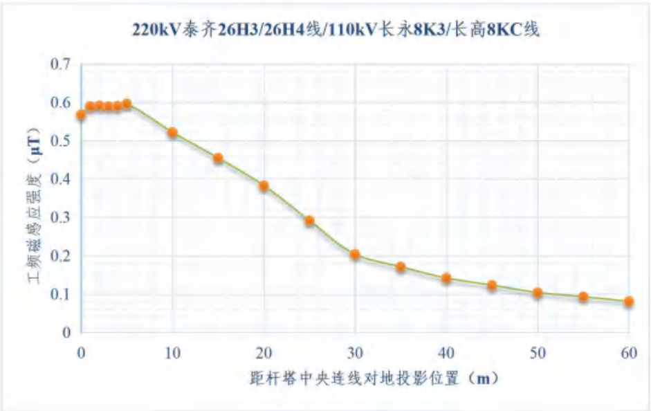
图 6.1-7 220kV 泰齐 26H3/26H4 线/110kV 长永 8K3/长高 8KC 线工频磁感应强度随距离的变化趋势
