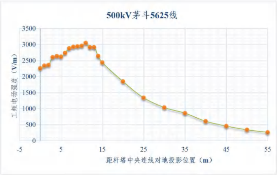
图 6.1-2 500kV 茅斗 5265 线工频电场强度随距离的变化趋势
