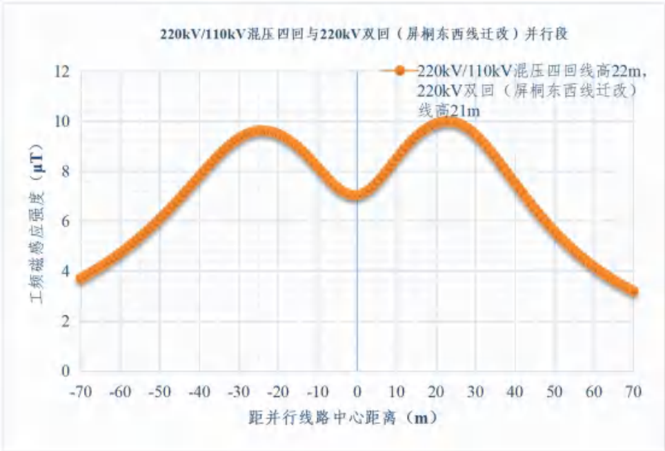
图6.1-49 220kV/110kV 混压四回与220kV 双回（屏桐东西线迁改）并行段 地面1.5m 处产生工频磁感应强度变化趋势
