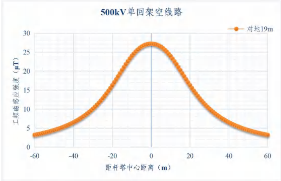
图6.1-34 500kV 单回架空线路导线对地高度19m 时地面1.5m 处工频磁感应强度变化趋势
