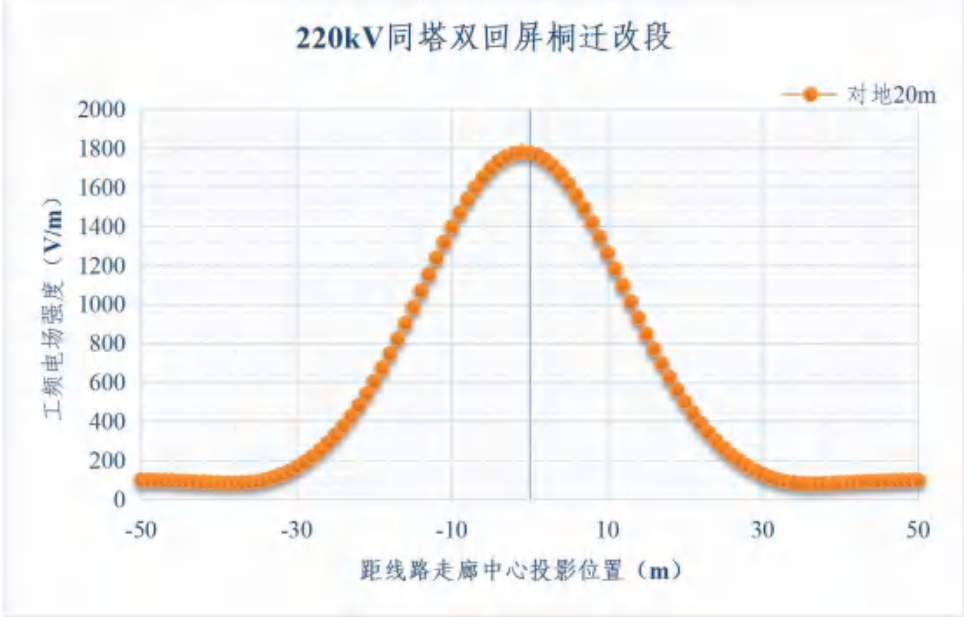
图 6.1-25 220kV 同塔双回（220kV 屏桐东西线迁改段）导线对地高度 20m 时 1.5m 处工频电场强度变化趋势
