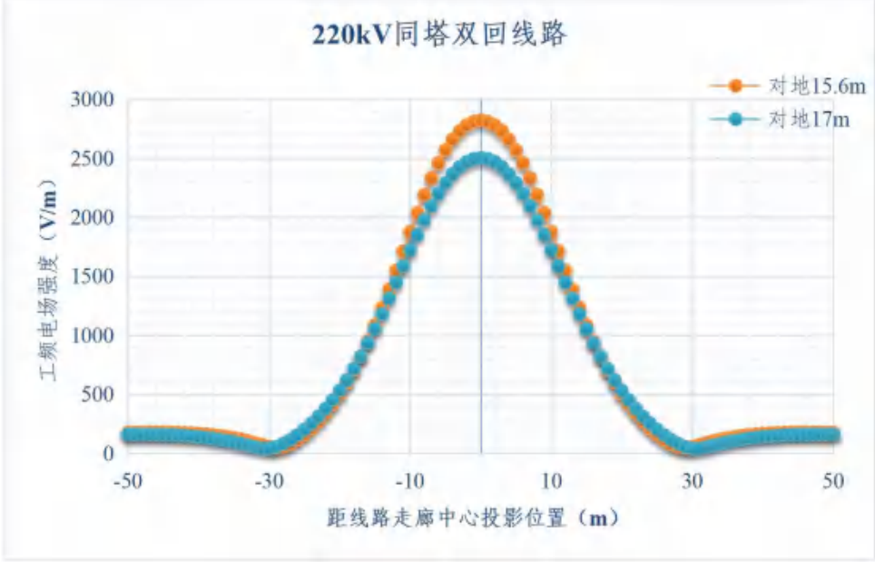
图 6.1-21 220kV 同塔双回线路（桐子湾~科学城段）不同对地高度时地面 1.5m 处工频电场强度变化趋势
