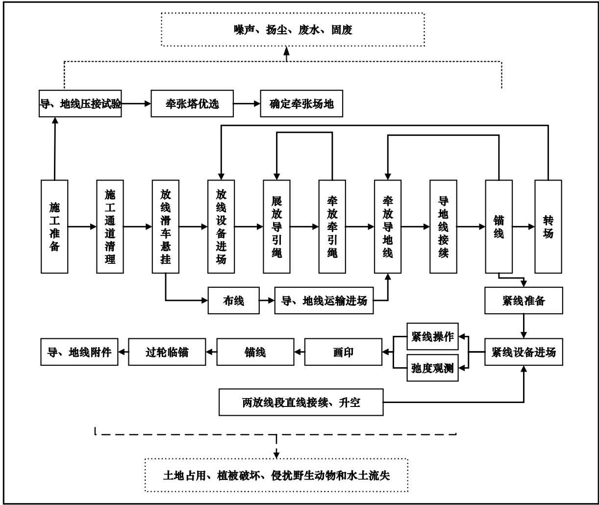
图3.1-8 架线施工流程图
