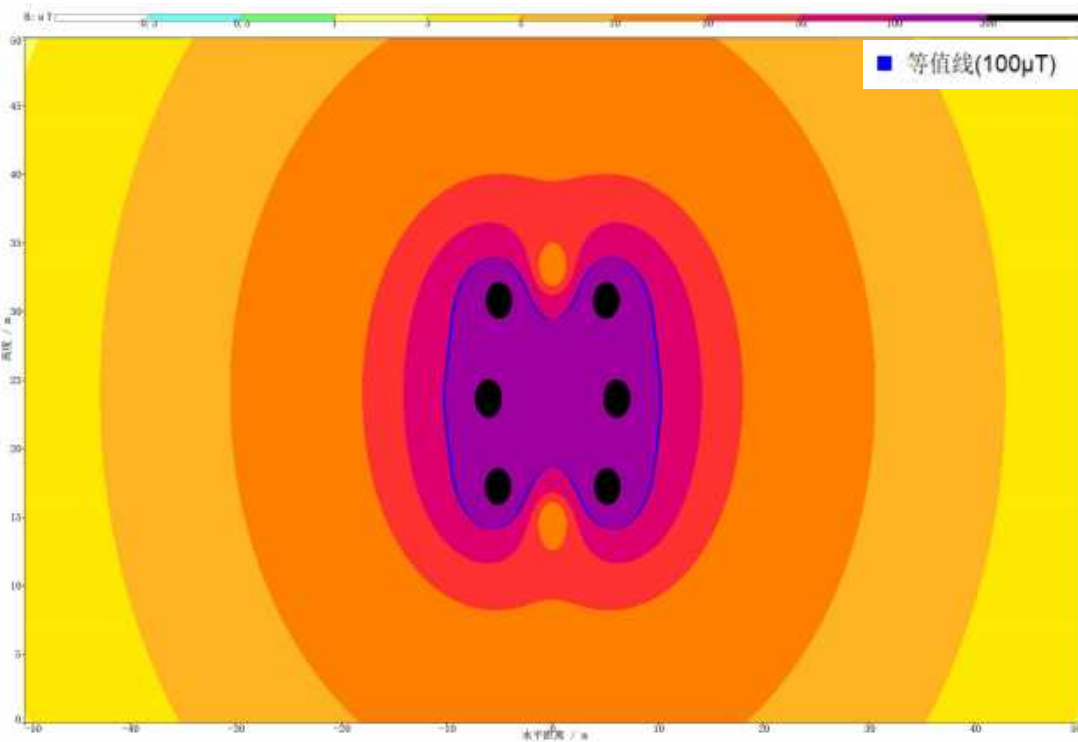
图 6.1-24 220kV 同塔双回线路（桐子湾~科学城段）导线对地 17m 工频磁感应强度空间分布图
