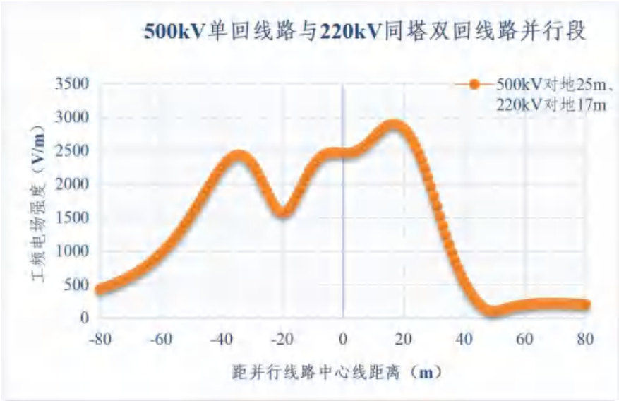
图 6.1-37 500kV 单回架空线路与 220kV 同塔双回架空线路并行段地面 1.5m 处 工频电场强度变化趋势
