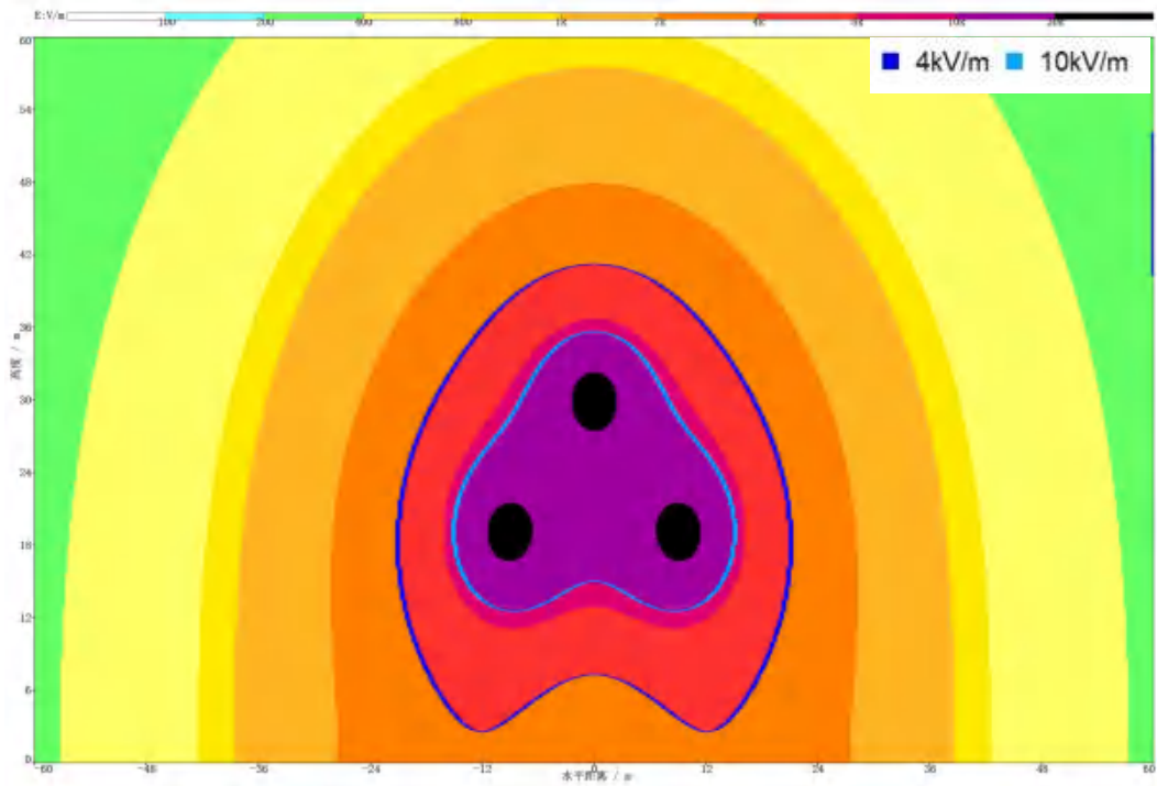
图 6.1-35 500kV 单回架空线路导线对地高度 19m 工频电场强度空间分布图
