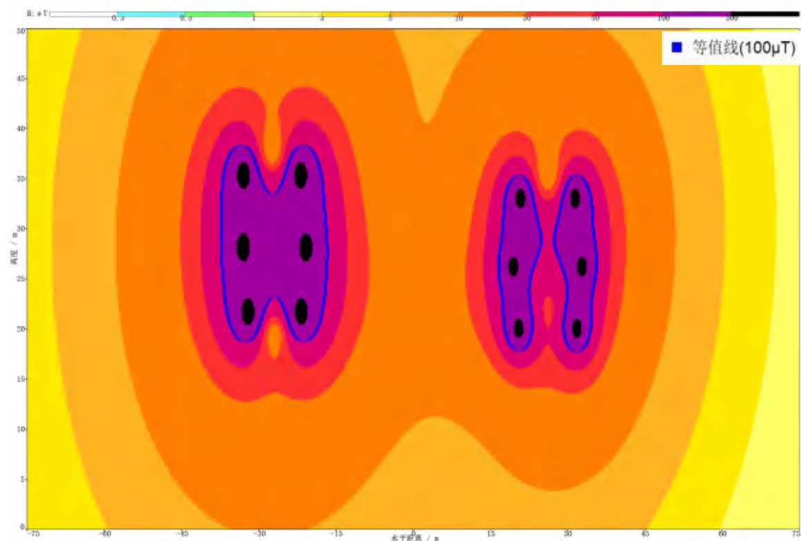
图 6.1-48 220kV 双回（桐子湾~科学城段）与 220kV 双回（屏桐东西线迁改）并行段工频磁感应强度空间分布图
