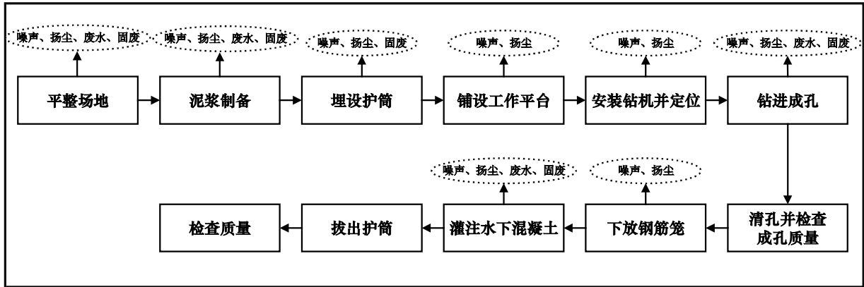
图 3.1-5 灌注桩施工流程图
