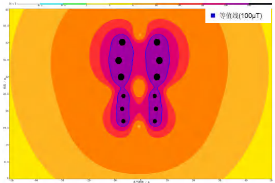
图 6.1-32 220kV/110kV 混压四回架空路导线对地高度 22m 工频磁感应强度空间分布图
