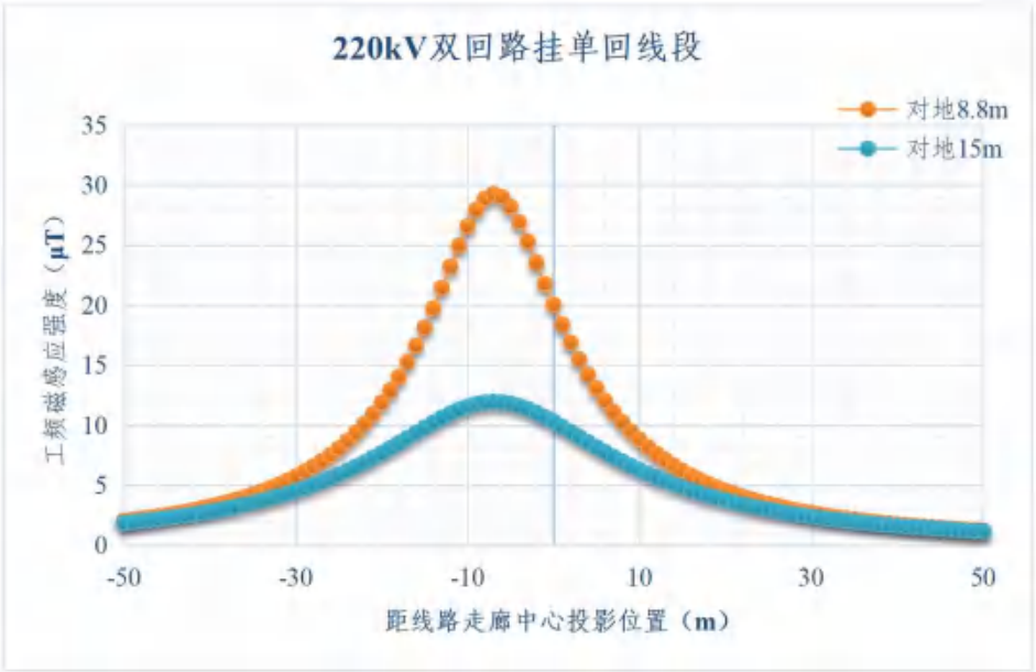
图 6.1-14 220kV 双回路挂单回线路导线对地不同高度时地面 1.5m 处工频磁感应强度变化趋势
