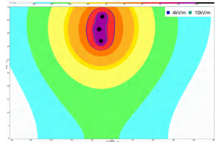
图 6.1-19 220kV 四回路挂单回线路导线对地 51.8m 时工频电场强度空间分布图
