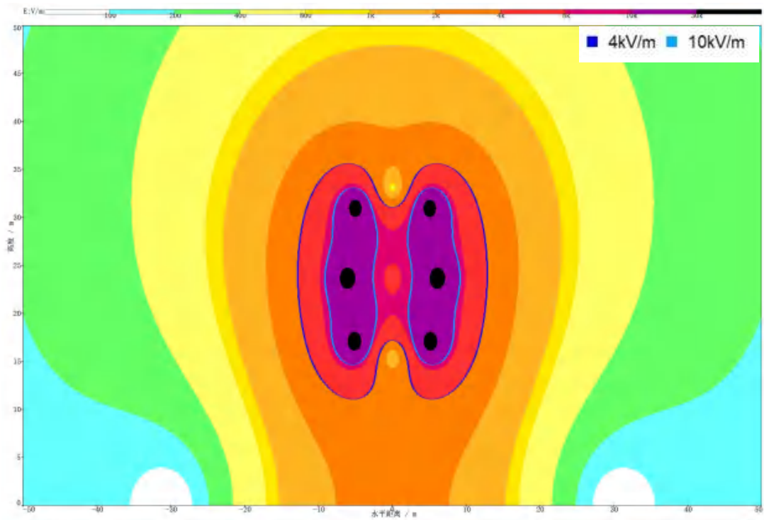
图 6.1-23 220kV 同塔双回线路（桐子湾~科学城段）导线对地 17m 工频电场强度空间分布图
