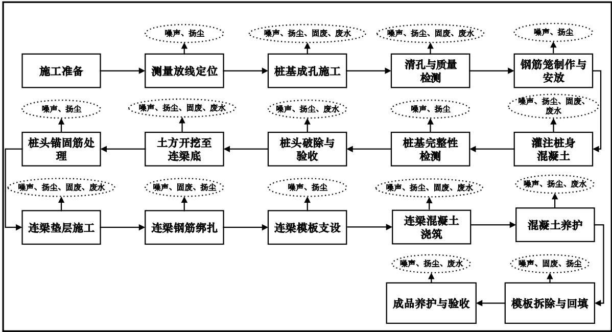
图 3.1-6 连梁桩基础施工流程图
