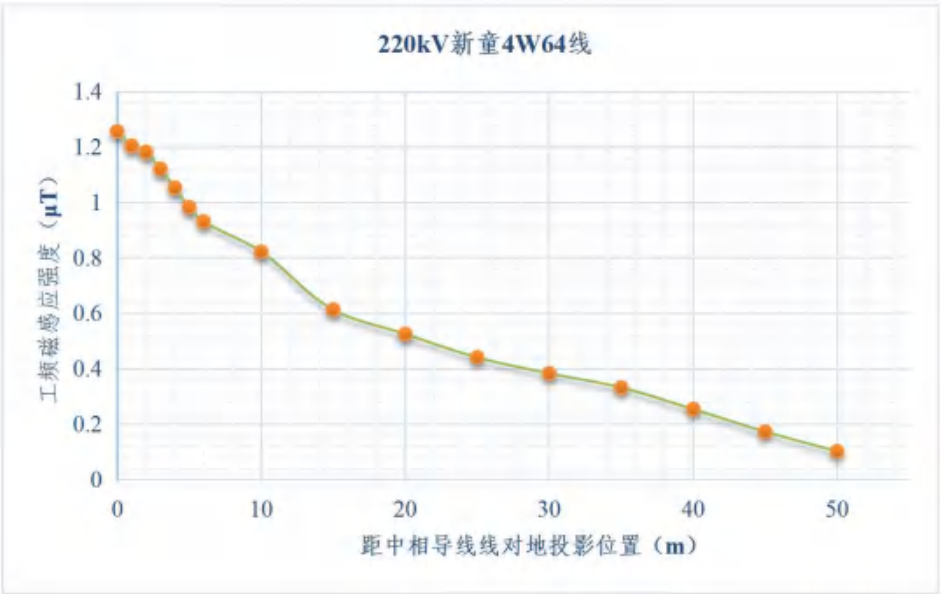
图 6.1-9 220kV 新童 4W64 线工频磁感应强度随距离的变化趋势
