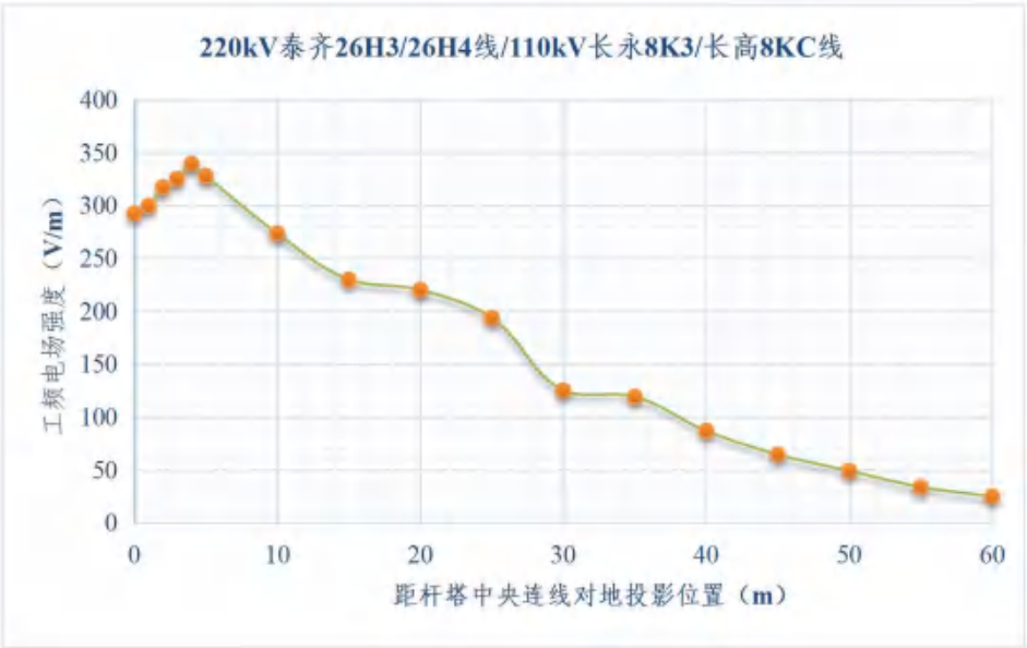
图 6.1-6 220kV 泰齐 26H3/26H4 线/110kV 长永 8K3/长高 8KC 线工频电场强度随距离的变化趋势
