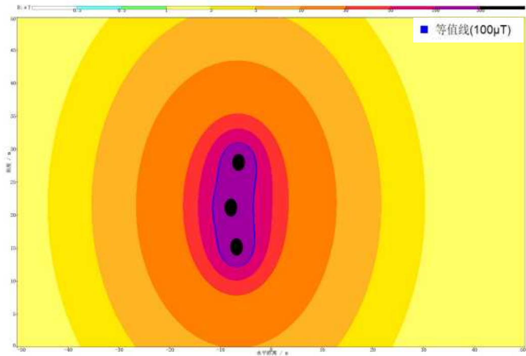
图 6.1-16 220-GB21S-JC4 塔型导线对地 15m 工频磁感应强度空间分布图
