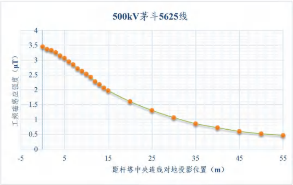
图 6.1-3 500kV 茅斗 5265 线工频磁感应强度随距离的变化趋势
