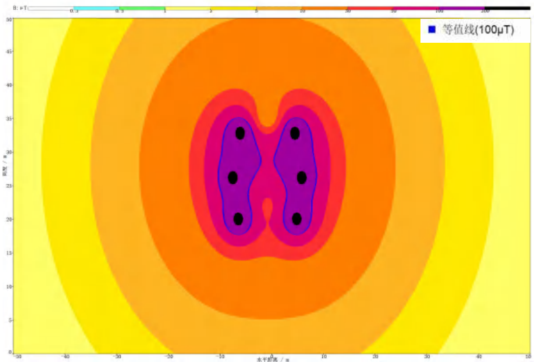
图 6.1-28 220kV 同塔双回（220kV 屏桐东西线迁改段）导线对地高度 20m 工频磁感应强度空间分布图
