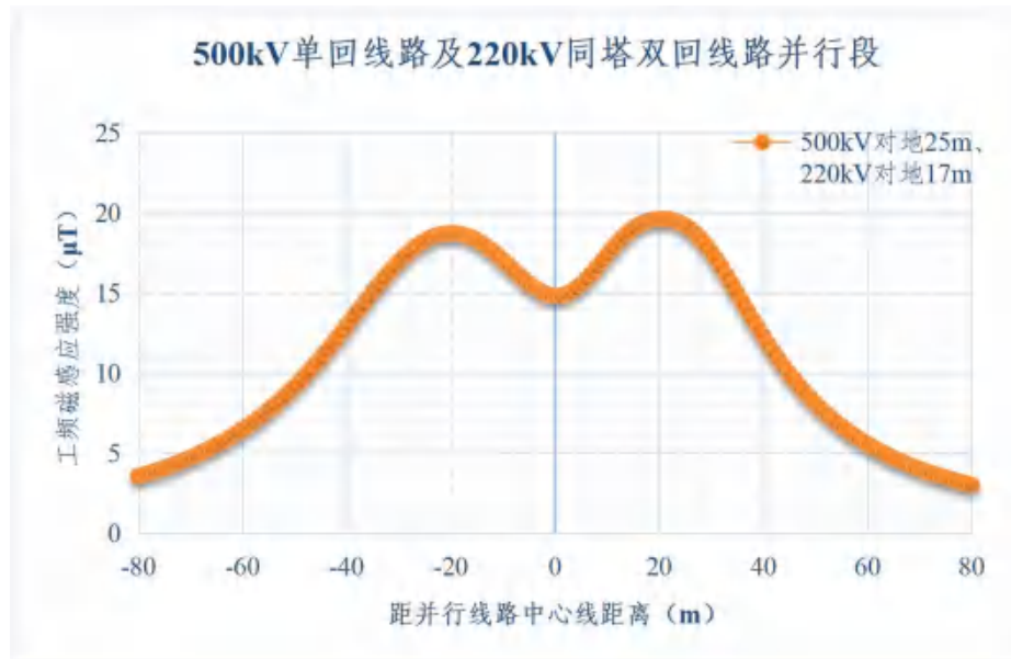
图6.1-38 500kV 单回架空线路与220kV 同塔双回架空线路并行段地面1.5m 产生 工频磁感应强度变化趋势
