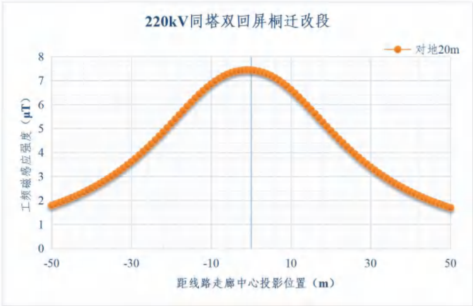
图6.1-26 220kV 同塔双回（220kV 屏桐东西线迁改段）导线对地高度20m 时 地面1.5m 工频磁感应强度变化趋势
