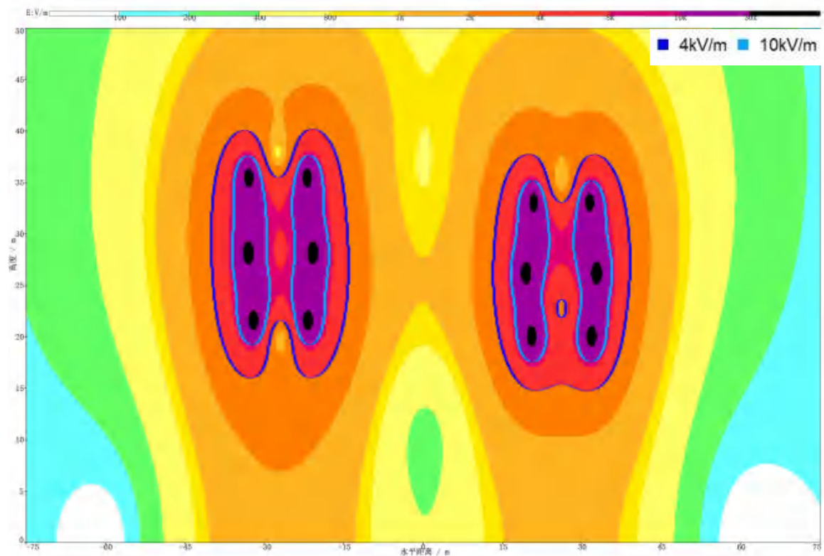
图 6.1-47 220kV 双回（桐子湾~科学城段）与 220kV 双回（屏桐东西线迁改）并行段工频电场强度空间分布图
