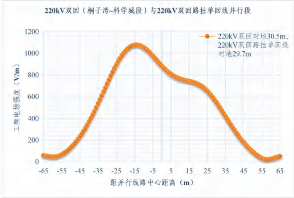
图 6.1-41 220kV 双回（桐子湾~科学城段）与 220kV 双回路挂单回线并行段地面 1.5m 处工频电场强度变化趋势
