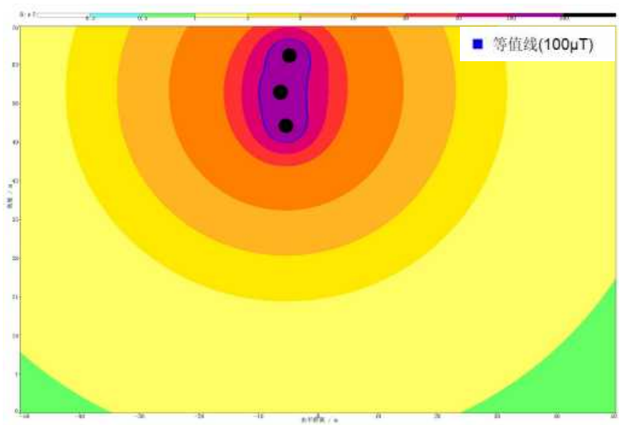
图 6.1-20 220kV 四回路挂单回线路导线对地 51.8m 时工频磁感应强度空间分布图
