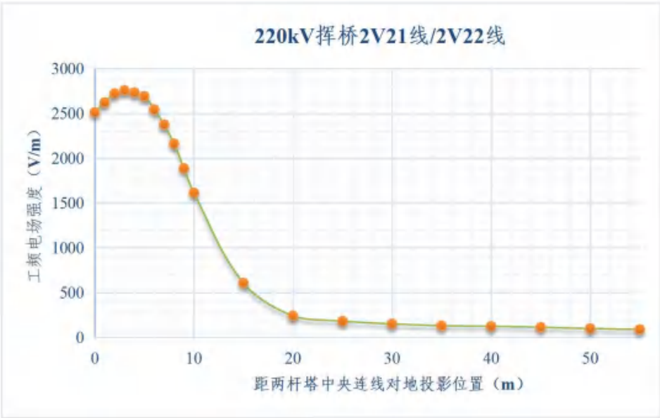
图 6.1-4 220kV 挥桥 2V21 线/2V22 线双回线路工频电场强度随距离的变化趋势
