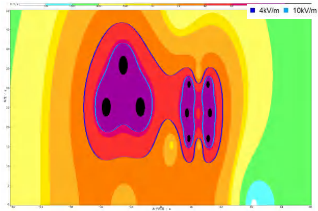
图 6.1-39 500kV 单回架空线路与 220kV 同塔双回架空线路并行段工频电场强度空间分布图
