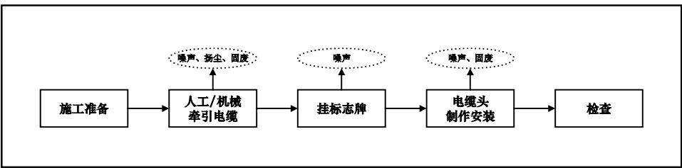
图3.1-10 电缆敷设施工流程图
