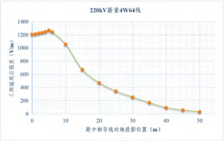
图 6.1-8 新童 4W64 线工频电场强度随距离的变化趋势
