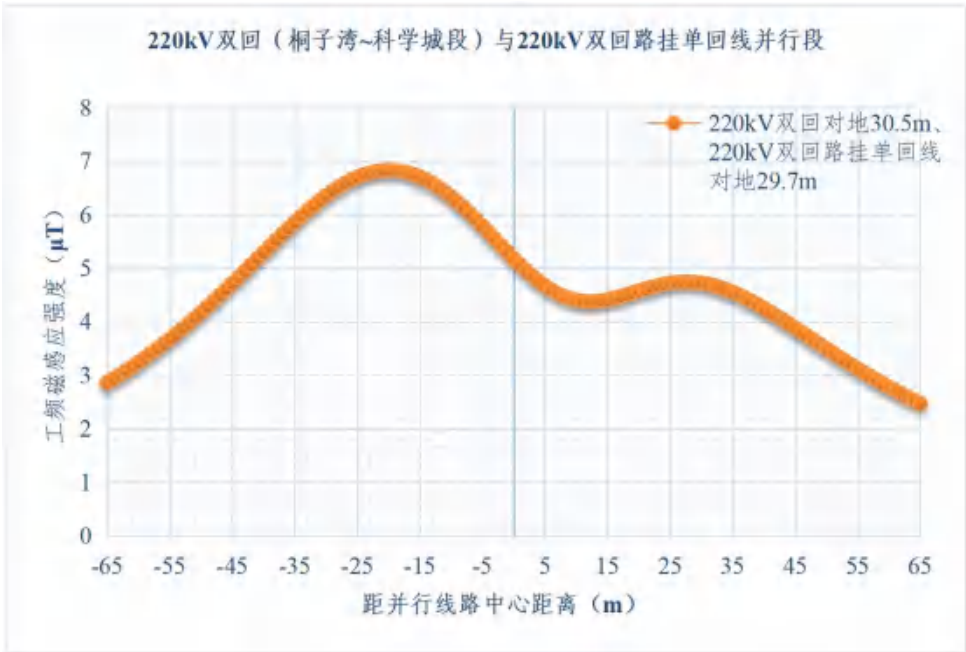
图6.1-42 220kV 双回（桐子湾~科学城段）与220kV 双回路挂单回线并行段地面1.5m 处产生工频磁感应强度变化趋势
