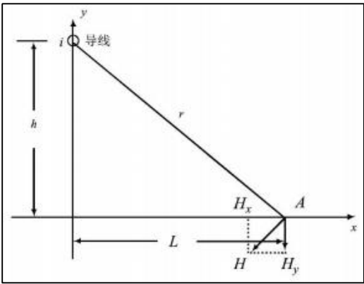
图 6.1-12 磁场向量图
