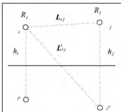
图 6.1-11 电位系数计算图
