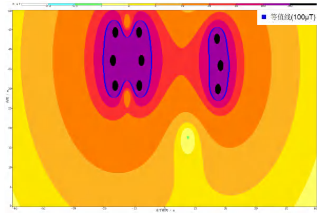
图 6.1-44 220kV 双回（桐子湾~科学城段）与 220kV 双回路挂单回线并行段工频磁感应强度空间分布图
