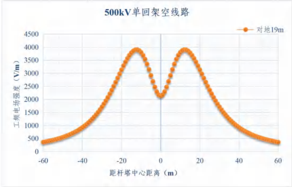
图 6.1-33 500kV 单回架空线路导线对地高度 19m 时地面 1.5m 处工频电场强度变化趋势
