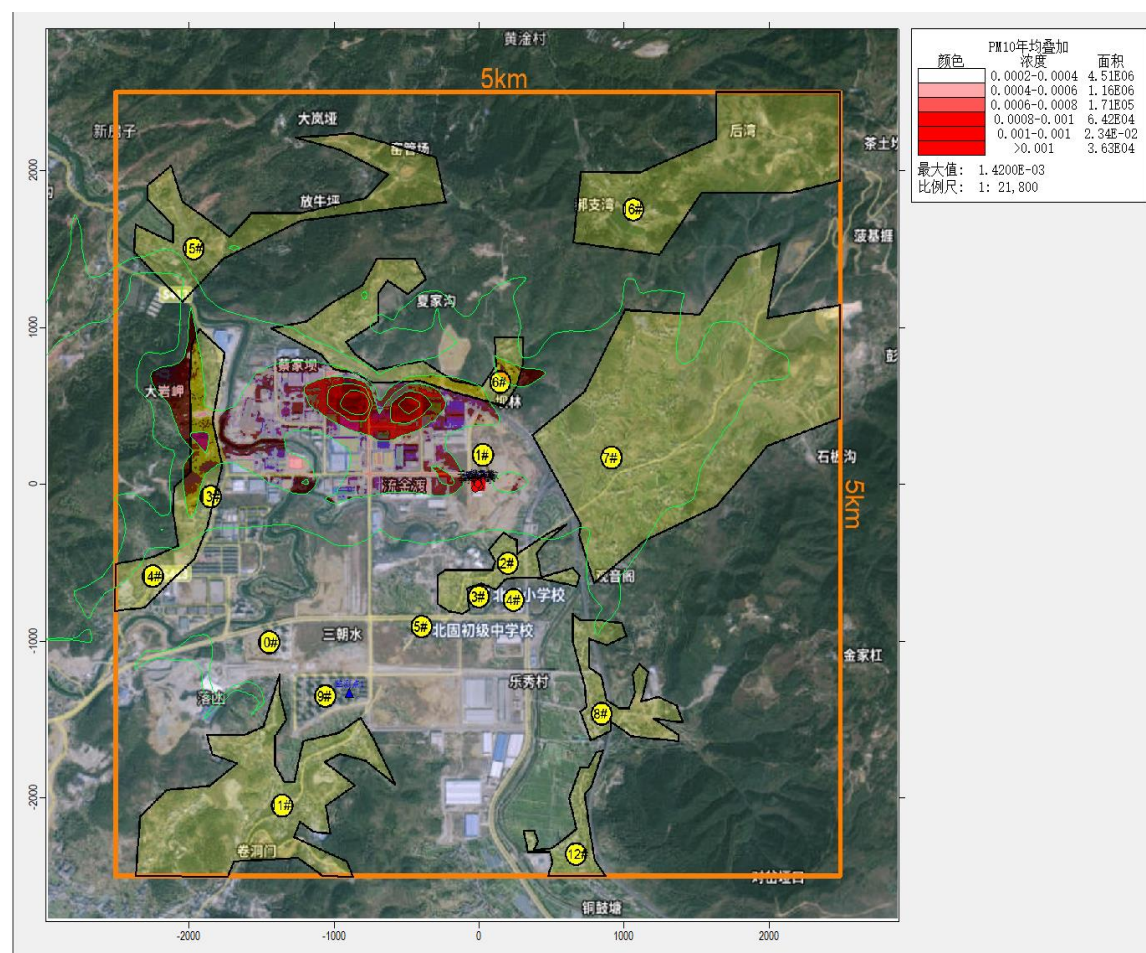
图 6.1-3-3 PM 10 叠加年均浓度影响分布图
