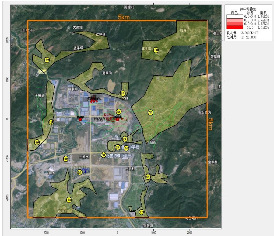
图 6.1-3-13 镉叠加年均浓度影响分布图
