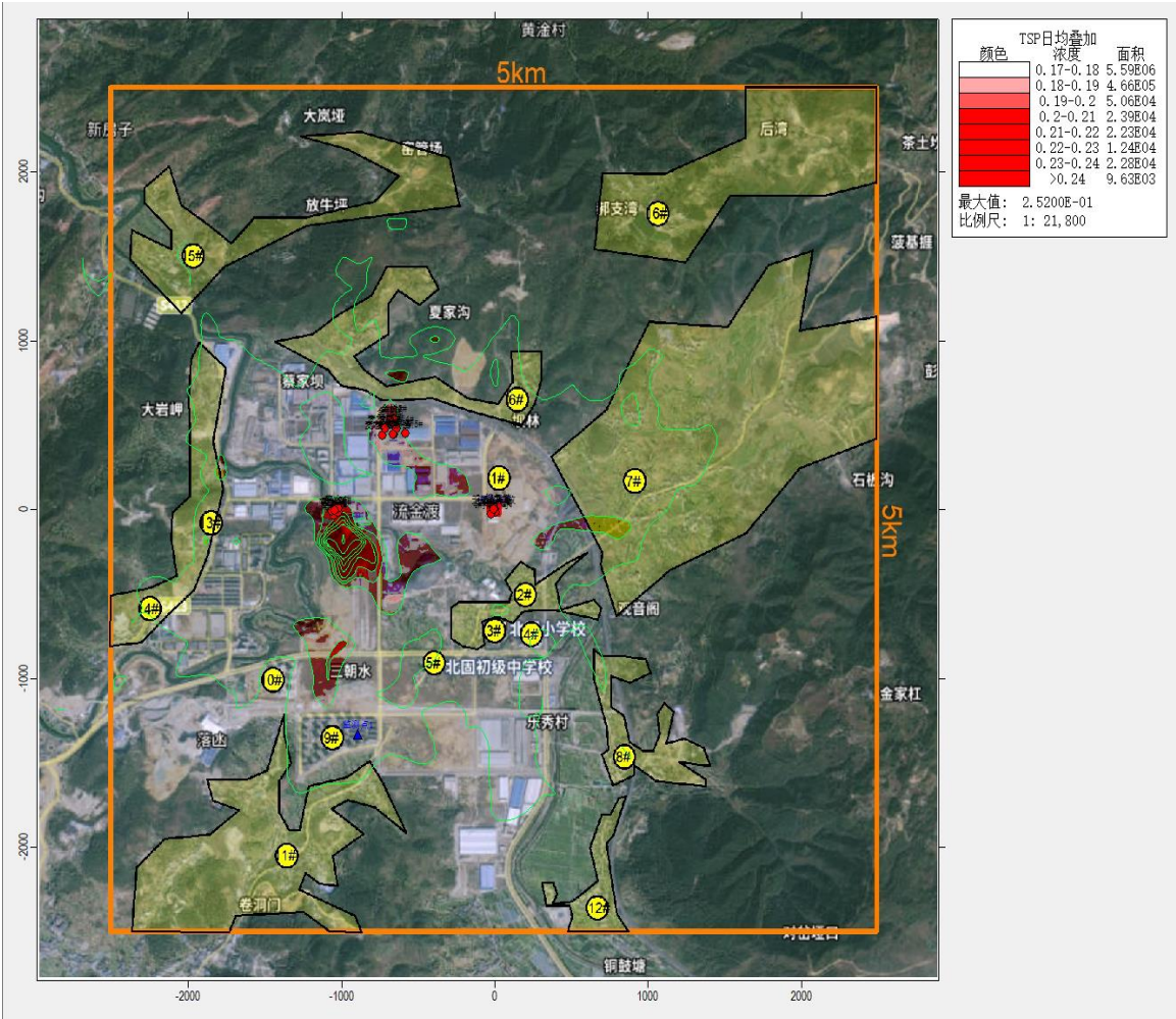
图 6.1-3-8 TSP 叠加日均浓度影响分布图
