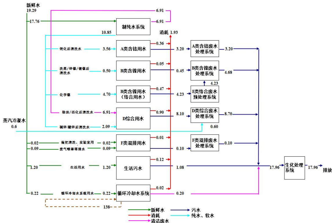
图 3.5-4 总水平衡图 单位: \text{m}^3/\text{d}
