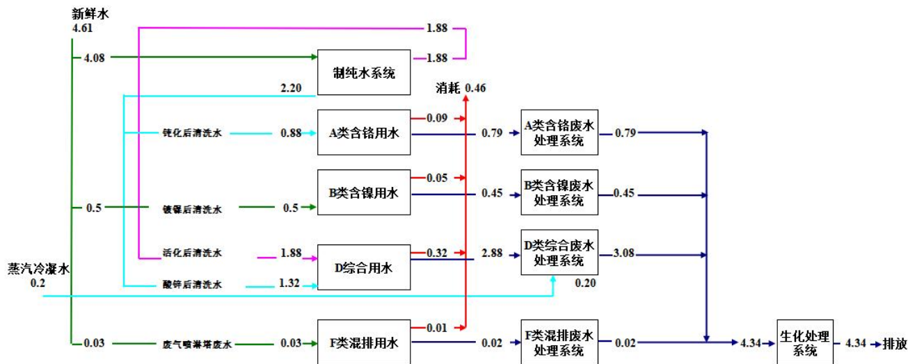
图 3.5-3 3#酸锌、锌镍生产线水平衡图 单位: \text{m}^3/\text{d}
