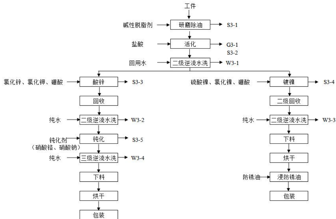
图 3.3-3 镀酸锌、镀镍生产线工艺流程及产污环节图
