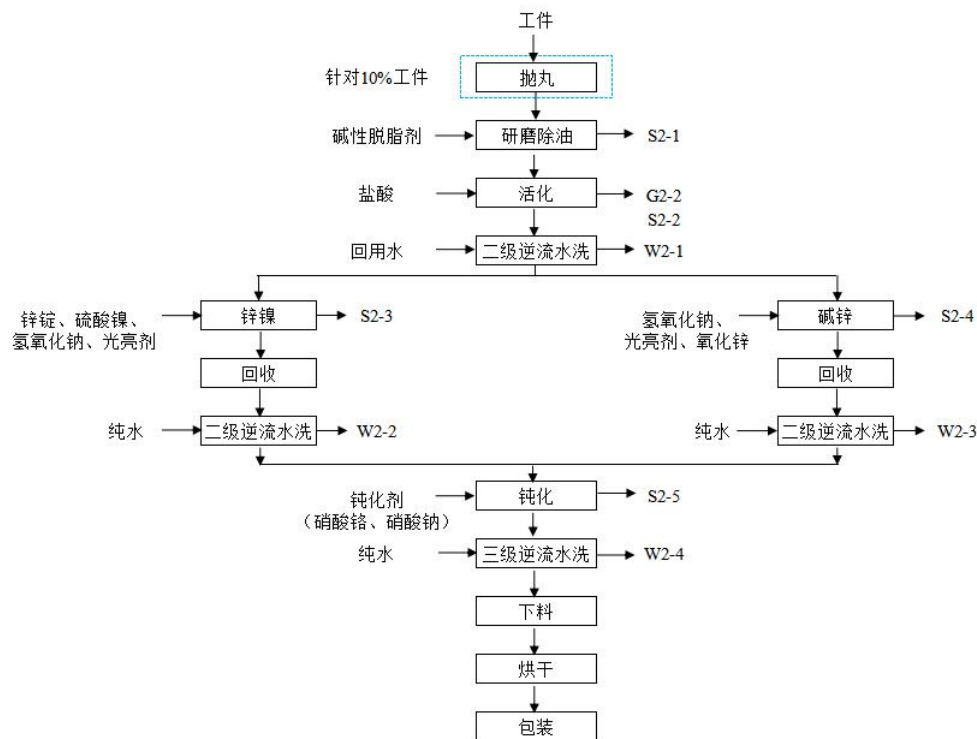
图 3.3-2 镀碱锌、锌镍生产线工艺流程及产污环节图
