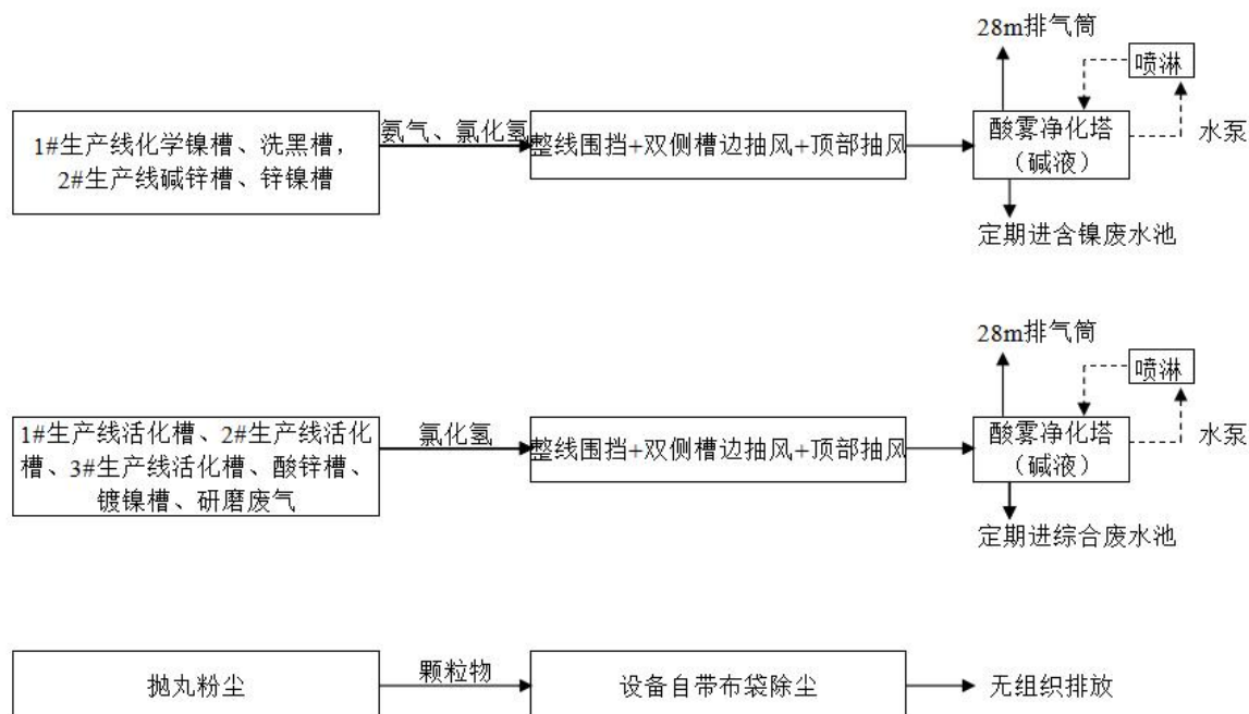
图 7.1-1 废气处理措施示意图
