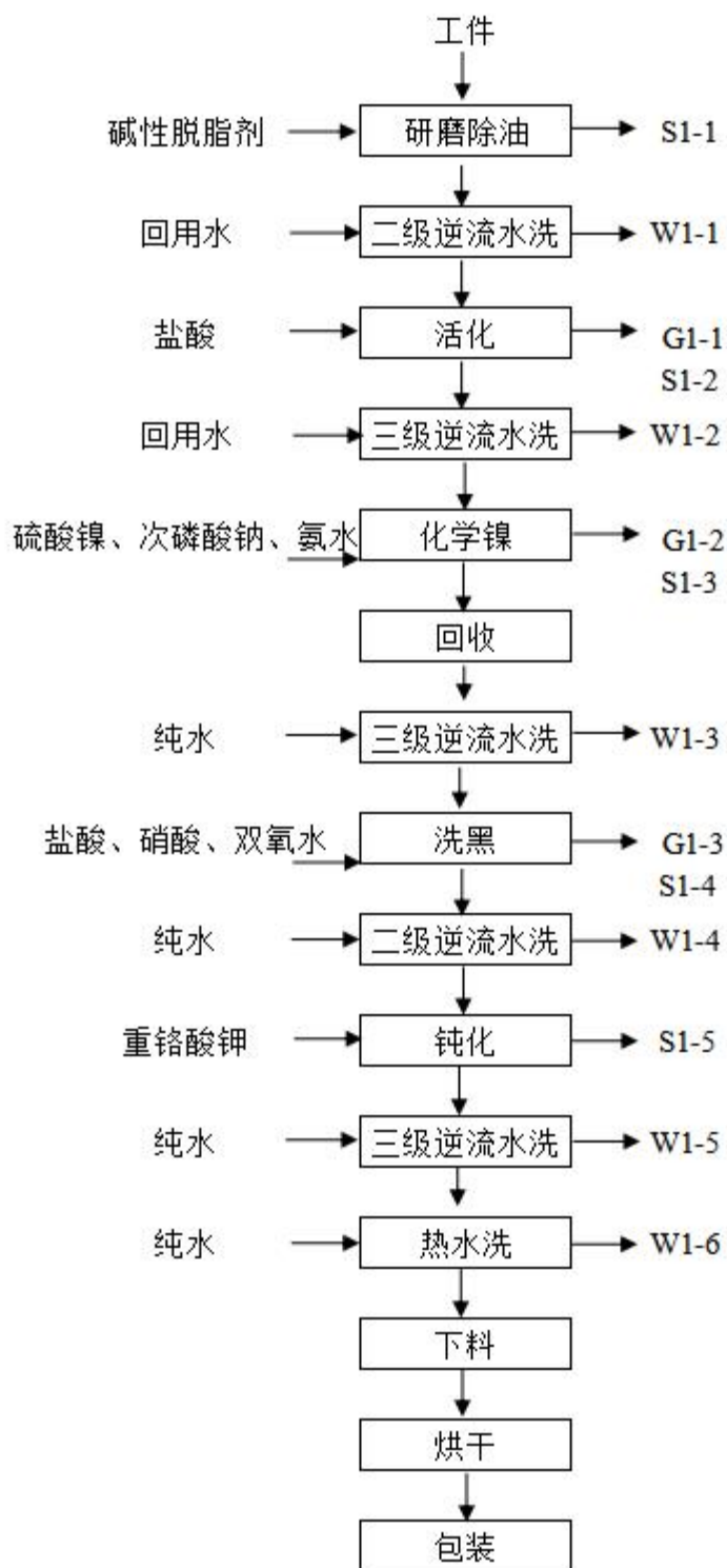
图 3.3-1 化学镍生产线工艺流程及产污环节图
