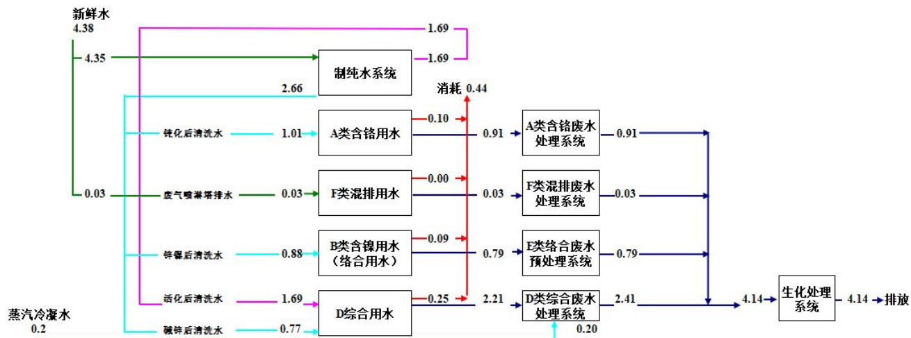
图 3.5-2 2#碱锌、锌镍生产线水平衡图 单位: \text{m}^3/\text{d}
