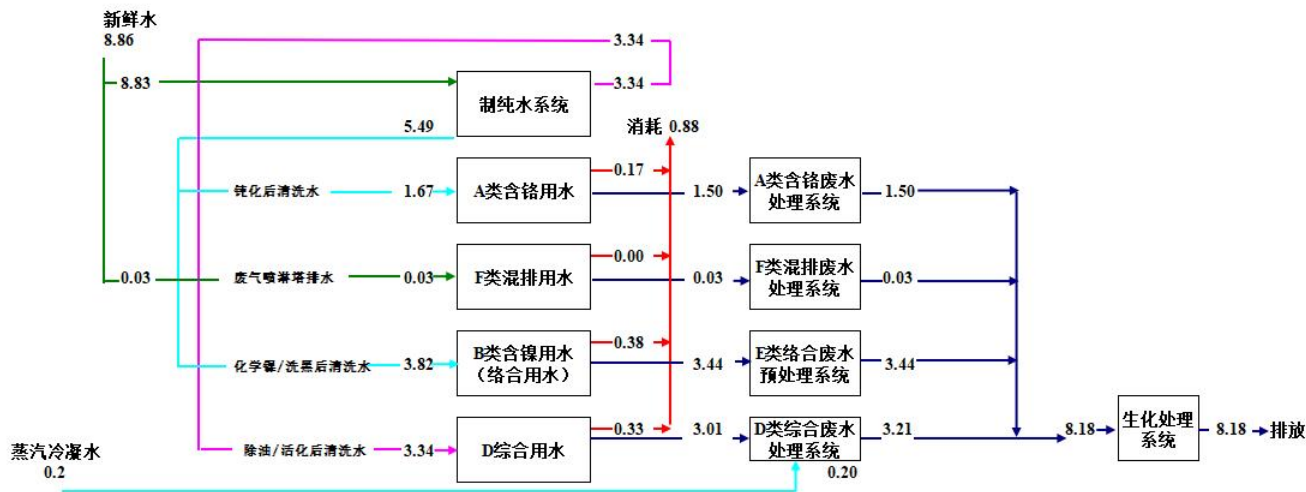
图 3.5-1 1#化学镍生产线水平衡图 单位：m³/d
