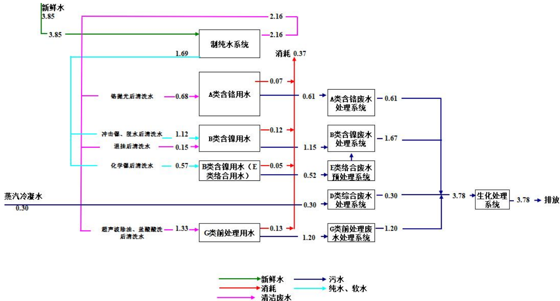
图 3.5-2 铁件化学镍线、退挂线水平衡图 单位: m³/d
