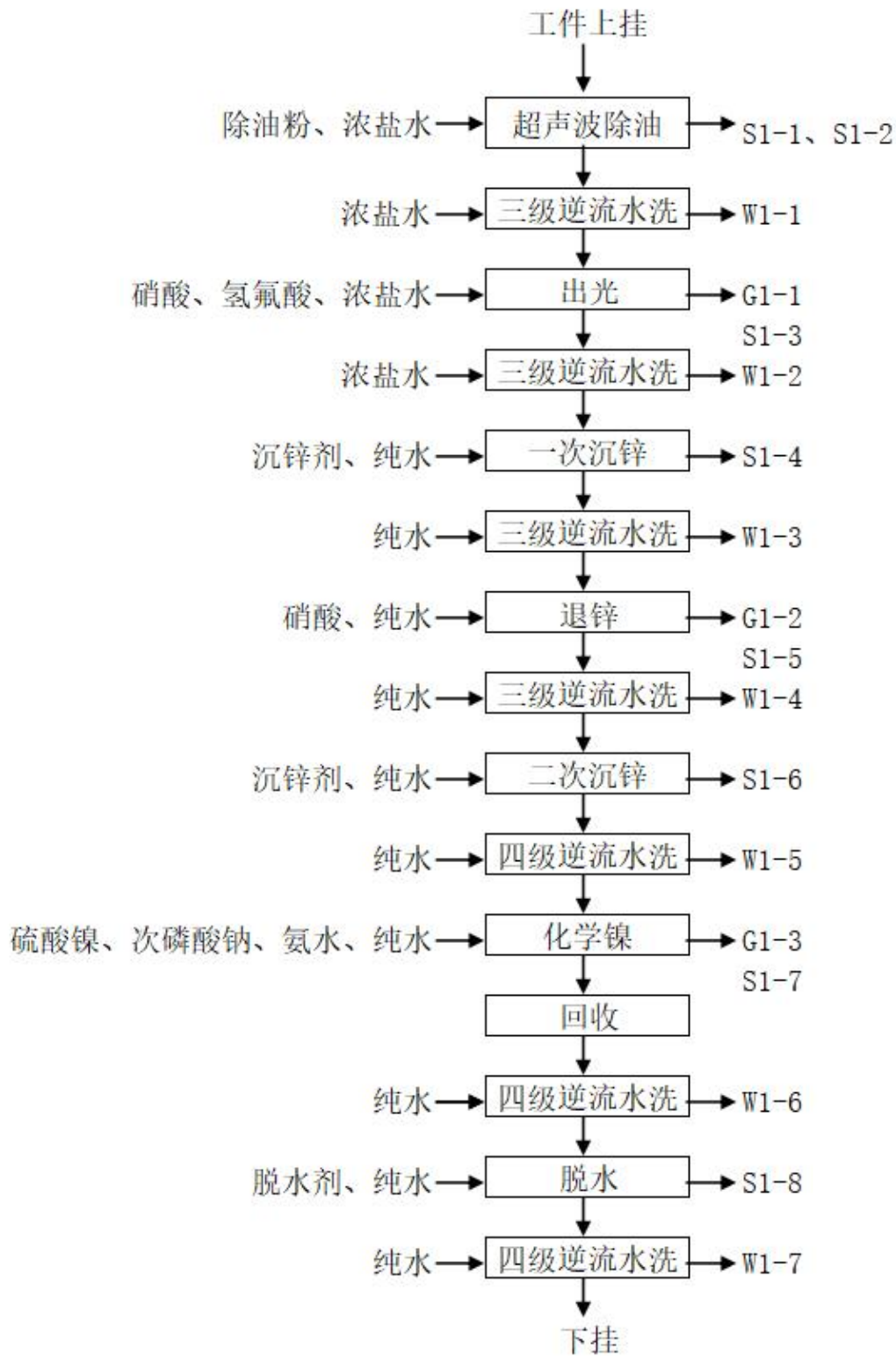
图 3.3-1 铝件化学镍生产线工艺流程及产污环节图
