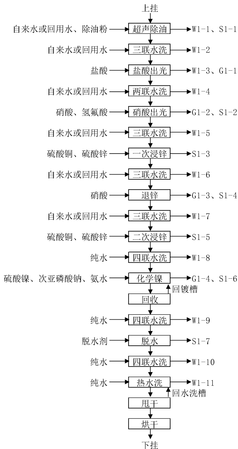
图 2.3-1 挂镀化学镍生产线工艺流程及产排污环节分析图
