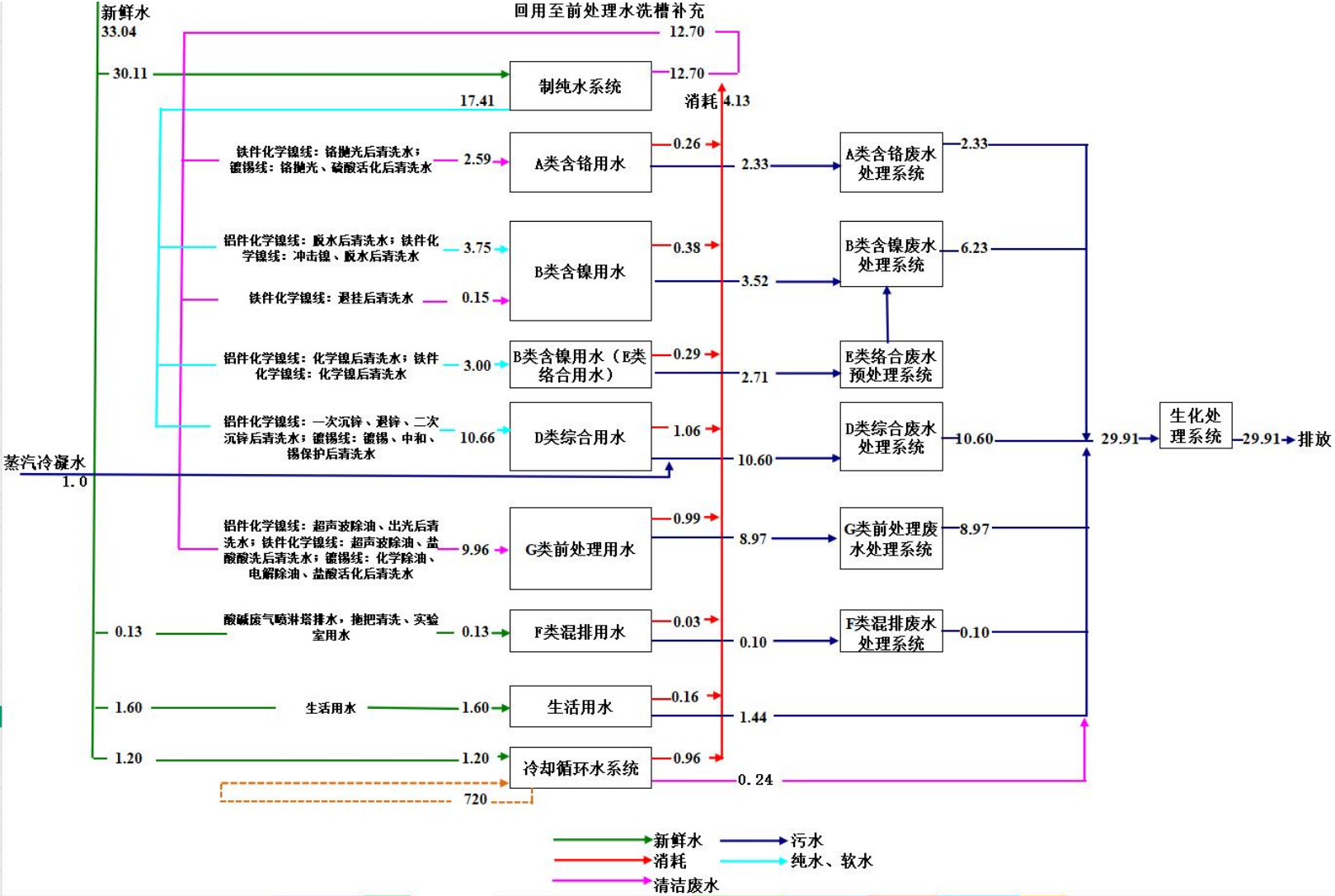
图 3.5-4 项目总水平衡图 单位: m³/d
