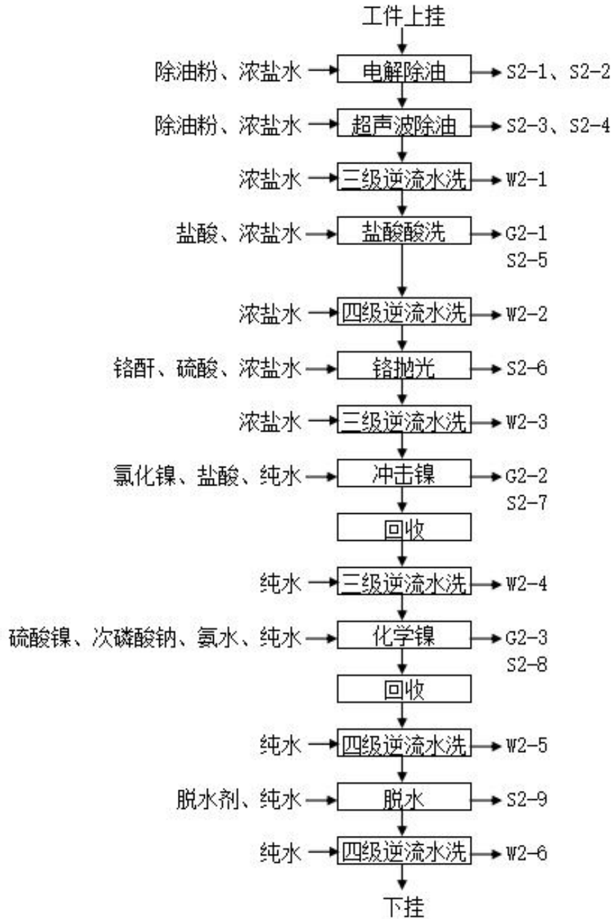
图 3.3-2 铁件化学镍生产线工艺流程及产污环节图
