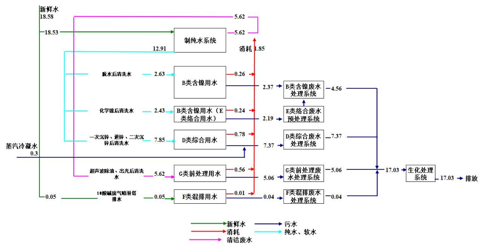
图 3.5-1 铝件化学镍线水平衡图 单位: m³/d
