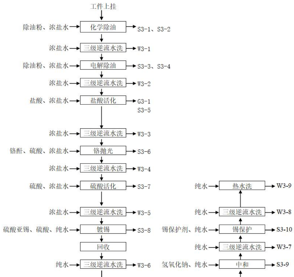
图 3.3-3 镀锡生产线工艺流程及产污环节图
