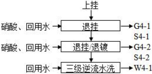
图 3.3-4 退挂退镀线工艺流程及产污环节图
