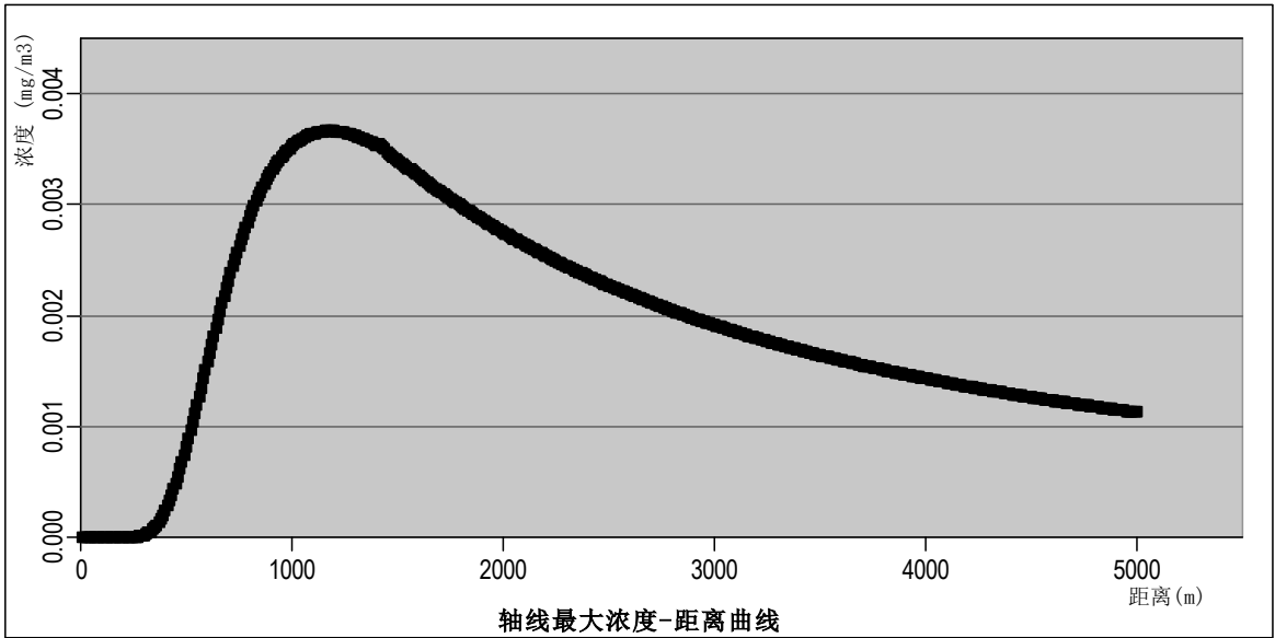
图 6.5-2 氨气轴线最大浓度分布图
