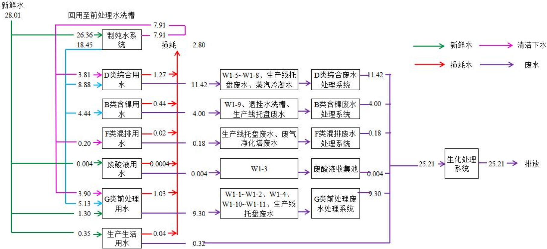
图 2.3-2 现有工程水平衡图 单位：m³/d
