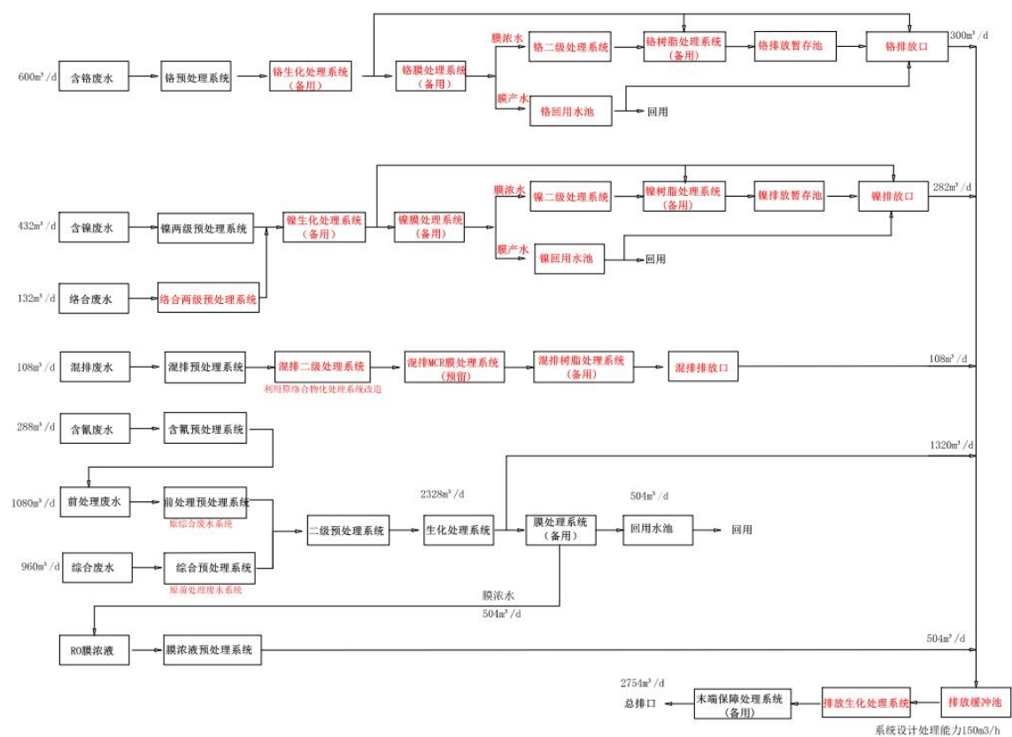
重润科技园废水处理中心工艺流程
