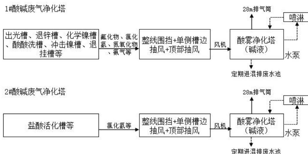
图 7.1-1 酸雾净化装置处理流程图
