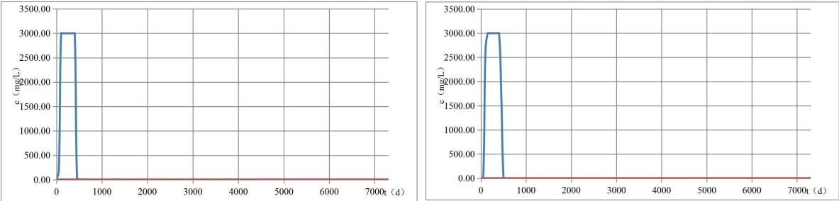
图 5.5.3-8 下游厂界处、高相沟处污染物氨氮浓度贡献值与时间变化关系图
