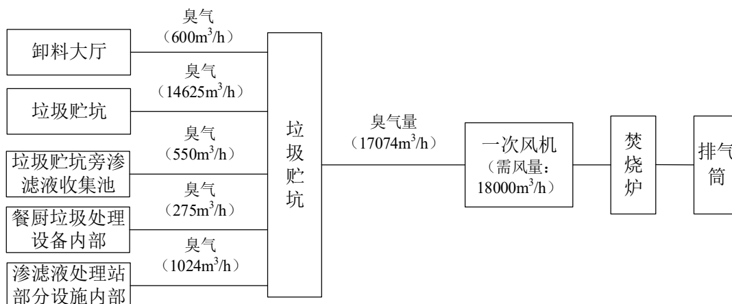
图 7.1-4 焚烧炉正常运行时高浓度臭气治理示意图
