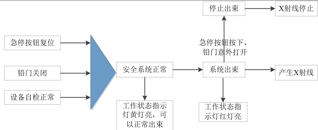
图 10-6 本项目辐射安全联锁逻辑图
