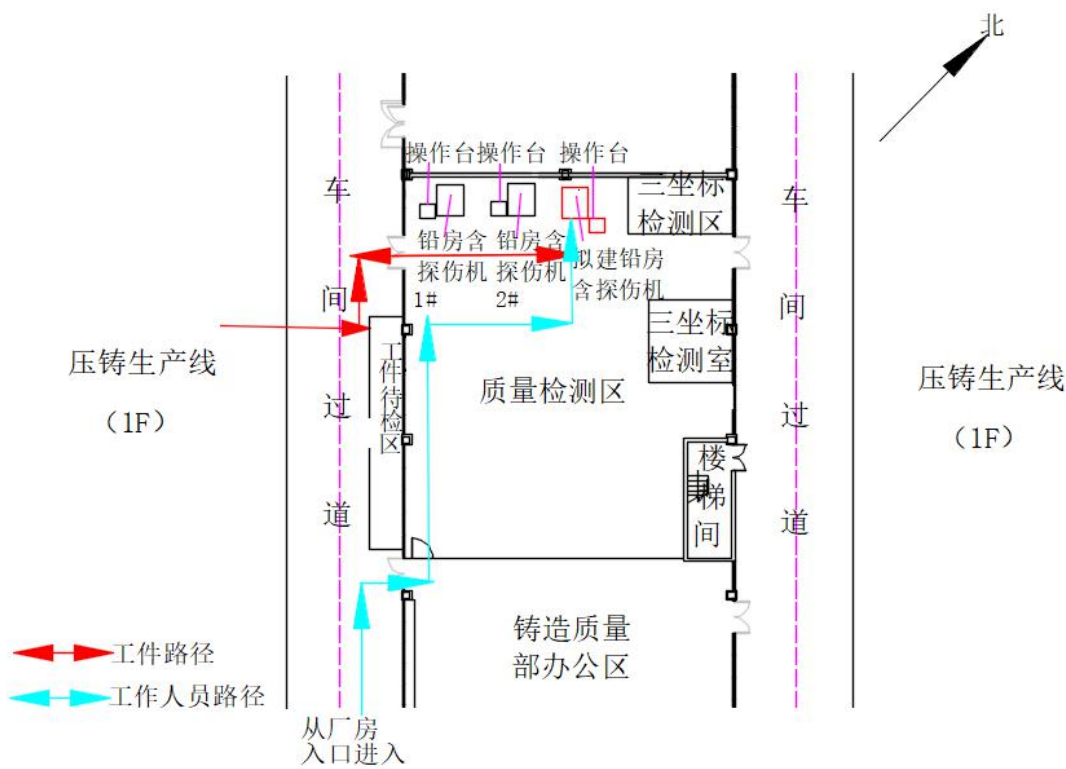
图 9-5 项目人流、物流路径规划示意图
