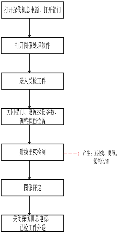
图 9-4 本项目 X 射线无损检测工艺流程及产排污简图
