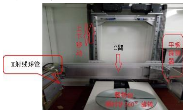
图9-2 运动轨迹示意图
