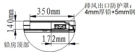
图 10-1 排风口防护罩示意图
