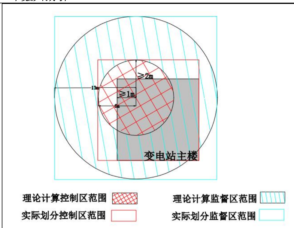
图 11-5 室内变电站现场探伤工作场所分区示意图 (照射方向竖直向下)
