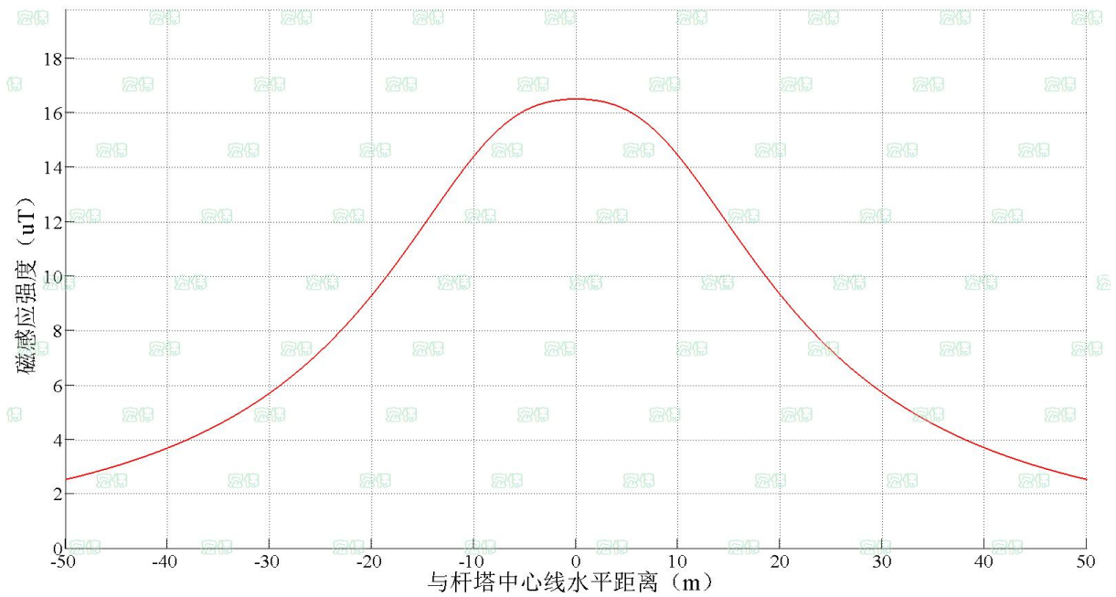
图 3-2 新建线路离地 1.5m 处工频磁感应强度分布曲线图 电场强度二维分布图 电场单位: kV/m
