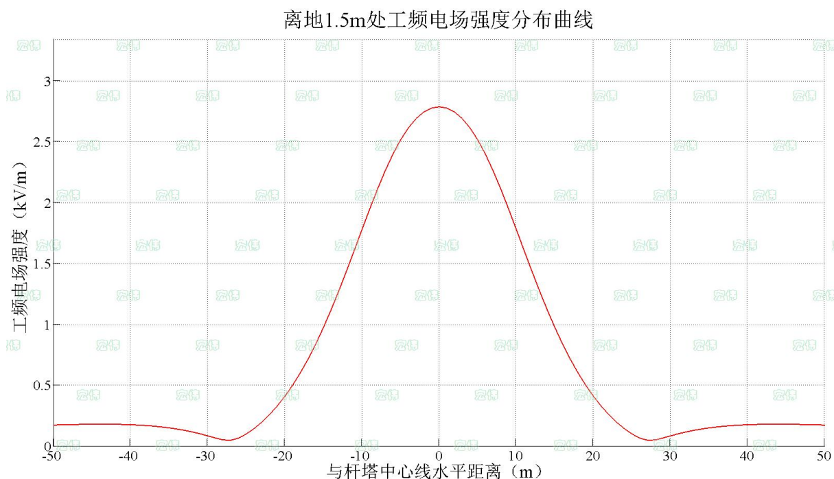
图 3-1 新建线路离地 1.5\text{m} 处工频电场强度分布曲线图
