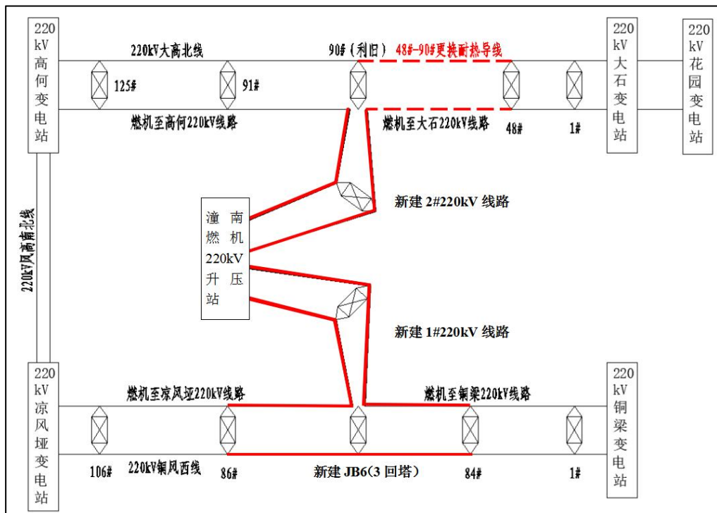
图 1-1 接入系统方案示意图
