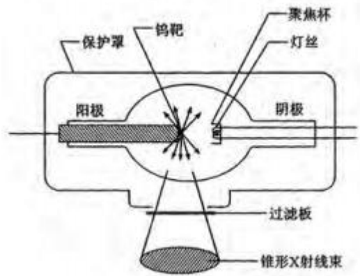
图 9-3 X 射线管示意图
