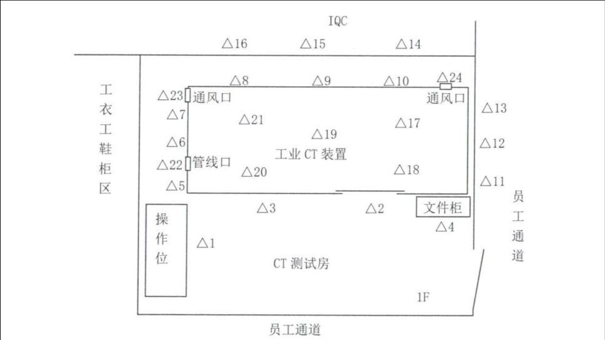
图 11-2 类比监测布点示意图
