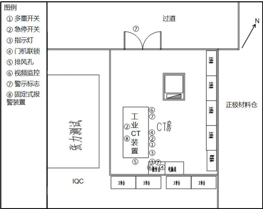
图 10-6 辐射安全与防护设施布置示意图
