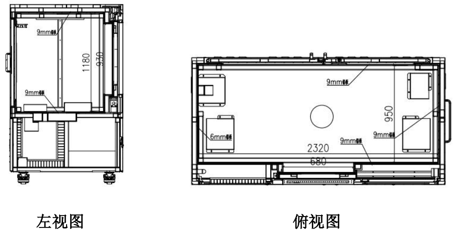
图 10-3 屏蔽体左视和俯视图
