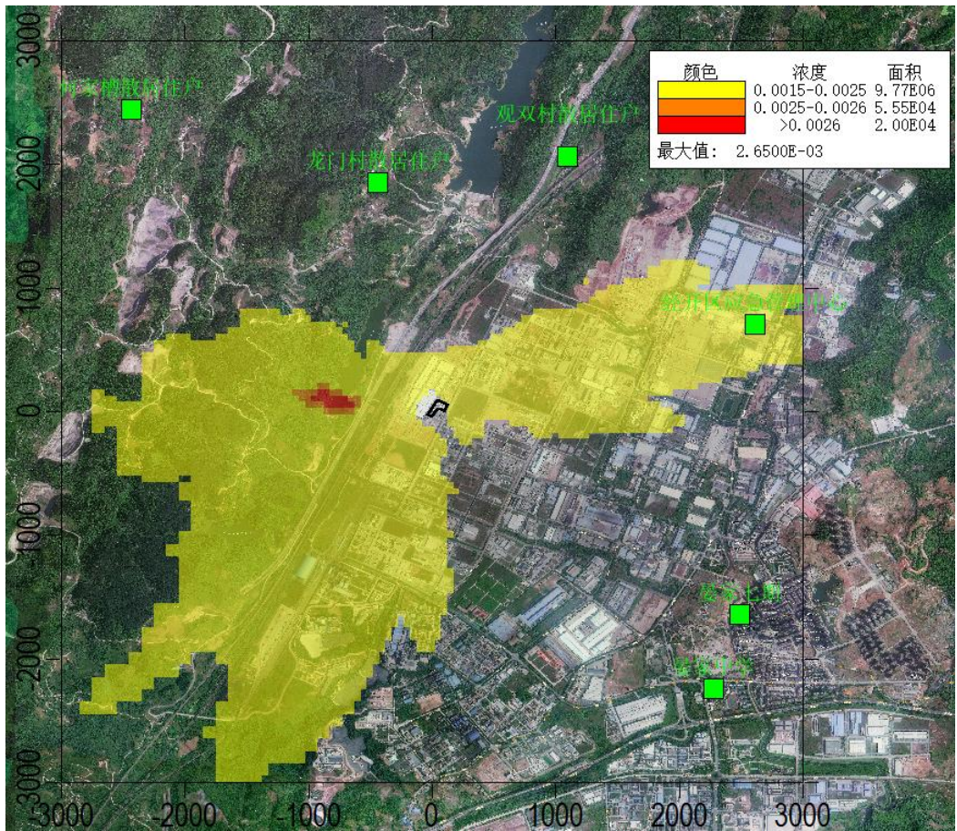
图5.1.8-8 镉日均浓度叠加值等值线图
