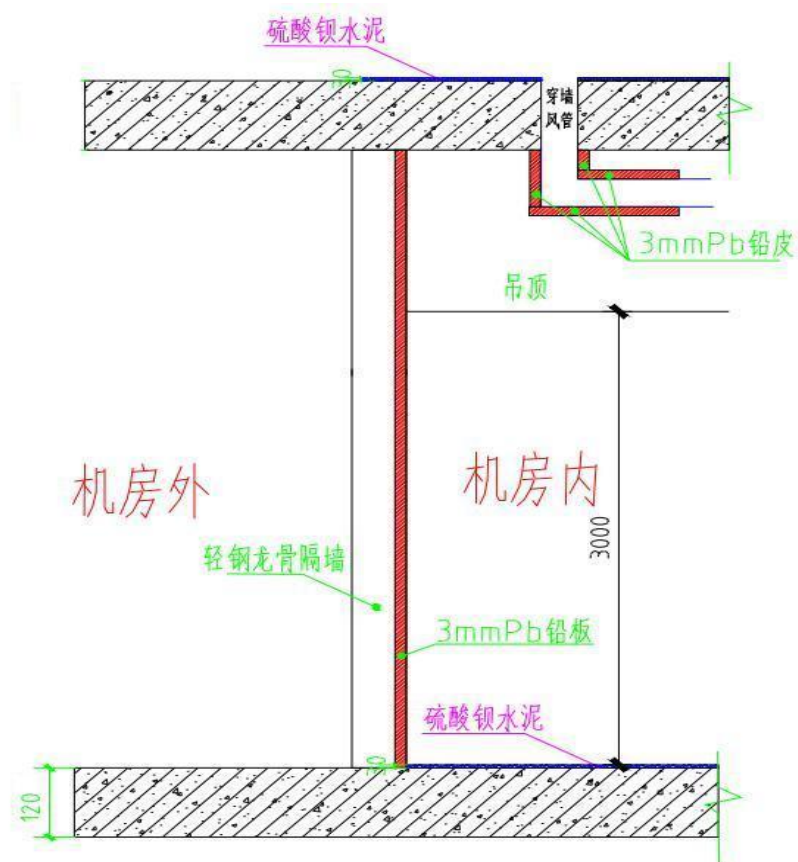
图10-3 排风井穿墙示意图
