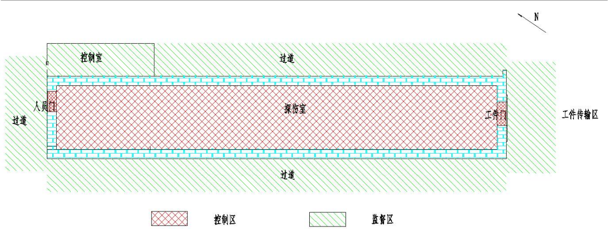
图 10-1 探伤室工作场所分区布置图
