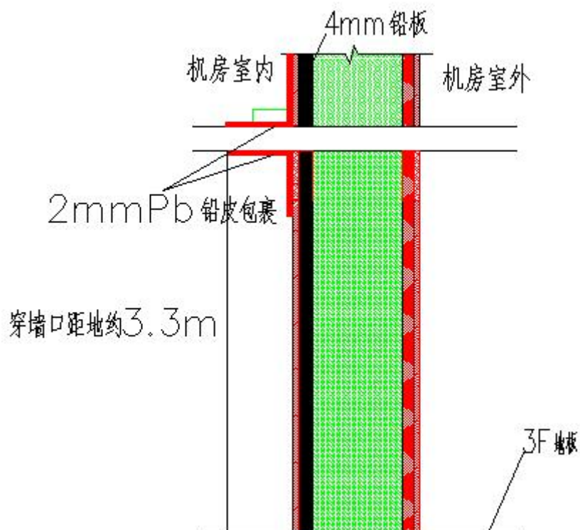
图10-3 风管穿越墙体示意图
