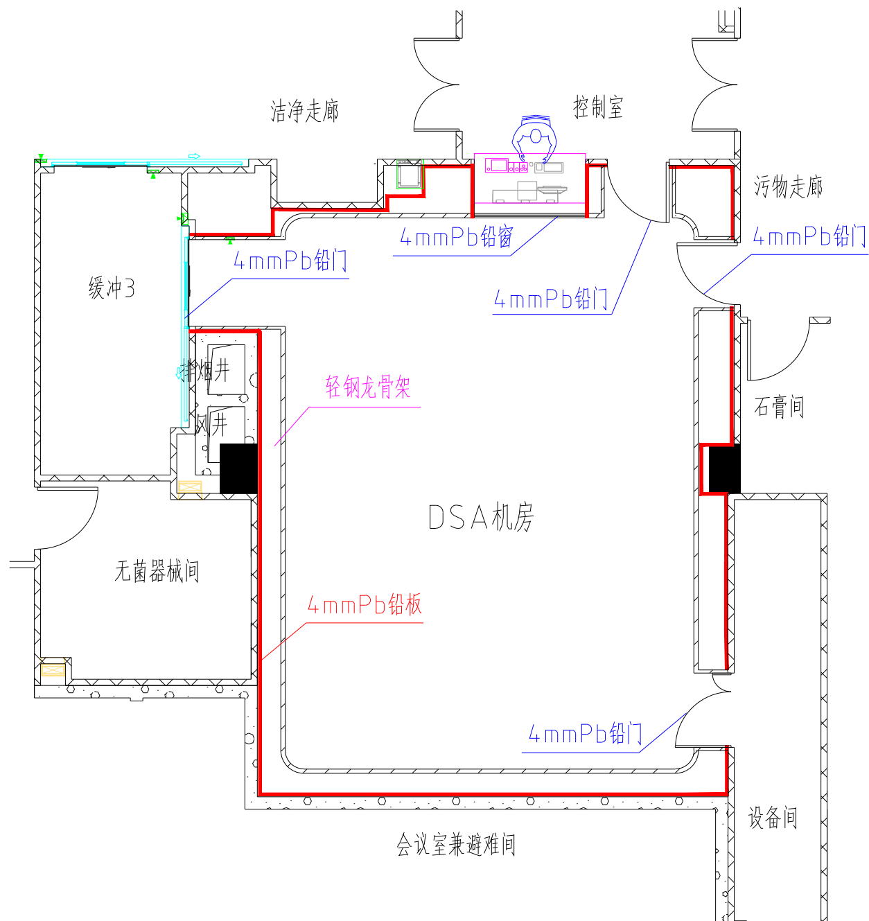
附图6-1 本项目DSA机房设计屏蔽防护平面图
