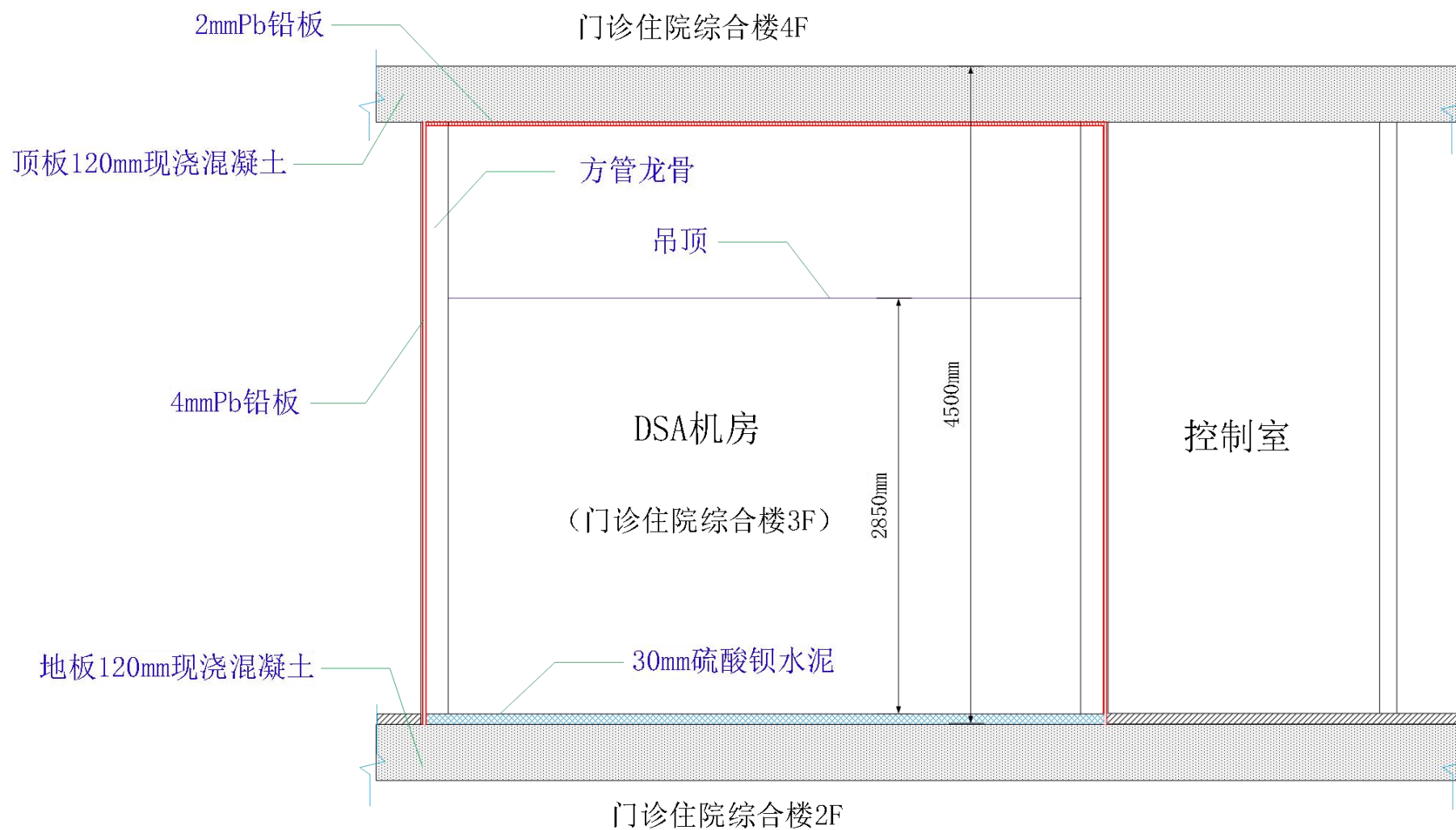
附图6-2 本项目DSA机房设计屏蔽防护立面图
