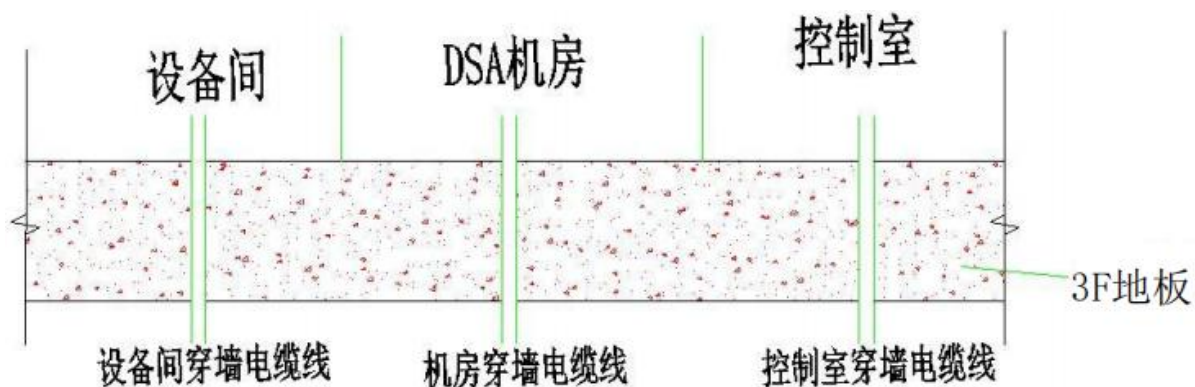
图10-4 电缆穿墙管线走向示意图
