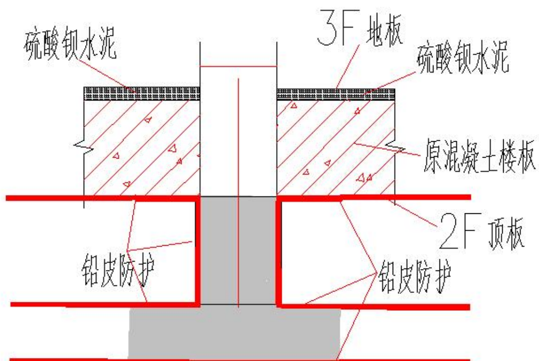
图10-5 电缆穿墙部分详图
