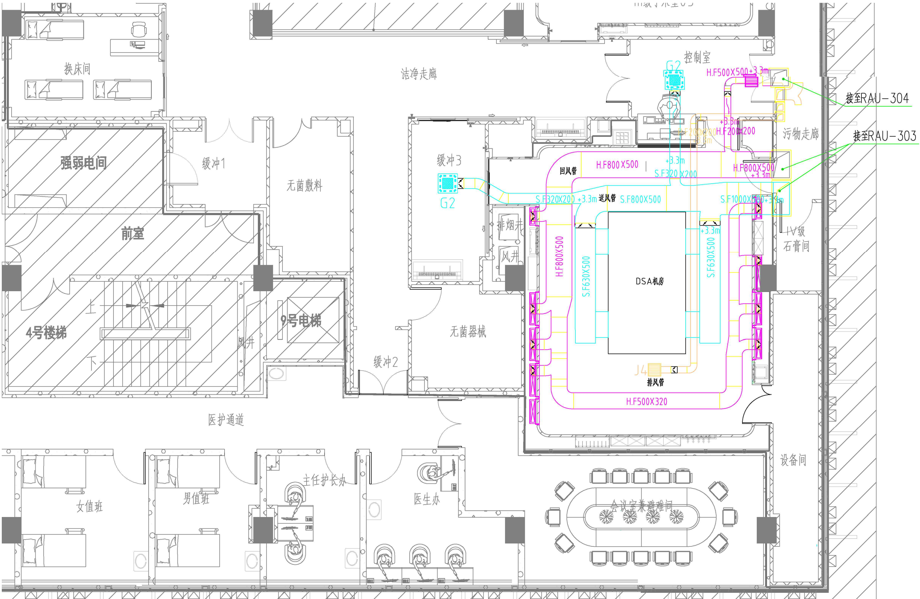
附图9 本项目拟建DSA机房通风图
