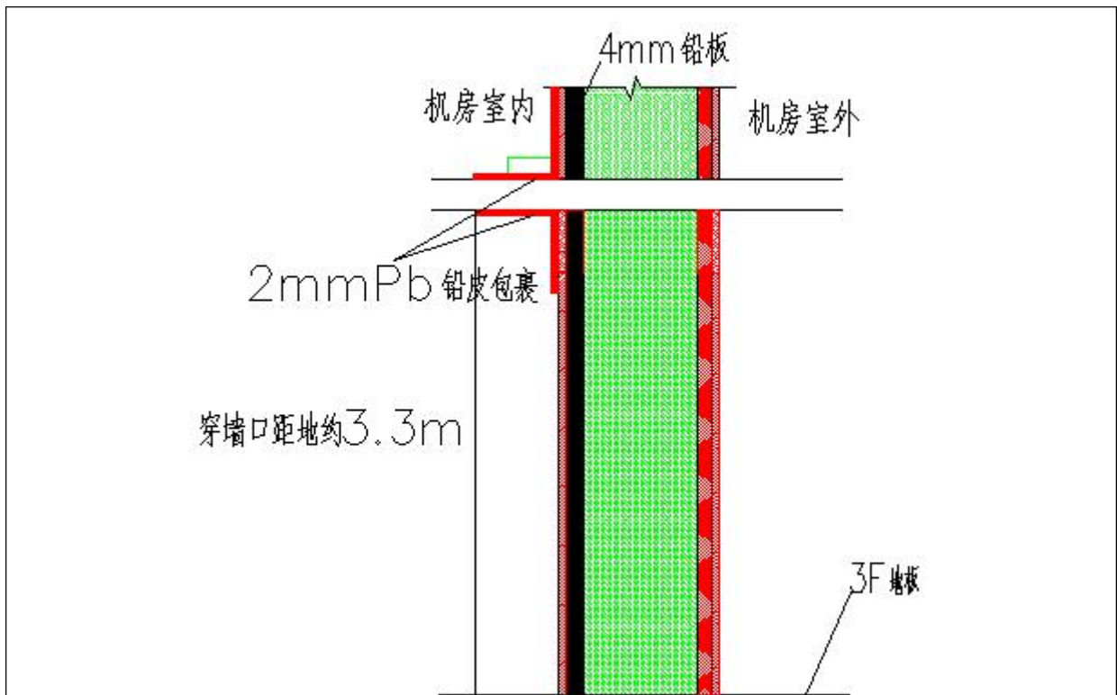
图10-3 风管穿越墙体示意图
