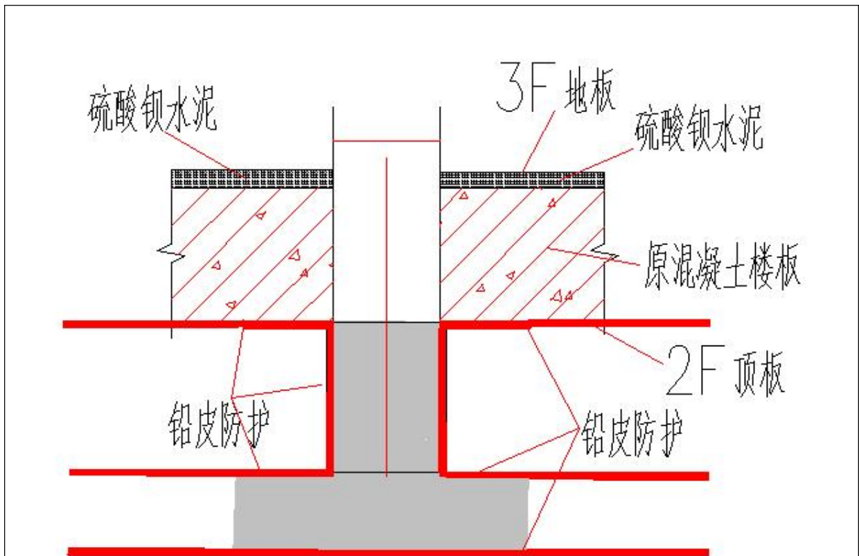
图10-5 电缆穿墙部分详图
