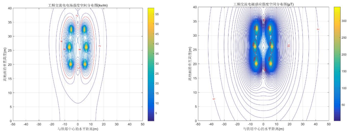
图 3-2 220kV 双回线路导线对地高度 20m 时工频电场强度空间分布图
