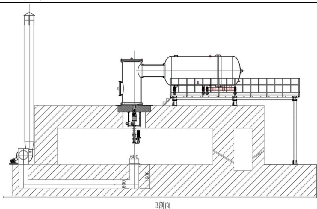
图 10-3 排风风道辐射防护屏蔽设计示意图
