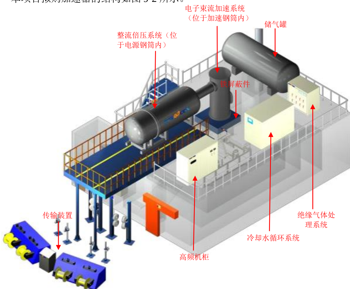
图9-2 L型半自屏蔽电子加速器结构示意图
