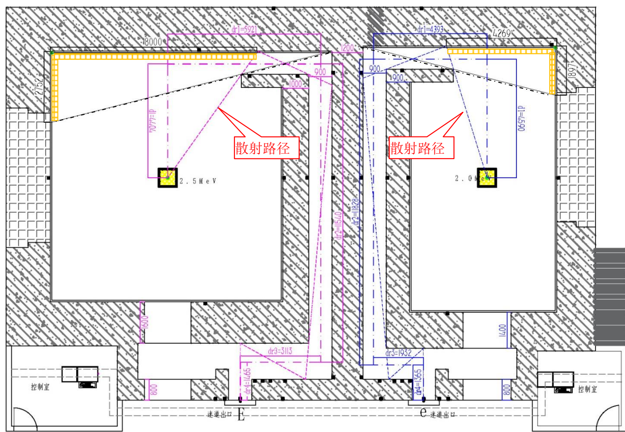
图11-3 辐照室反散射核算平面示意图
