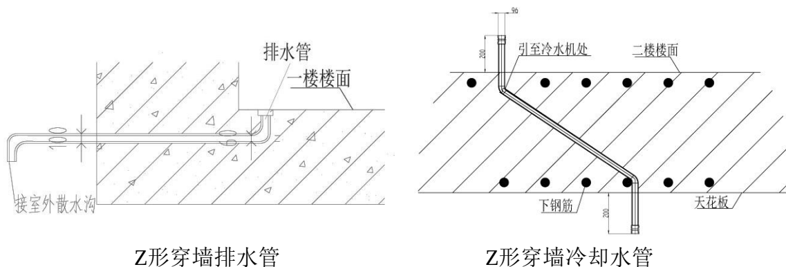
图10-2 穿墙管线辐射防护屏蔽设计示意图
