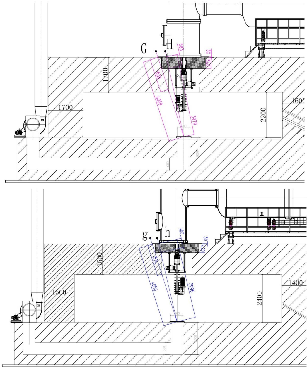
图11-2 辐照室X射线透射屏蔽效能立面核算示意图
