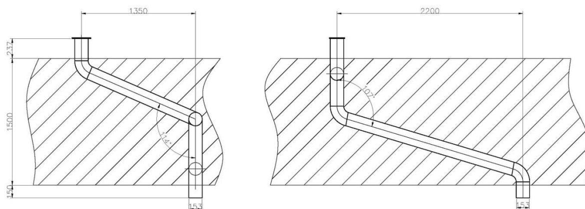
钛窗风管穿墙大样
