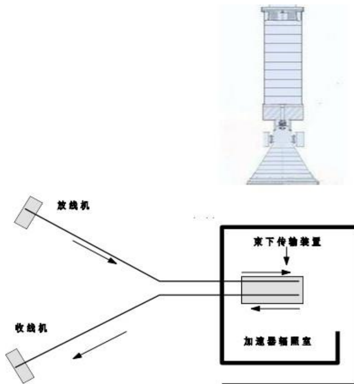
图 9-8 电缆辐照交联工艺示意图
