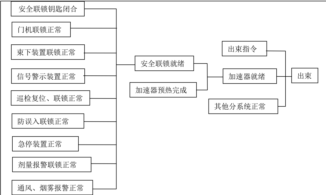
图10-9 安全联锁设施逻辑示意图
