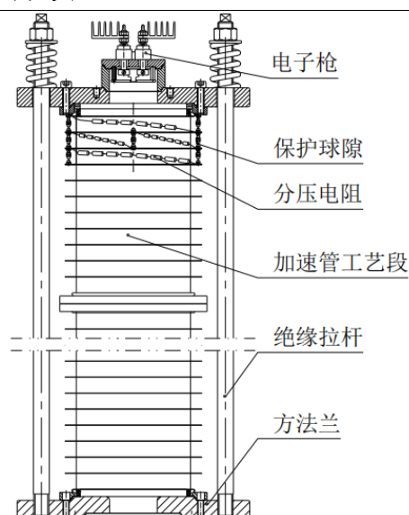
图9-4 束流加速系统示意图
