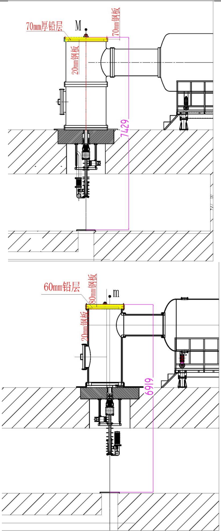
图11-4 顶棚设备区180° 反散射次级X射线计算点
