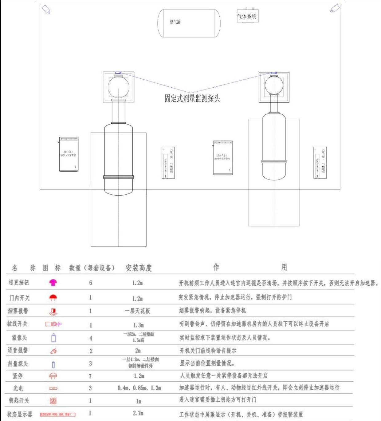
图10-8 辐射安全与防护设施布置示意图
