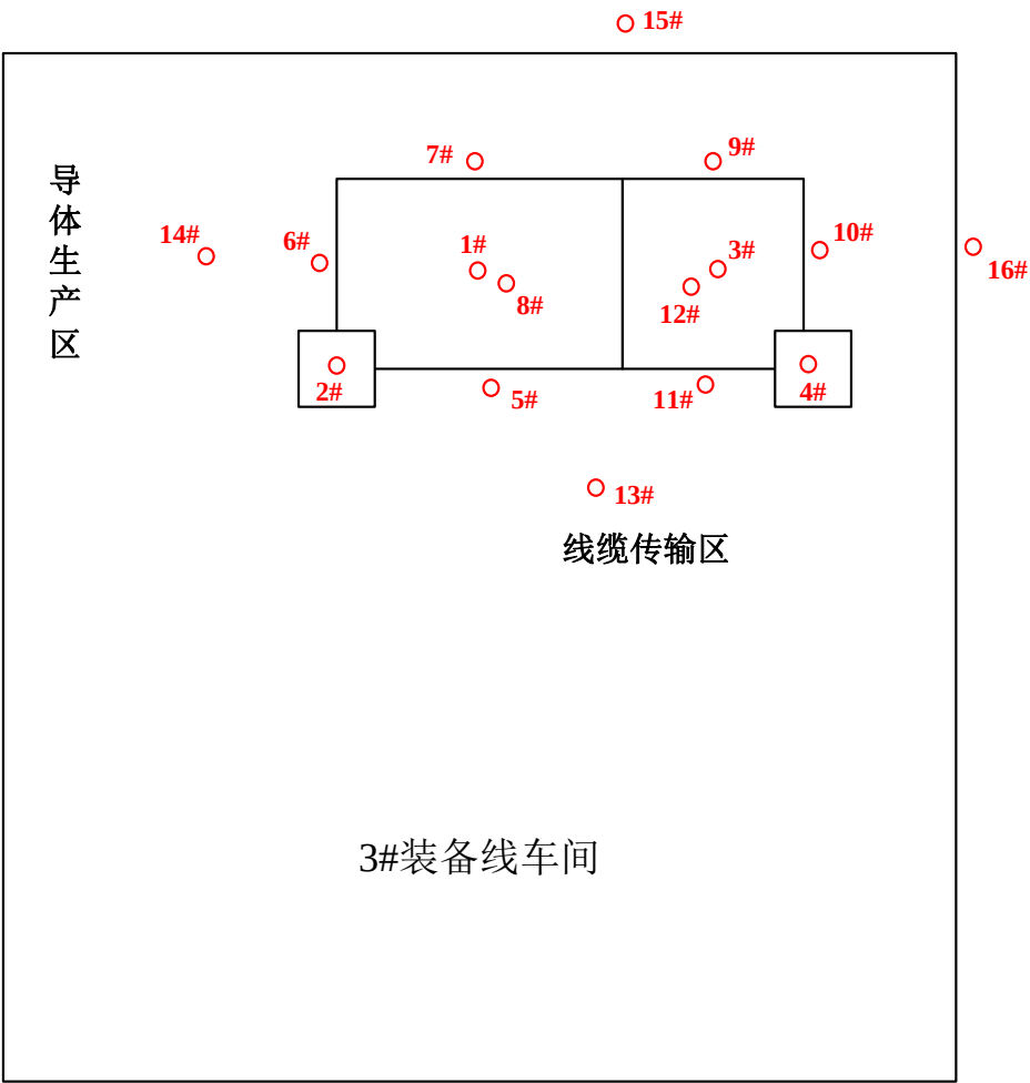
图8-1 项目监测布点示意图
