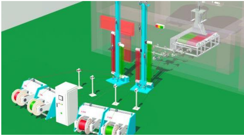
图9-7 束下传输系统示意图
