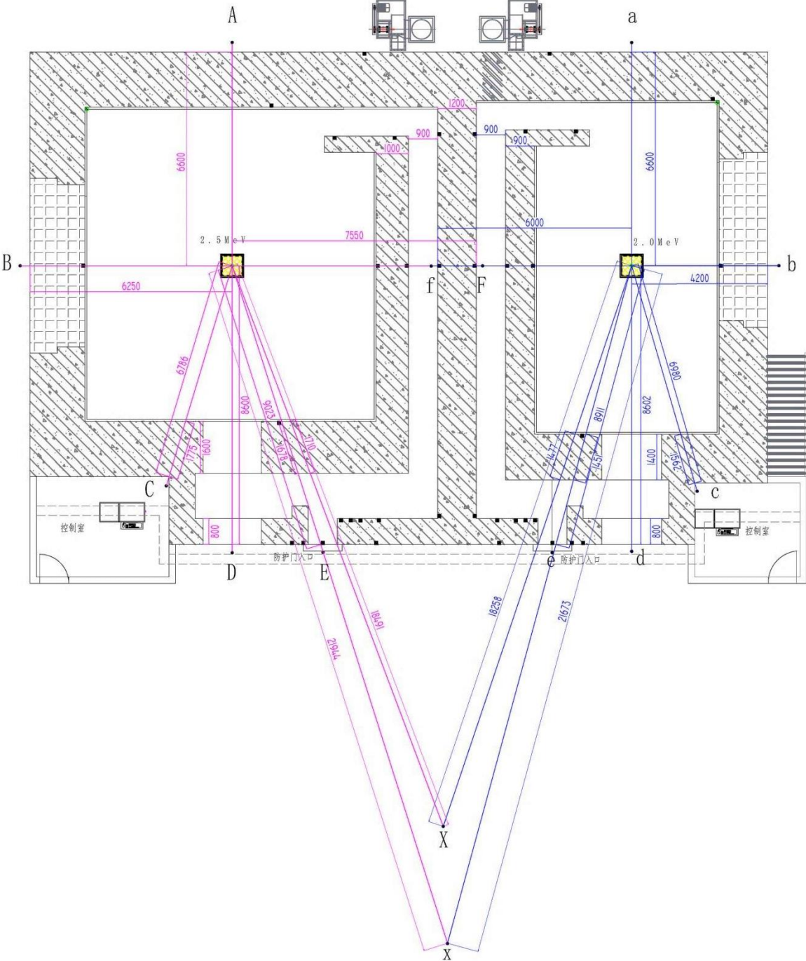
图11-1 辐照室X射线透射屏蔽效能平面核算示意图
