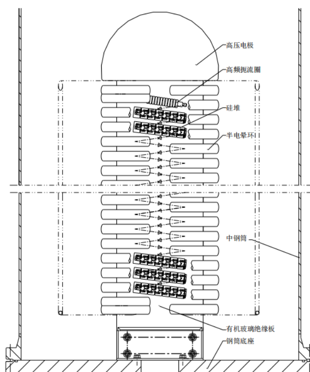
图9-3 整流倍压系统示意图
