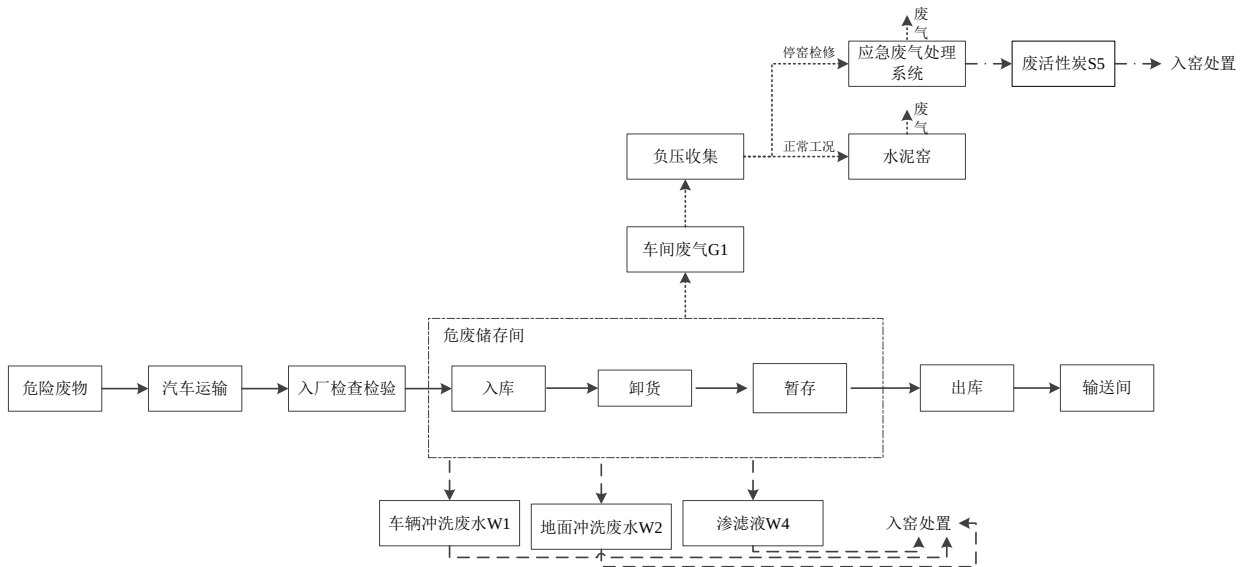
图 4.4-5 危废暂存库工艺流程图
