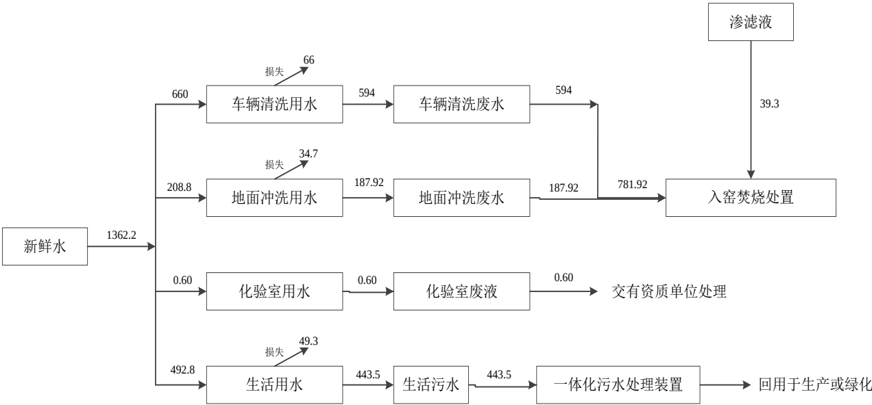
图 4.5-1 拟建项目水平衡图 (m³/a)
