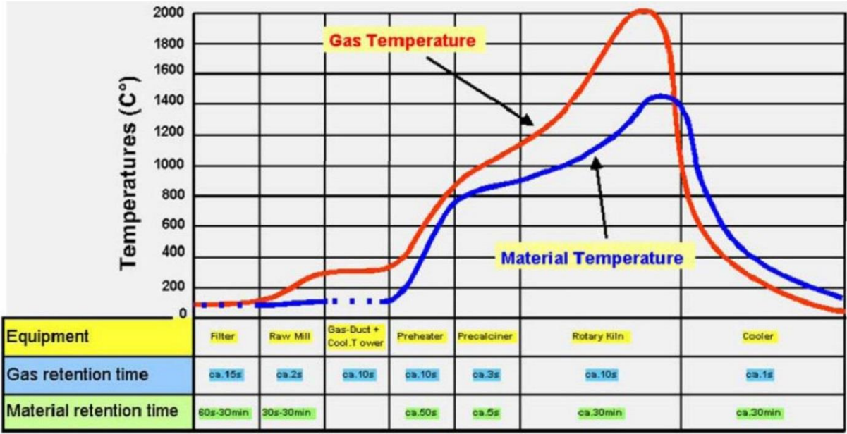
图 4.4-3 新型干法水泥窑窑内的气固相温度分布和停留时间
