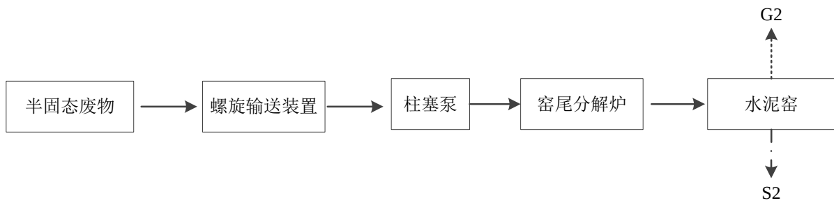
图 4.4-7 输送、投加、焚烧系统工艺流程图
