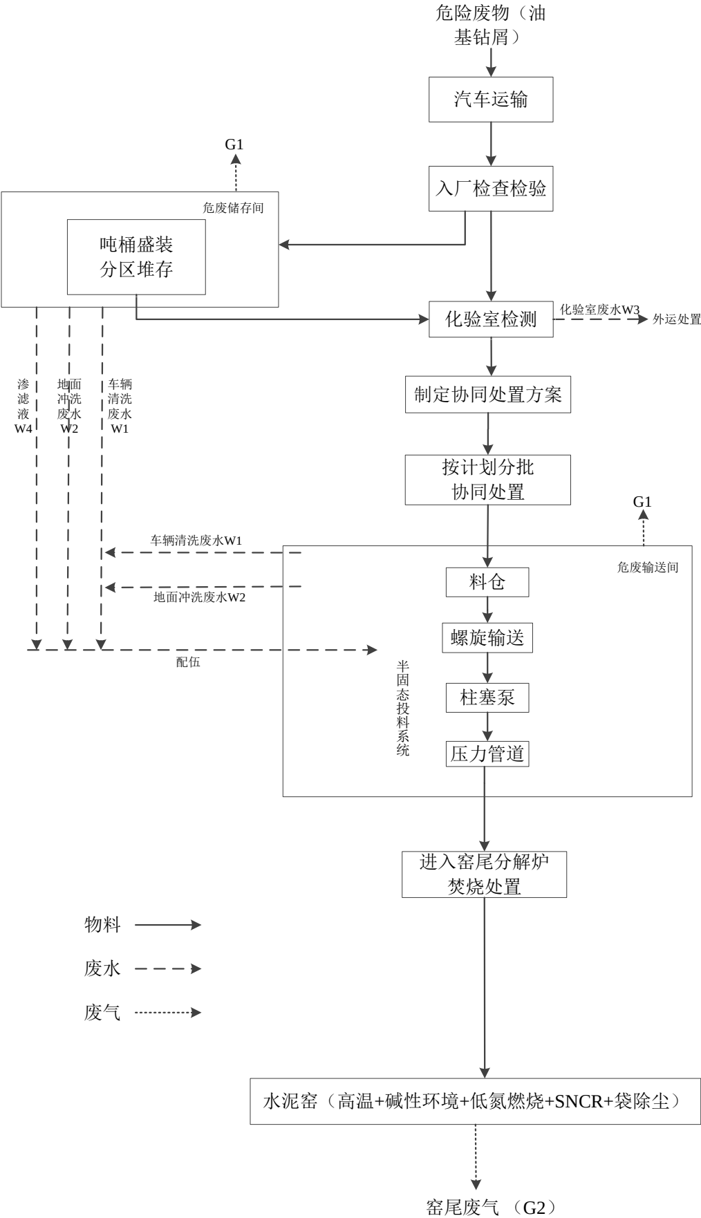
图 4.4-4 固体废物协同处置总体工艺流程图
