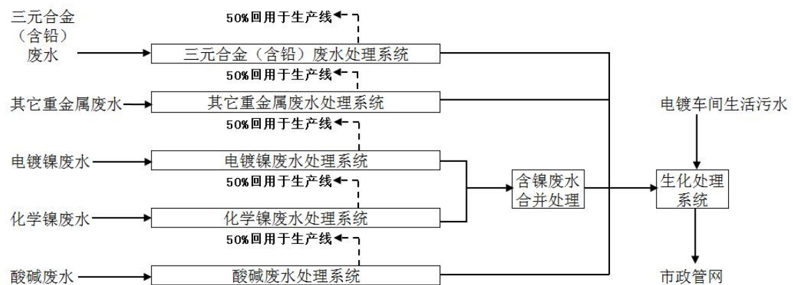
图 8.3-2 电镀废水处理系统总工艺流程图
