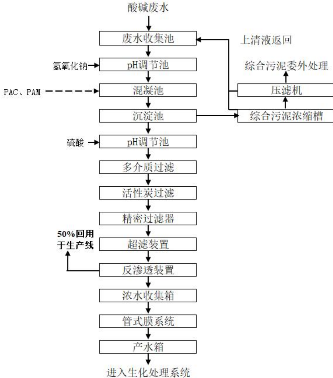
图 8.3-6 酸碱废水处理系统工艺流程图
