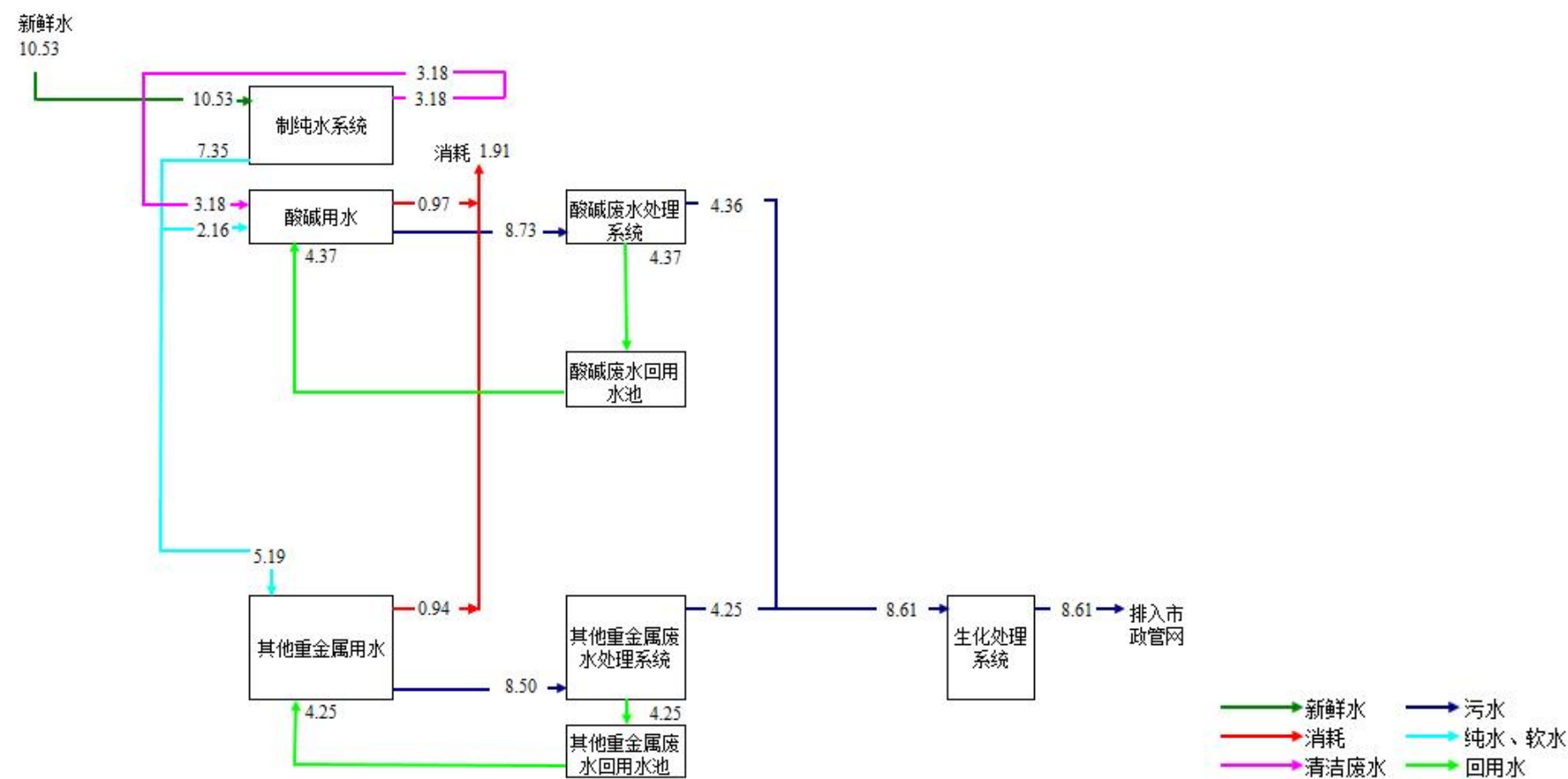
图 4.3-2 铜瓦镀锡线（电镀）水平衡图 单位：m³/d
