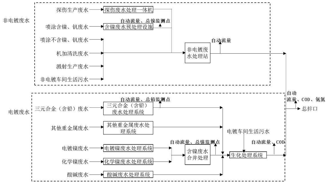
图 8.3-1 全厂污水处理收集处理监控示意图
