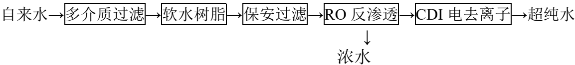
图 3.6-2 超纯水制备工艺流程
