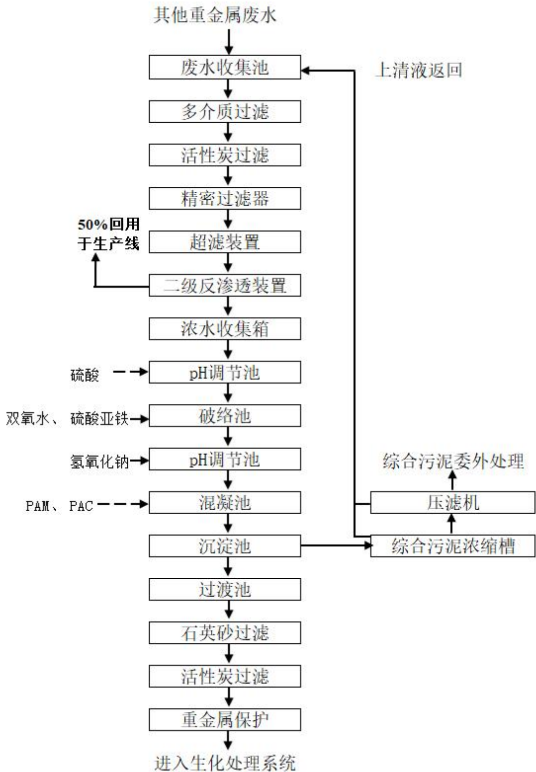
图 8.3-4 其他重金属废水处理系统工艺流程图
