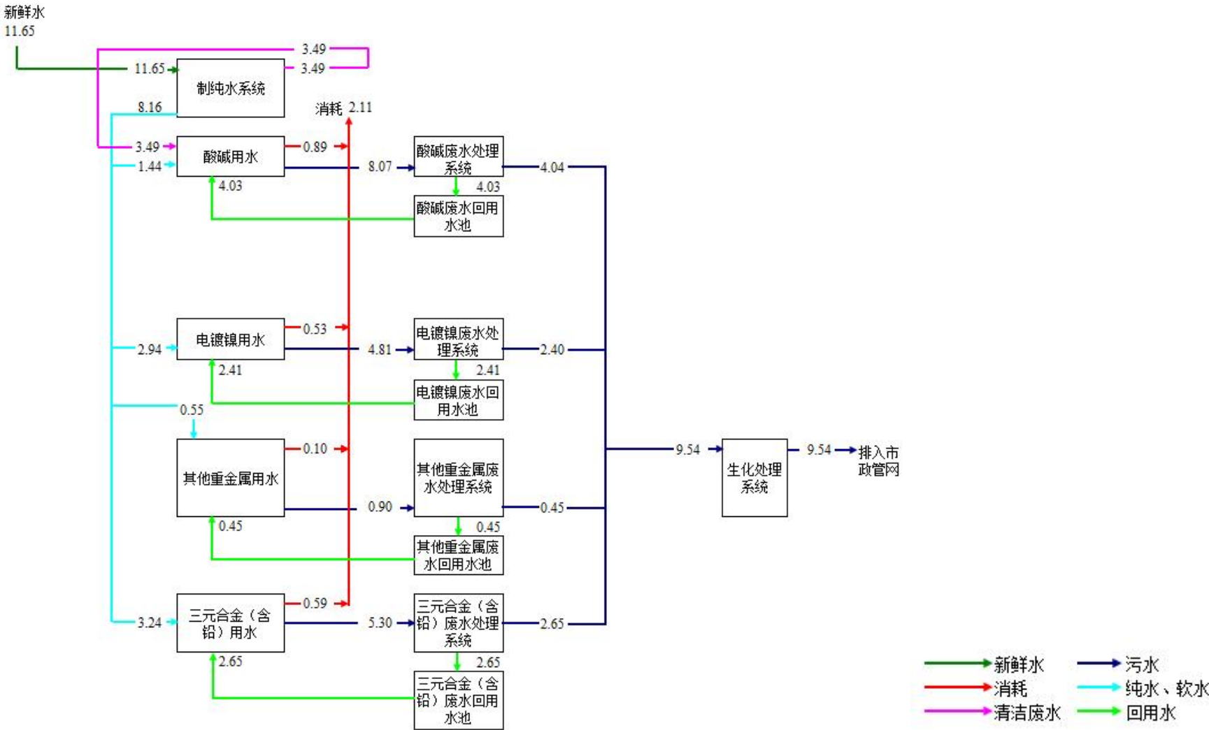
图 4.3-1 铜瓦铜套线（电镀）水平衡图 单位：m³/d
