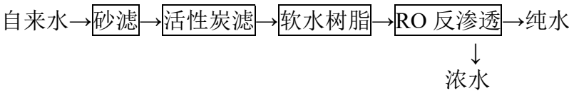
图 3.6-1 纯水制备工艺流程
