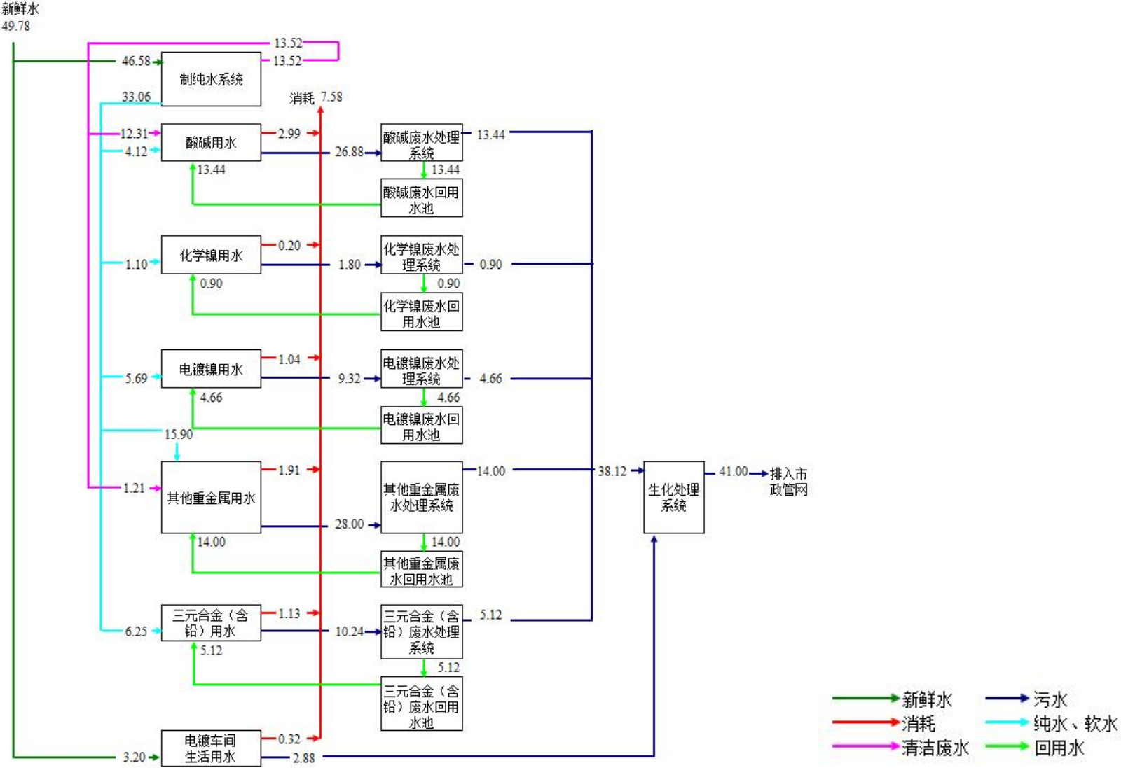
图 4.3-5 电镀车间总水平衡图 单位：m³/d
