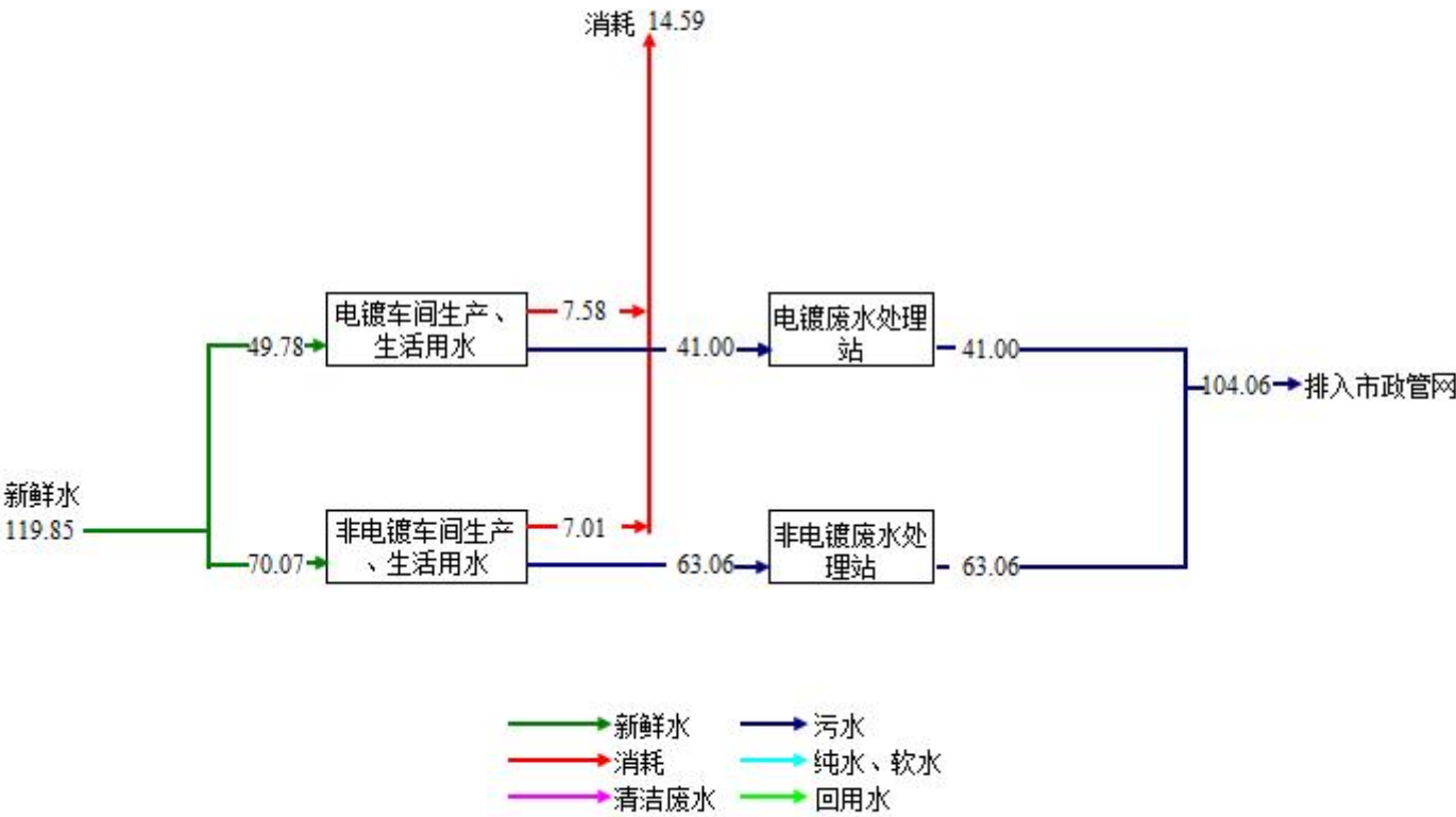
图 4.3-7 全厂水平衡图 单位：m³/d
