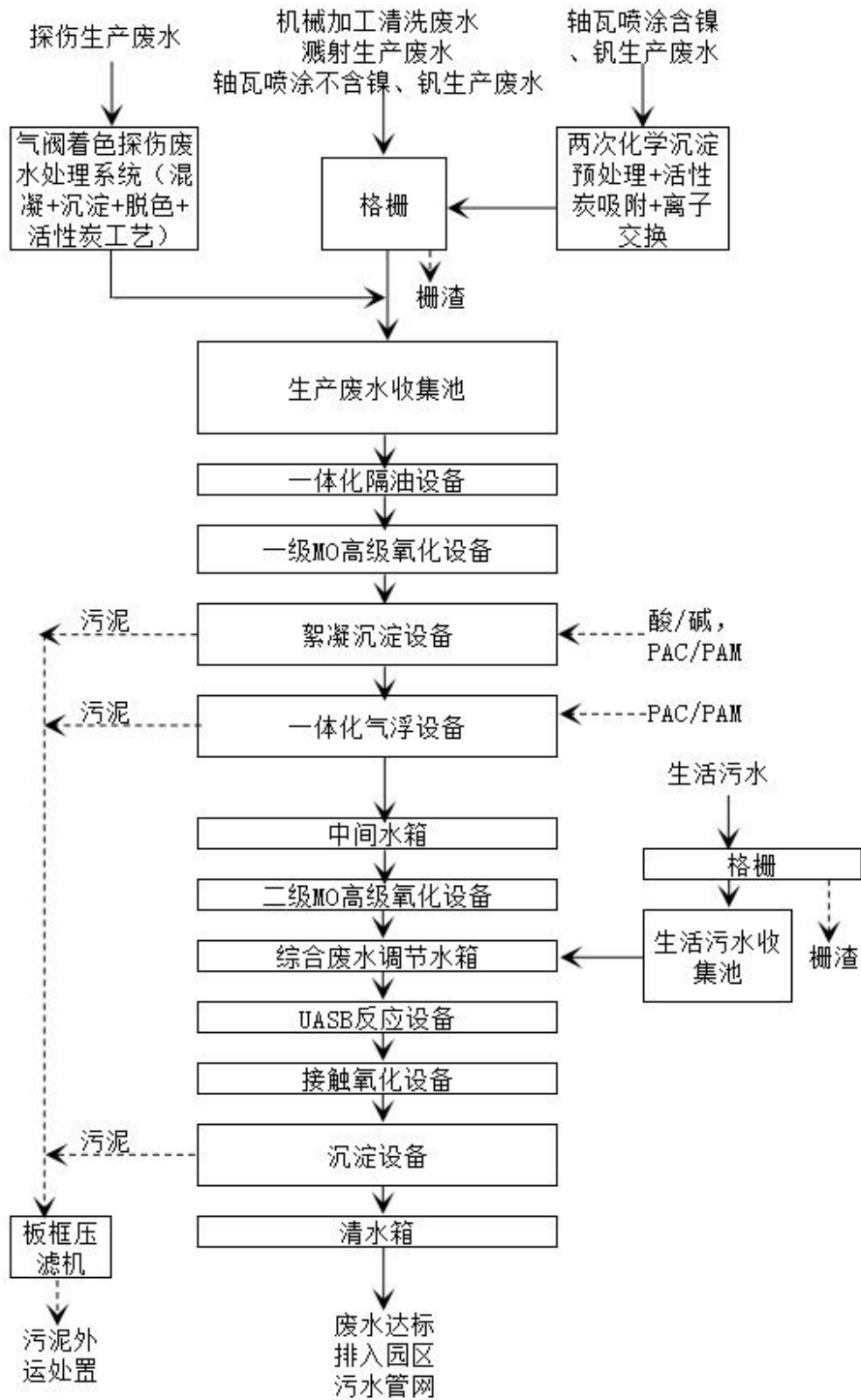
图 8.3-7 非电镀废水处理站工艺流程图
