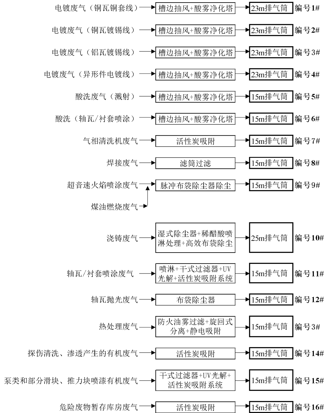
图 8.2-1 废气污染防治措施流程框图
