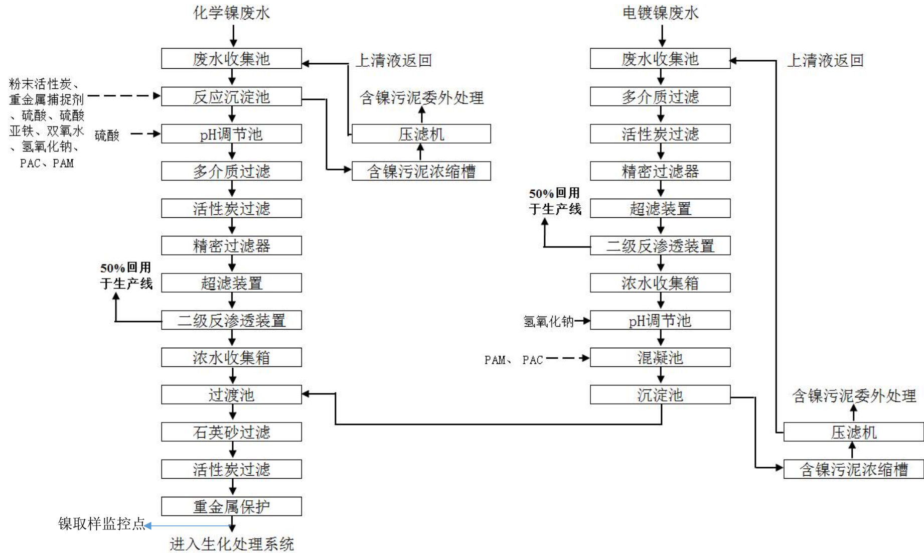
图 8.3-5 电镀镍和化学镍废水处理系统工艺流程图
