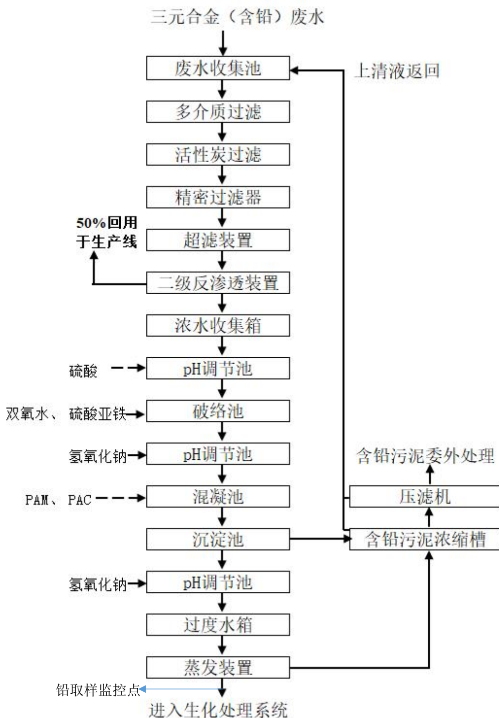
图 8.3-3 三元合金（含铅）废水处理系统工艺流程图
