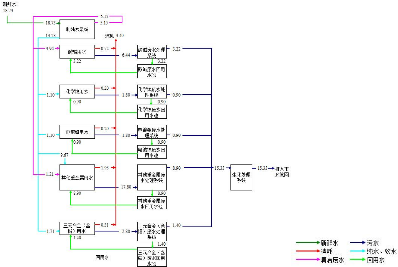
图 4.3-3 铝瓦镀锡线（电镀）水平衡图 单位： m^3/d
