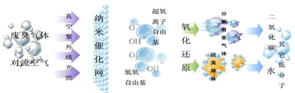
图 8.2-2 UV 光催设备化原理图
