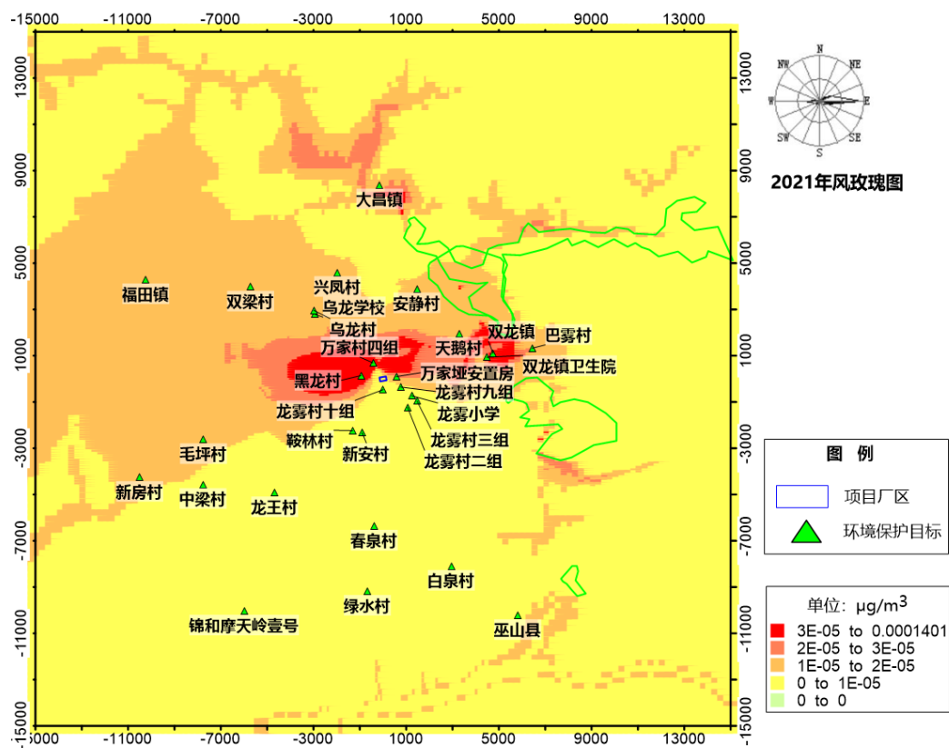
图 6.1.6-14 铅叠加年平均浓度影响分布图
