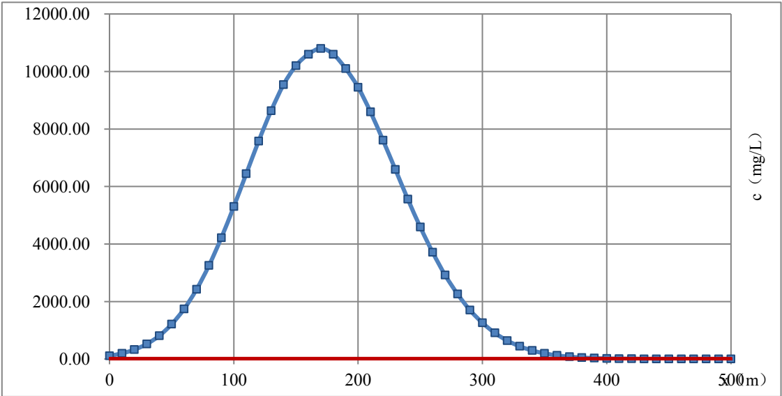
图 6.4.4-2 第 1000 天时污染物浓度与距离变化关系图（COD）
