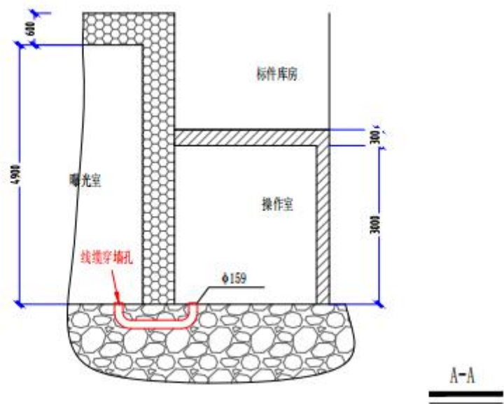
图 10-3 项目穿墙管线剖面示意图 (线缆管)
