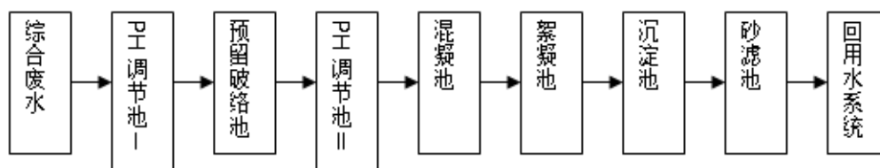
图 7.2-2 综合废水处理工艺
