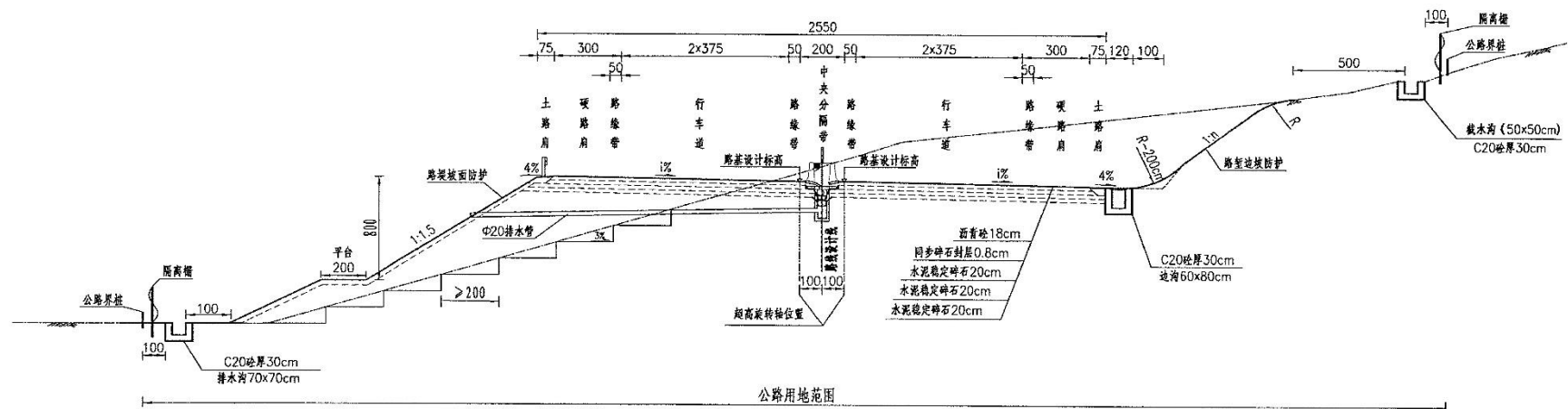
图 2.5-1 路基标准横断面示意图
