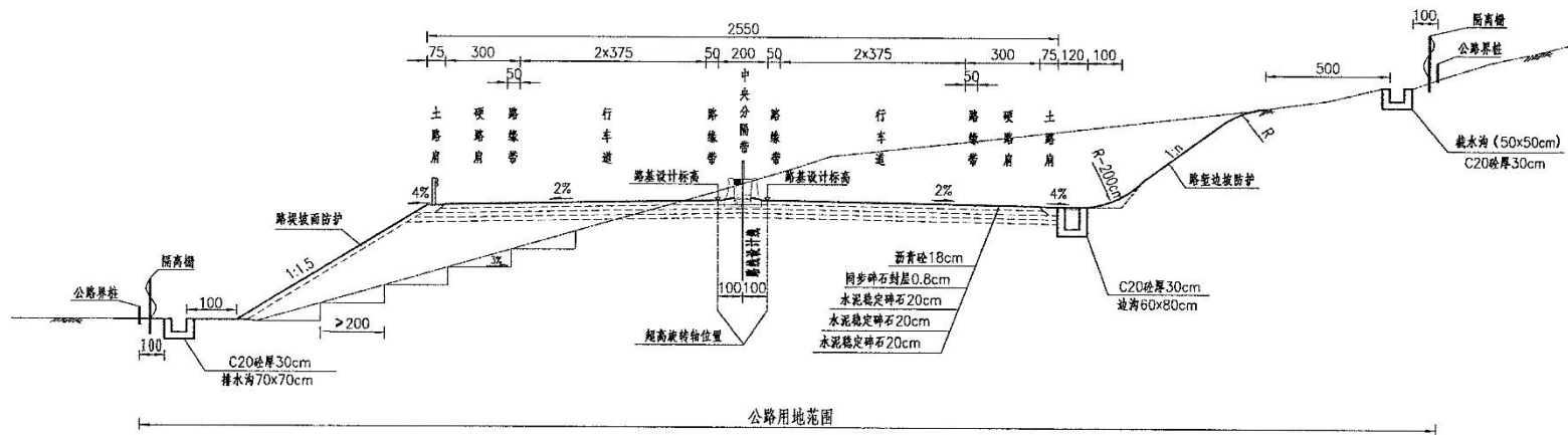
主线整体式路基标准横断面(超高路段)
