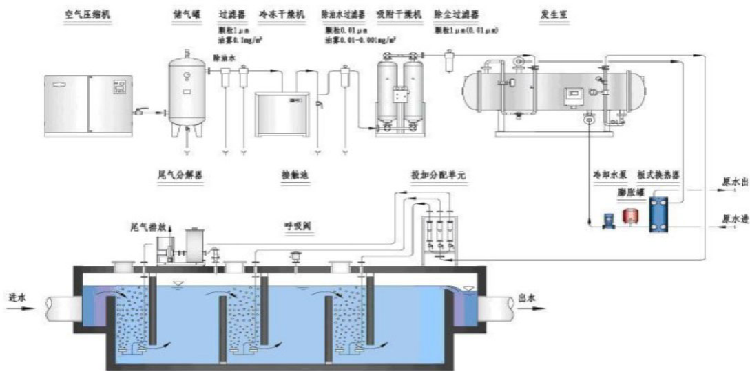
图 8.2—1 臭氧发生器工艺流程示意图
