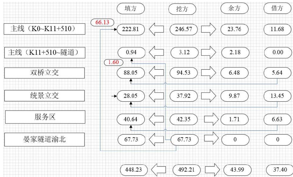
图 2-13 两江新区、渝北区段土石方平衡流向
