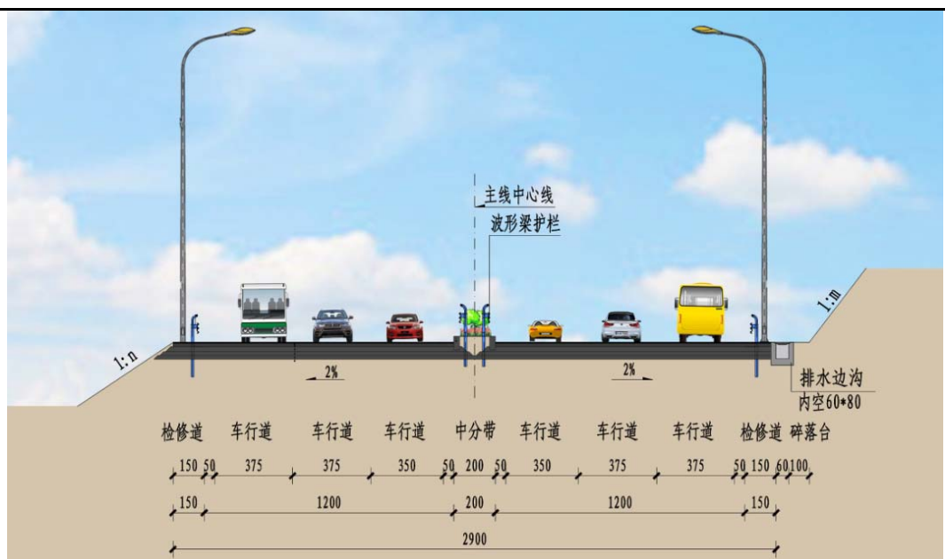
图 2-8 本项目（主线及三环连接道）标准横断面布置（全线近期）
