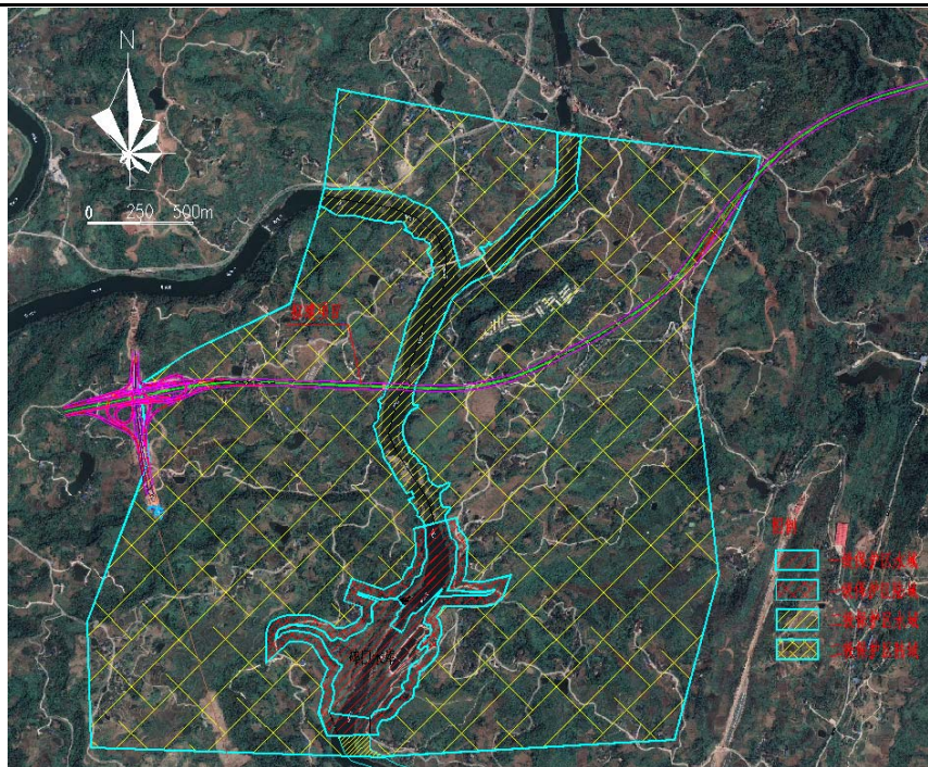
图 1-5 拟建项目与碑口水库保护区位置关系示意图
