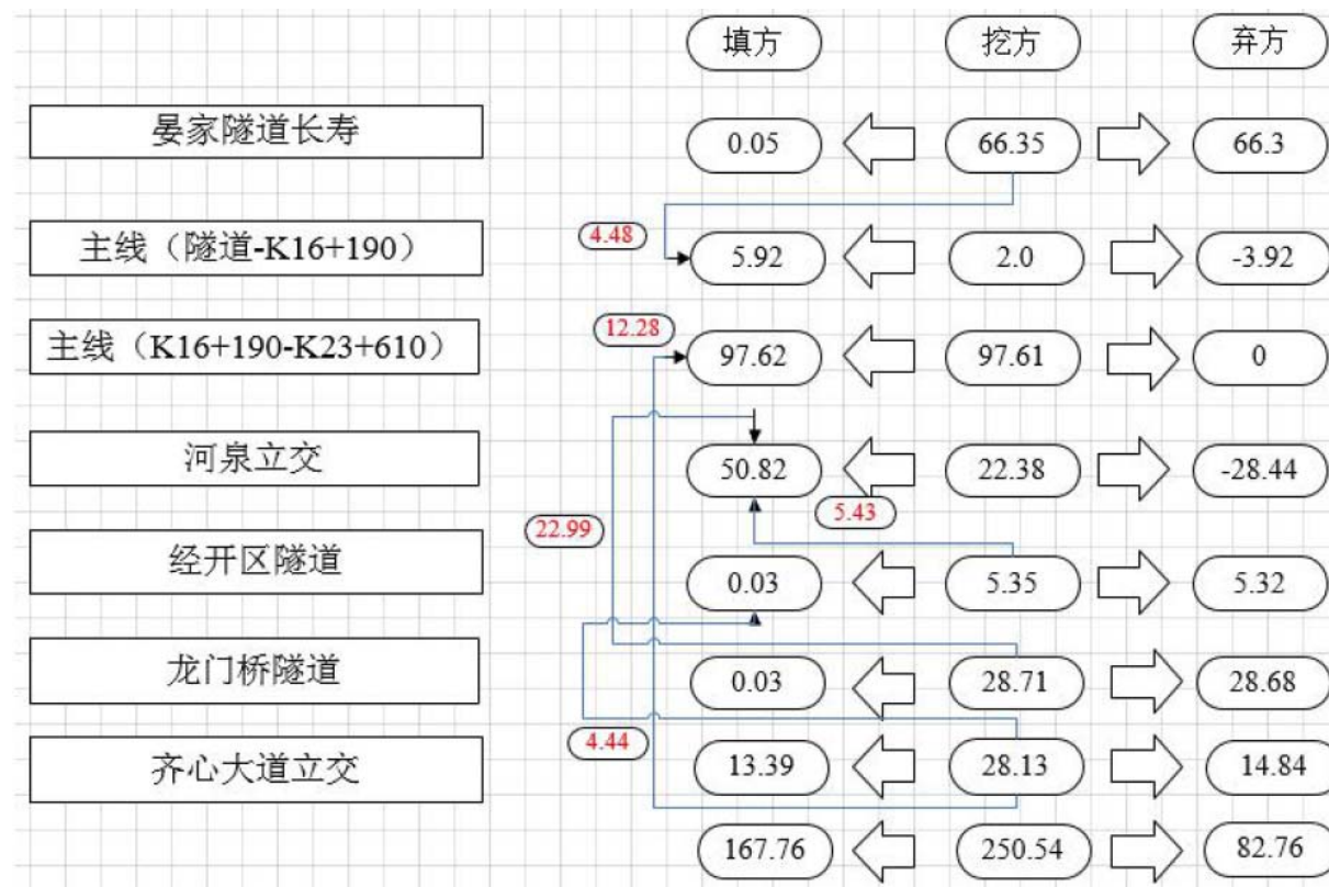
图 2.5-3 长寿区段土石方平衡流向图
