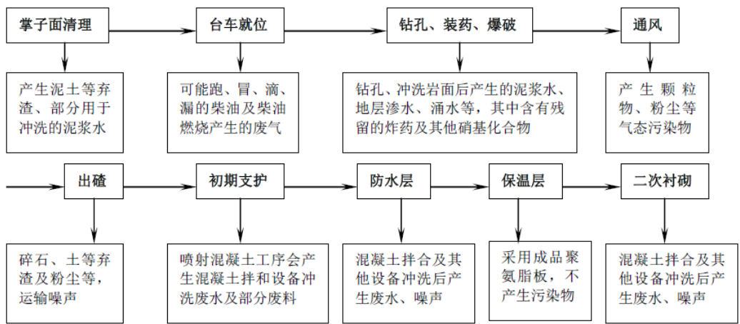
图 2-14 隧道施工工艺及产排污环节
