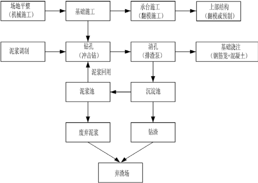
图 2-16 不涉水桥梁基础施工工艺
