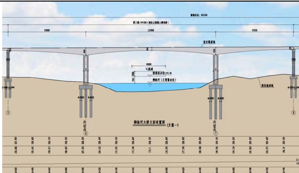
图 4-7 主桥立面布置图
