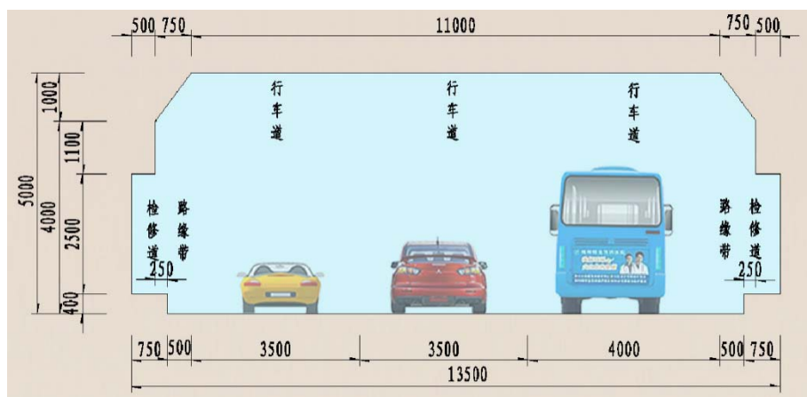
图 2-9 晏家隧道主线建筑限界（单洞）
