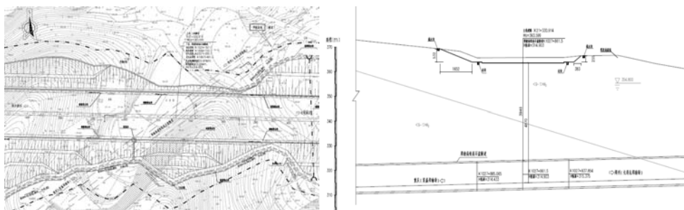
图 2-5 主线路堑段与郑渝高铁相交情况
