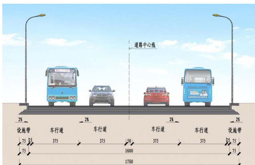
图 2-10 晏家联络道标准横断面布置
