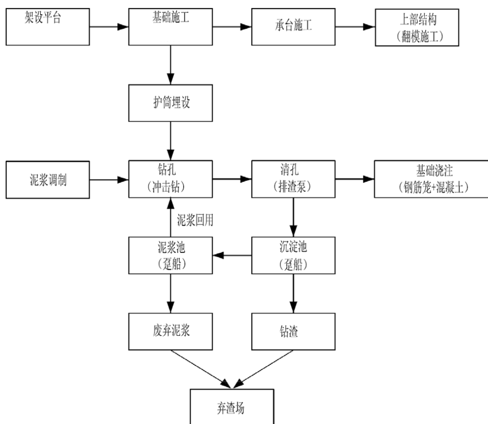
图 2-15 涉水桥梁施工工艺
