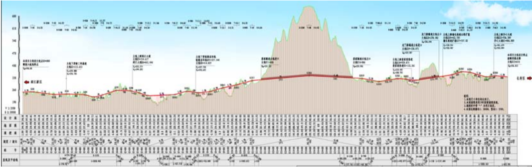
图 2-7 主线纵断面总图
