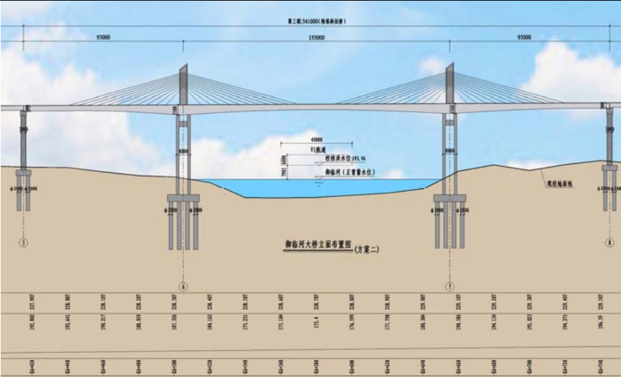
图 4-9 主桥立面布置图
