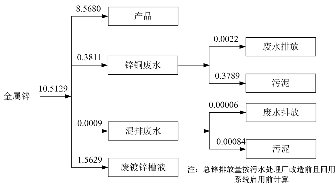
图 3.3.1-1 镀锌生产线锌平衡图 单位：t/a
