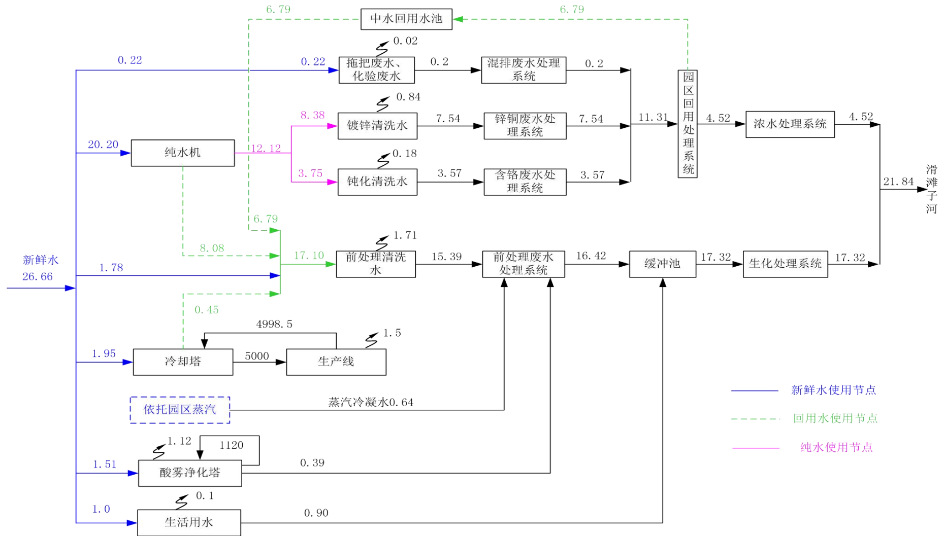
图 3.3.2-1 回用系统启用后拟建项目水平衡图 单位: m³/d
