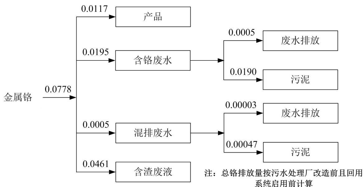
图 3.3.1-2 镀锌生产线钝化铬平衡图 单位：t/a
