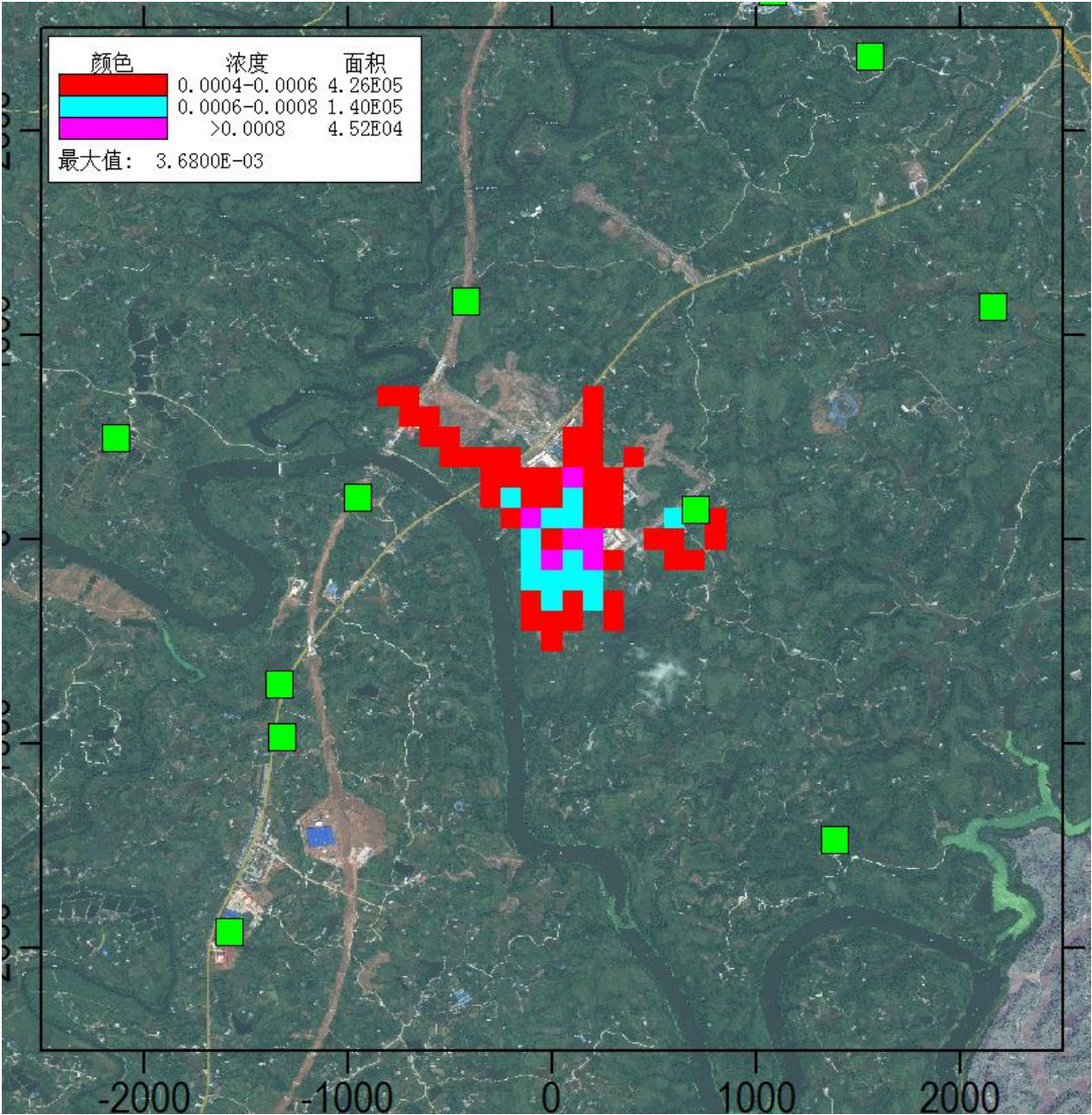
图 5.1-1 氯化氢日平均叠加浓度网格浓度分布图
