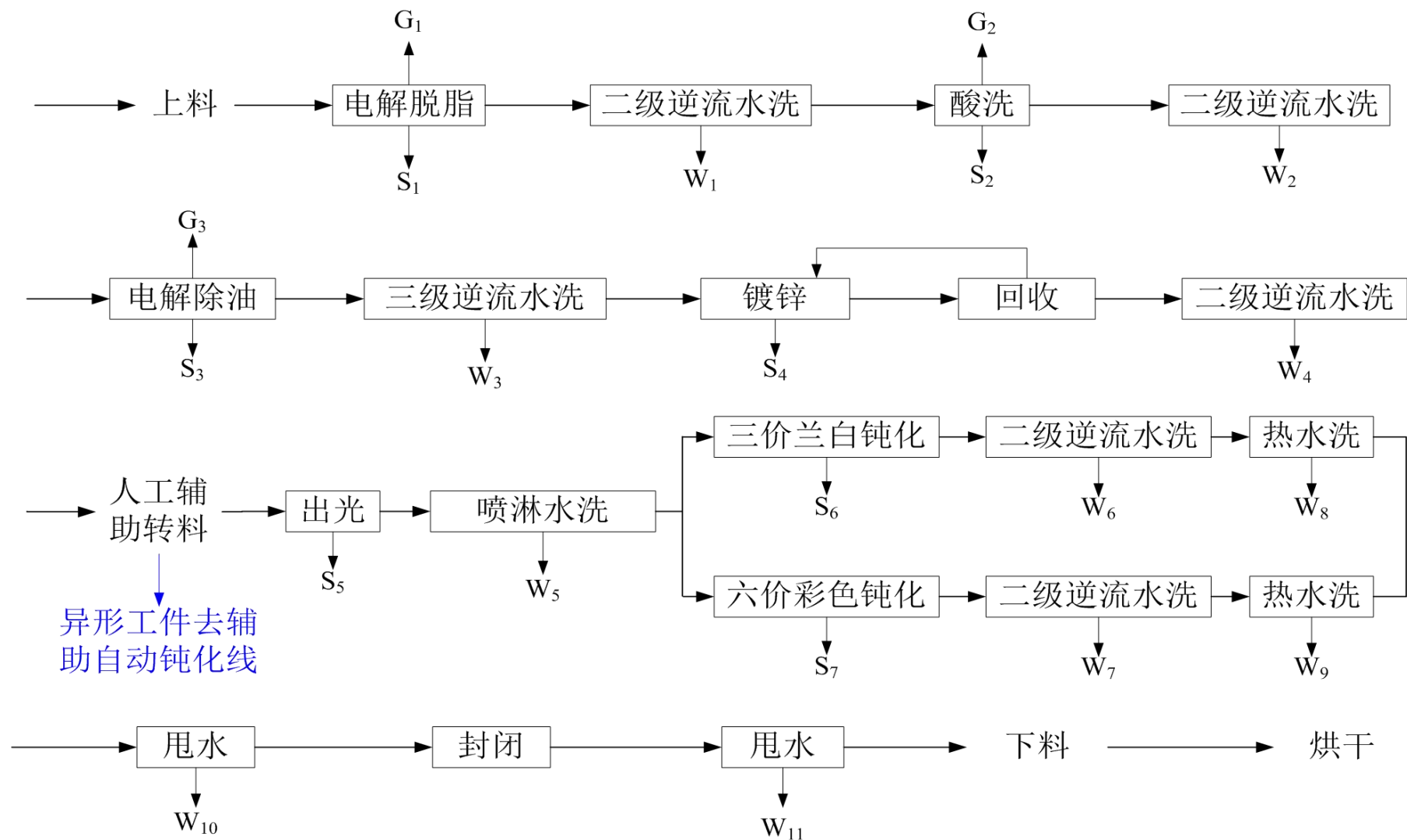
图 3.2.1-1 镀锌生产线工艺流程及产排污节点图
