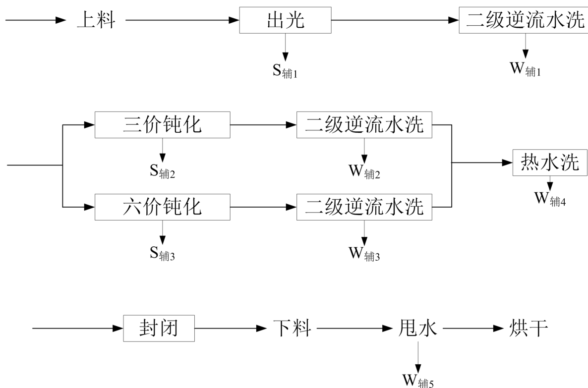
图 3.2.2-1 辅助自动钝化线工艺流程及产排污节点图
