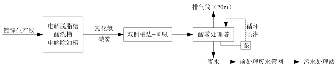
图 7.1.2-1 镀锌生产线碱雾、氯化氢净化装置处理流程图
