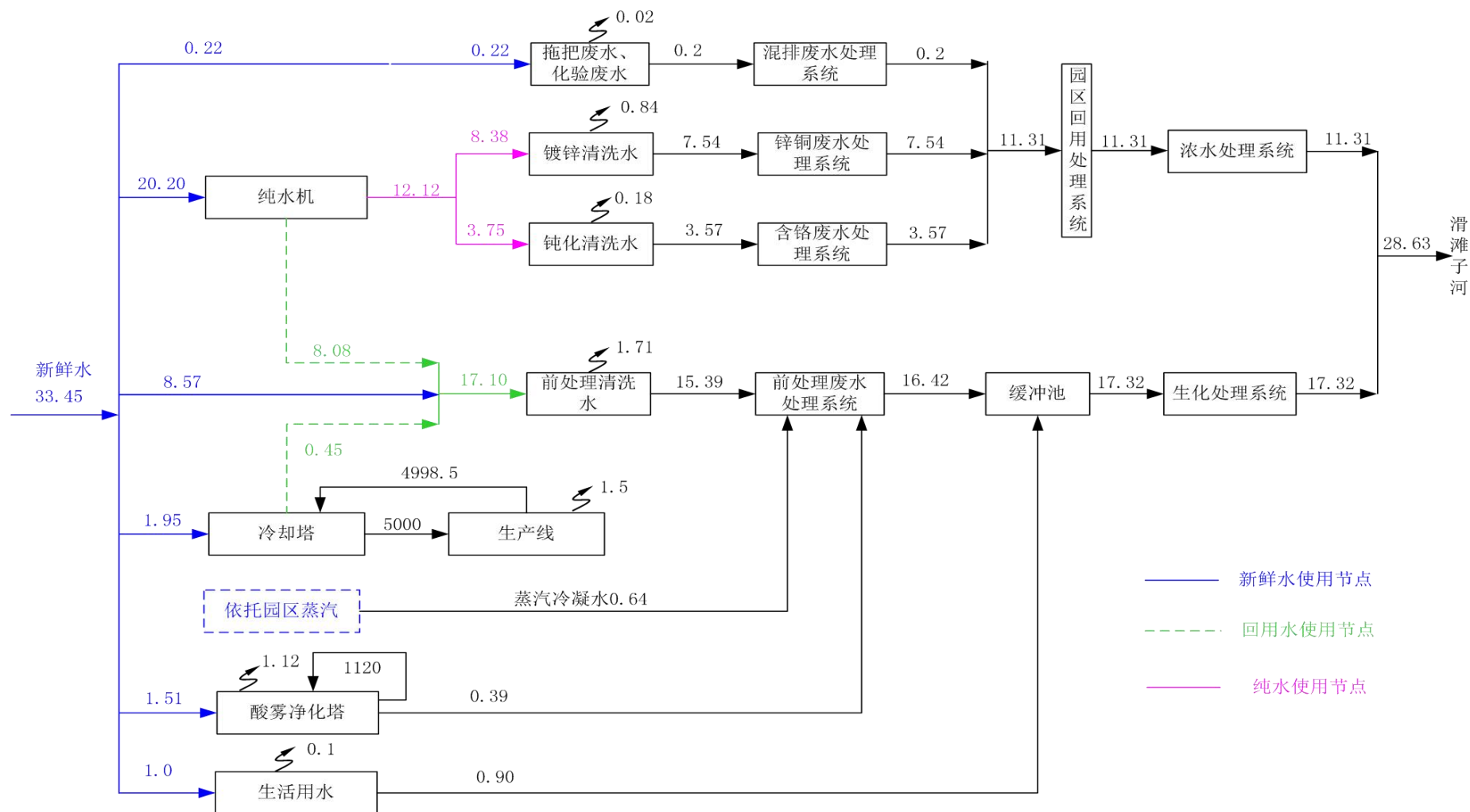
图 3.3.2-2 回用系统启用前拟建项目水平衡图 单位: m³/d
