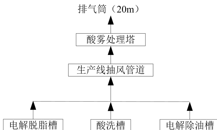
图 3.4.3-1 生产线废气收集示意图（酸雾处理塔）
