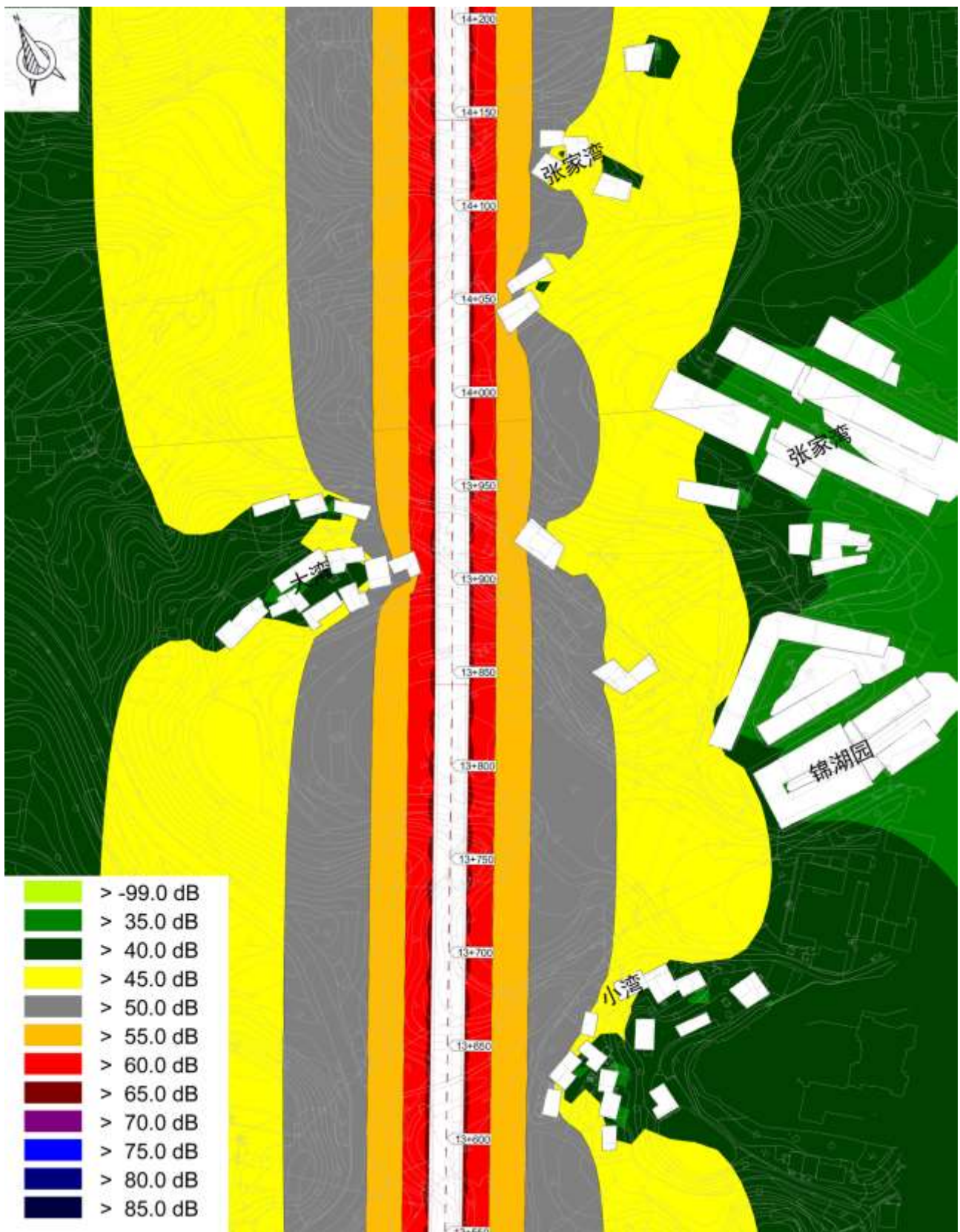
图 6-2-7 运营中期夜间等声级曲线图
