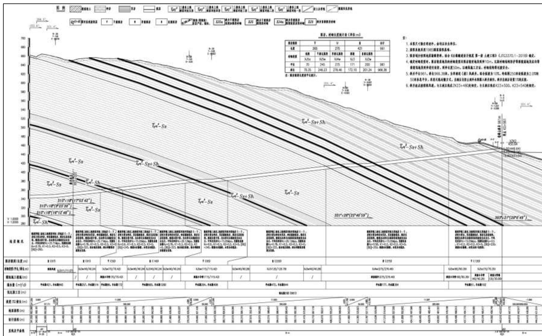
图 2-5-14 铁峰山隧道纵断面设计图
