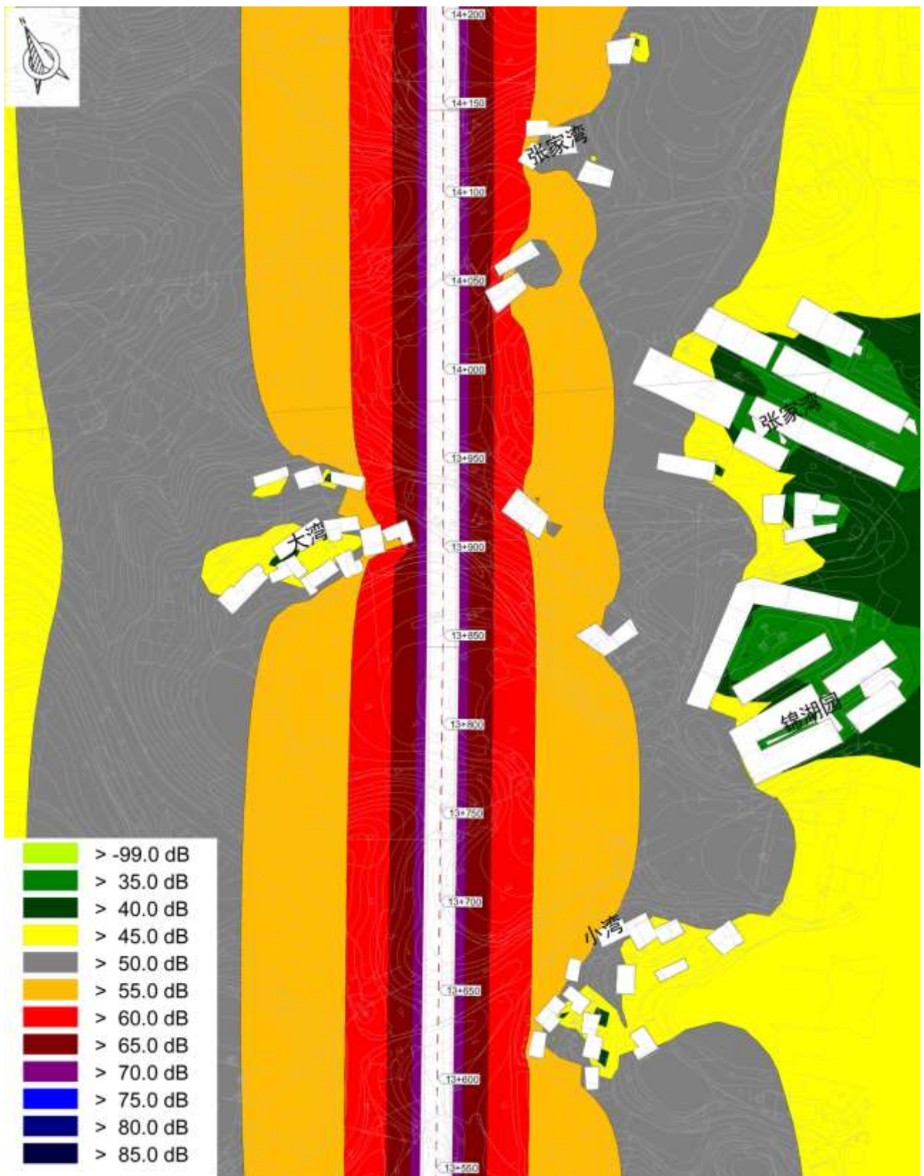
图 6-2-6 运营中期昼间等声级曲线图
