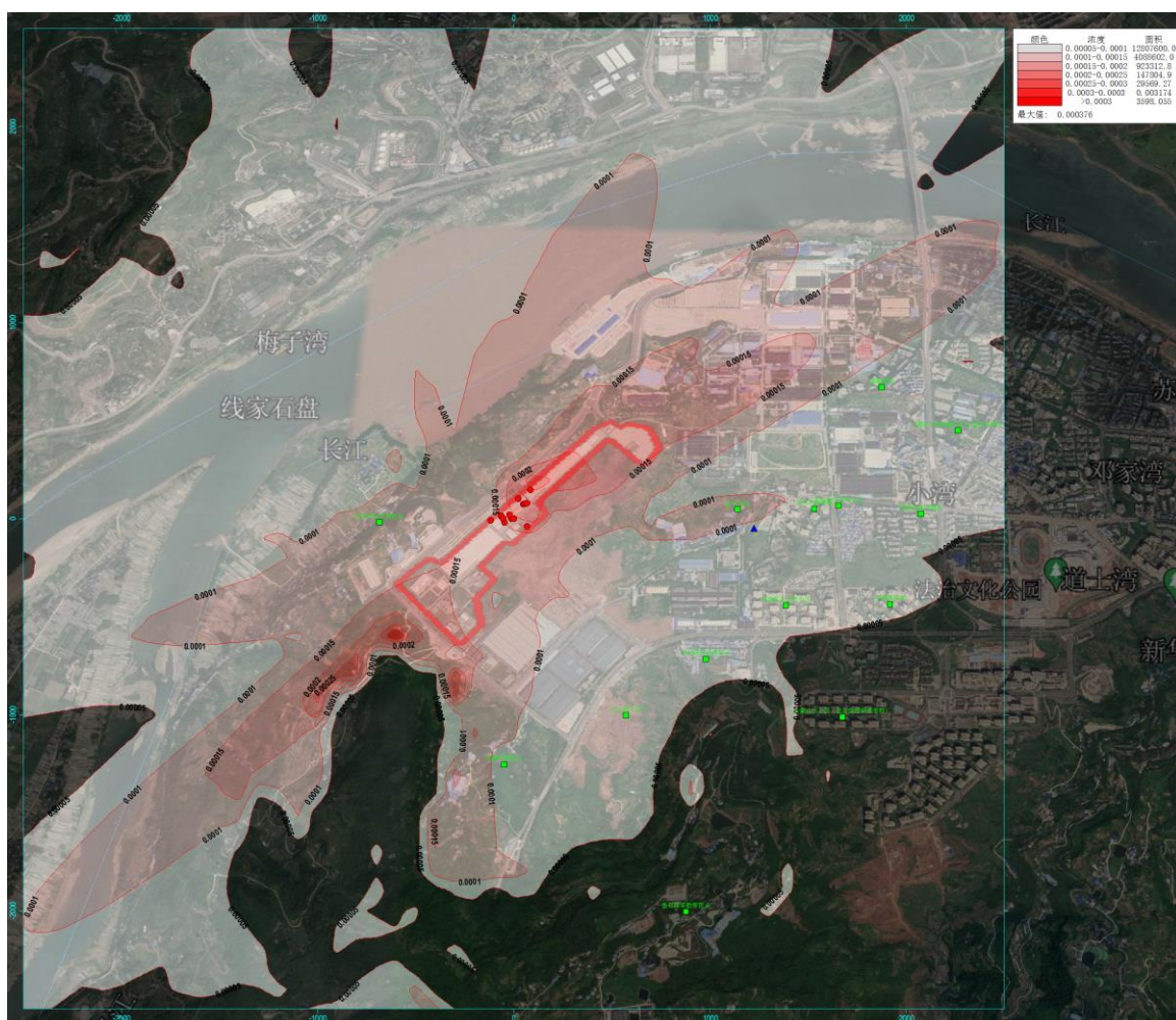
图 6.1.6 甲醛小时浓度叠加值分布图
