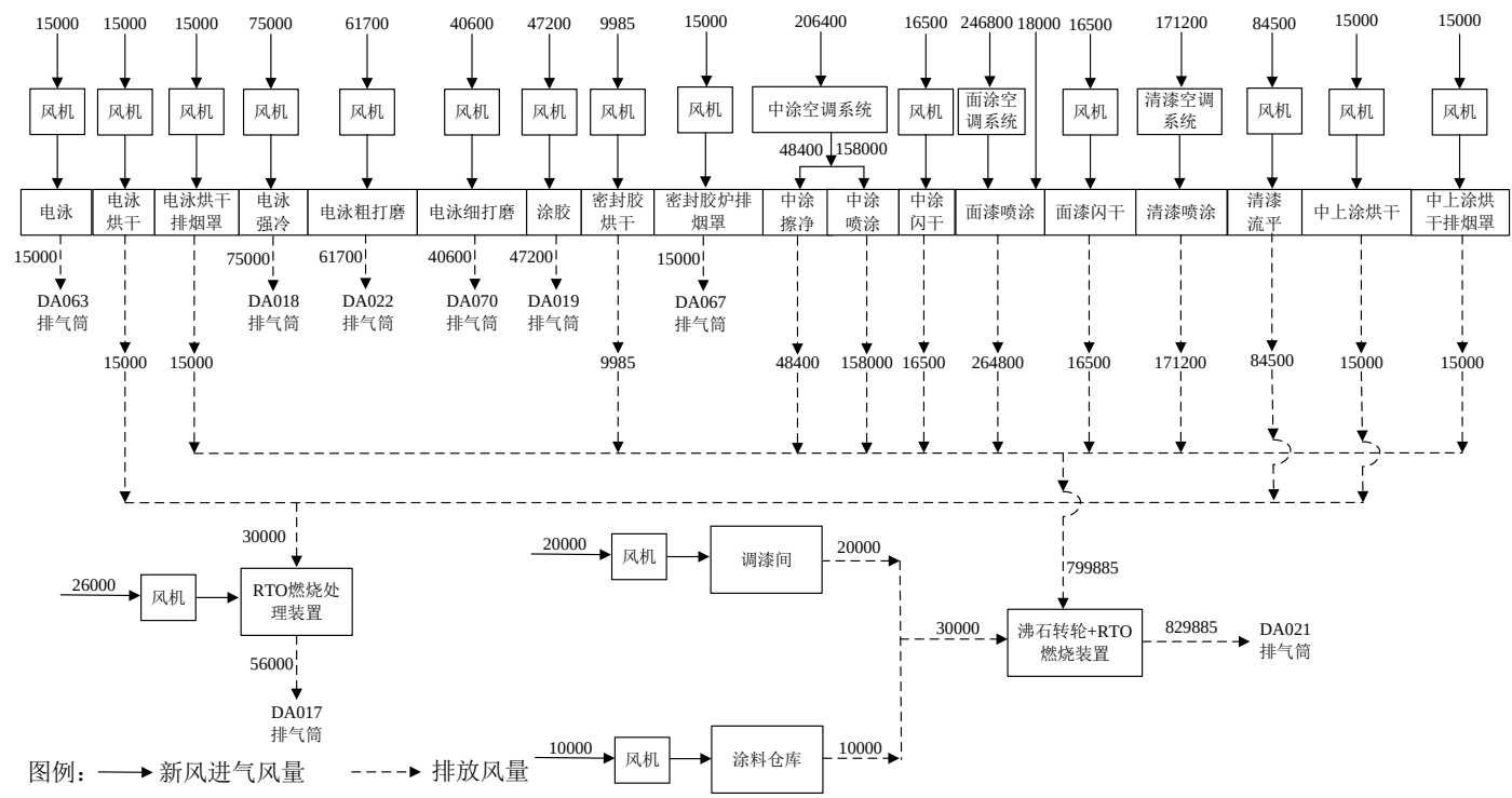
图 4.7.1 涂装车间风量平衡图 (m³/h)
