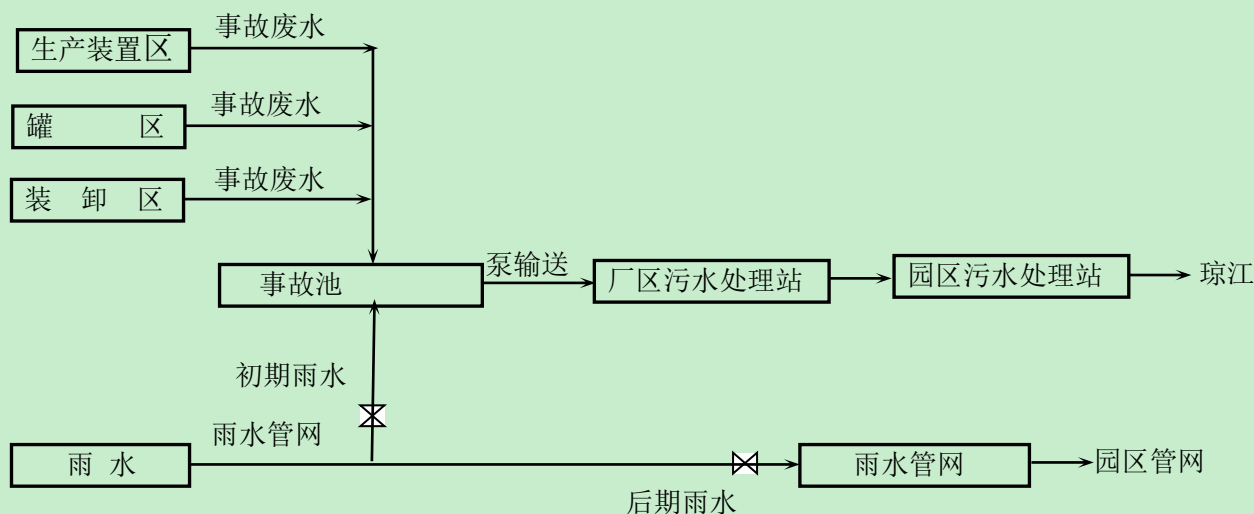
图 5.8.3-1 厂区事故废水收集处理系统图
