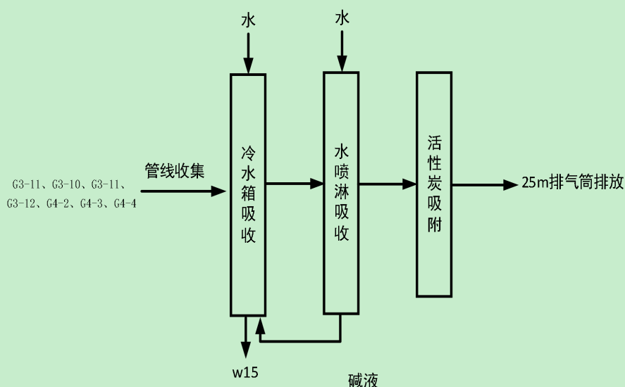
图2.2.8-4 含乙醇废气处理工艺
