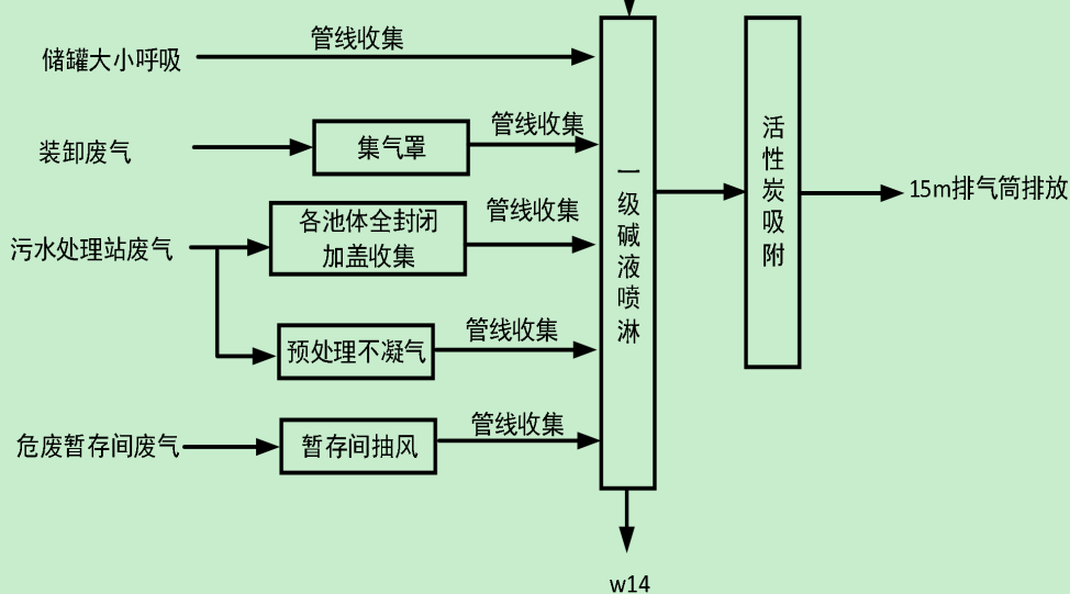
图2.2.8-3 罐区、污水处理、危废暂存废气处理工艺
