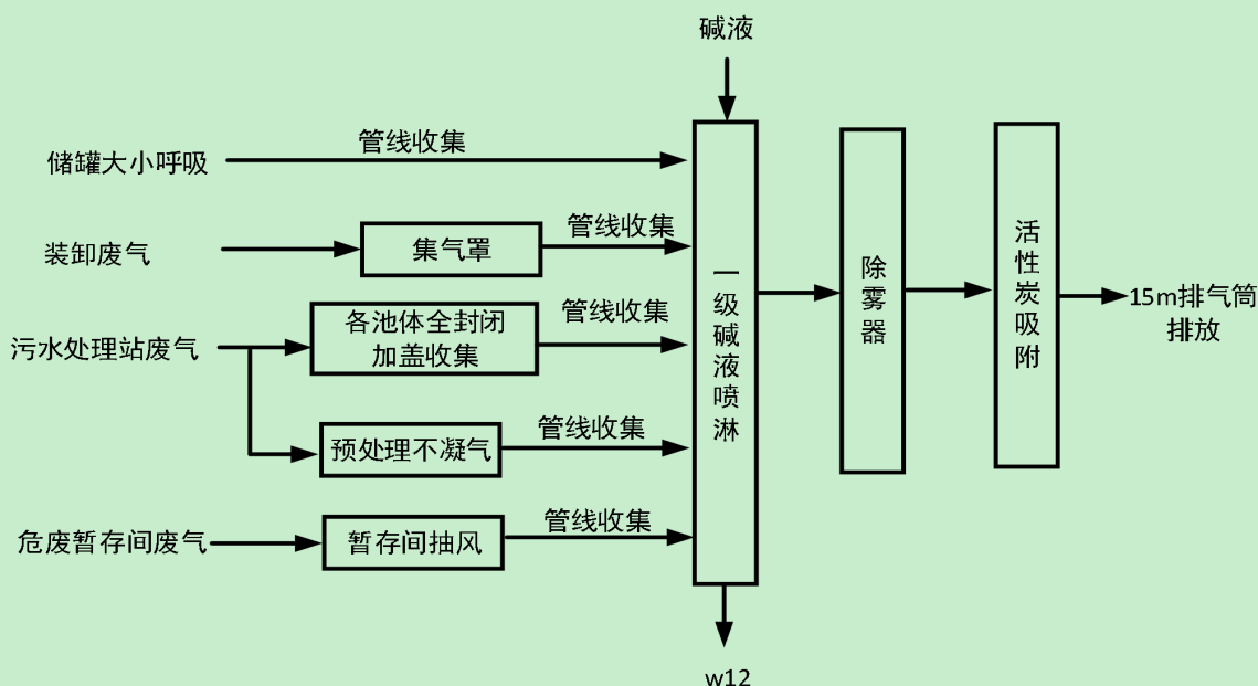
图6.1.2-4 罐区、污水处理、危废暂存废气处理工艺
