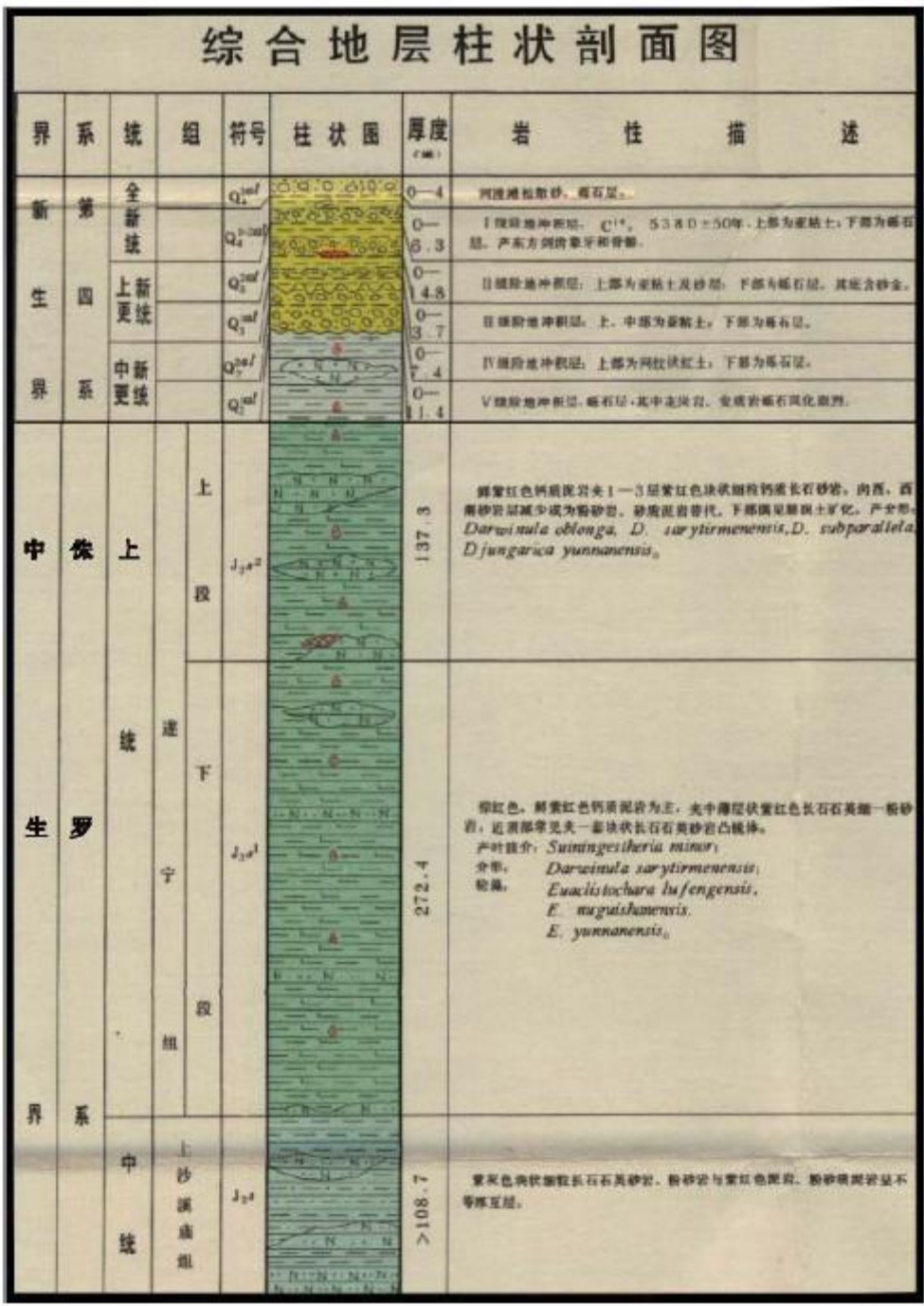
图 3.1-4 (2) 综合地层柱状剖面图
