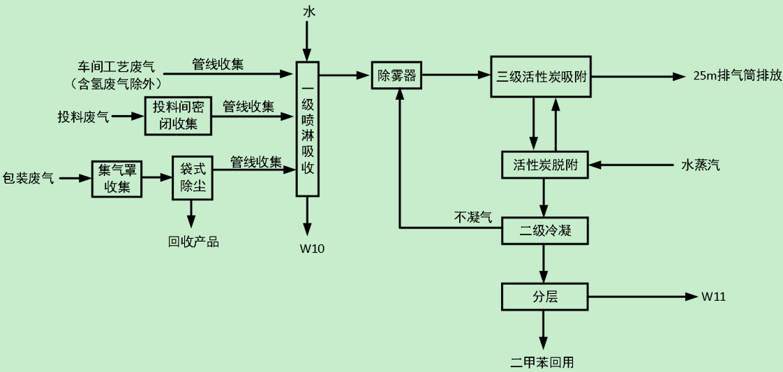
车间不含氢、乙醇废气处理工艺
