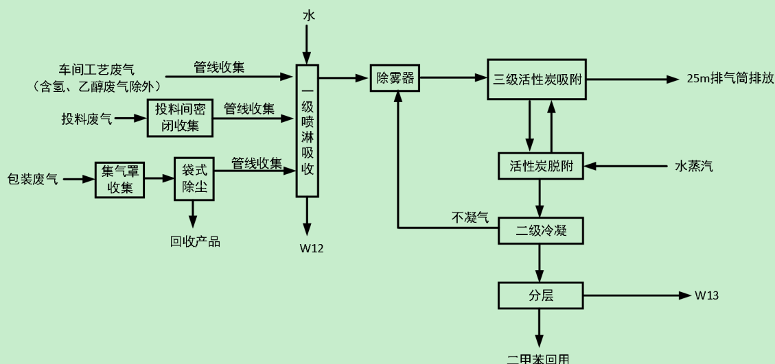
图2.2.8-1 车间不含氢废气处理工艺
