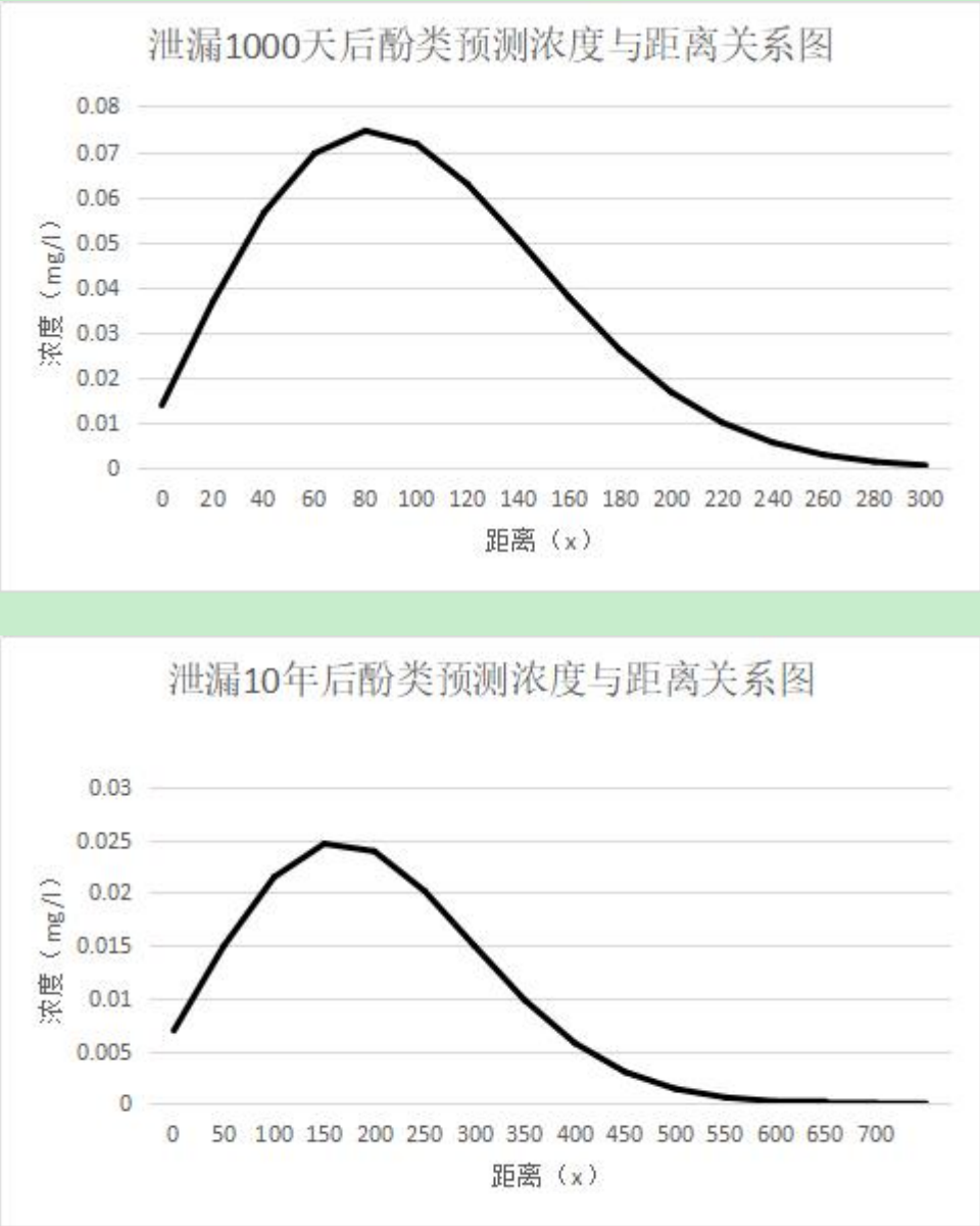
图4.2.3-3 挥发酚类浓度与距离变化关系图
