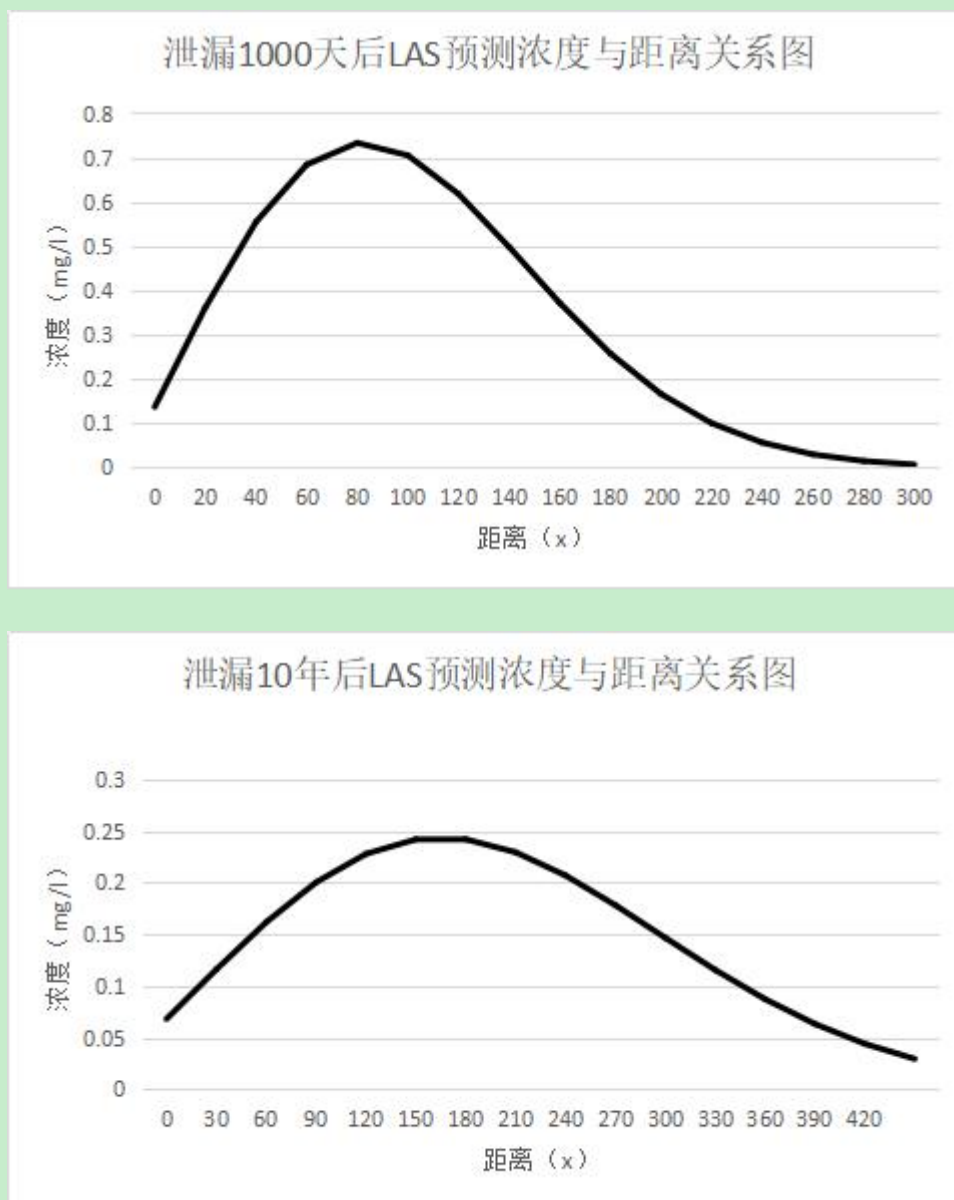
图4.2.3-4 LAS浓度与距离变化关系图
