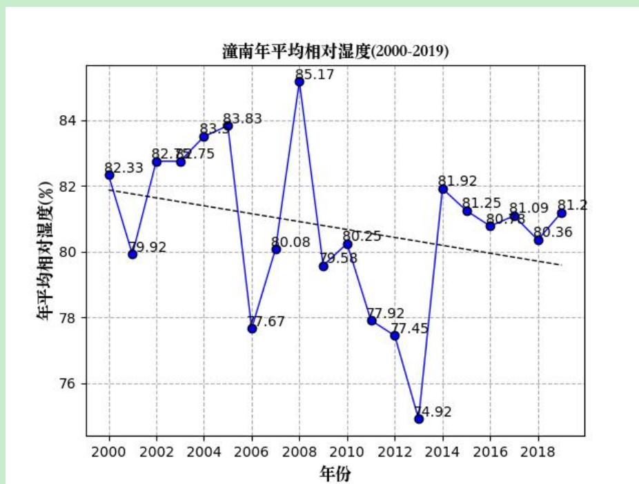
图 4.2.1-9 潼南（2000-2019）年平均相对湿度（纵轴为百分比，虚线为趋势线）
