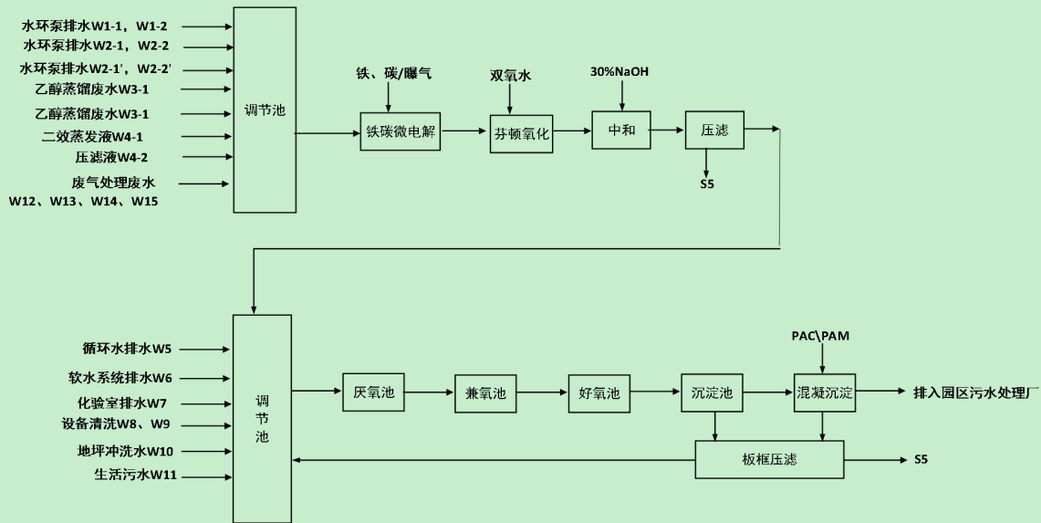
图6.2-1 污水处理工艺流程图
