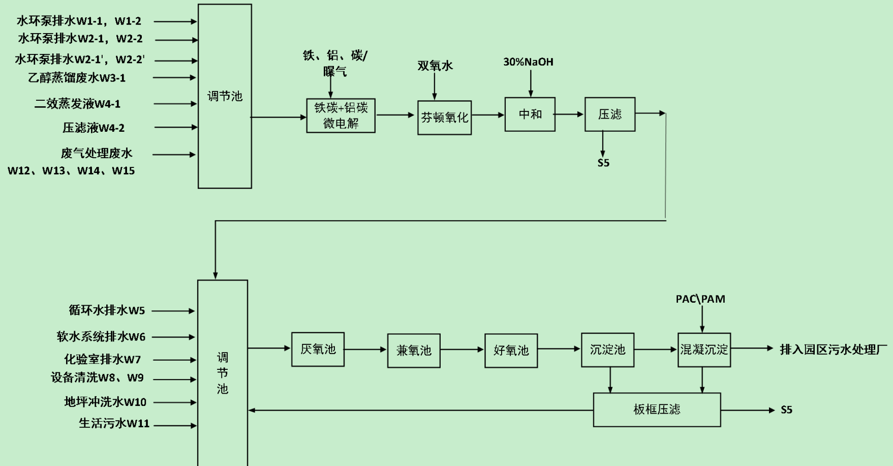
图2.2.8-5 污水处理工艺流程图
