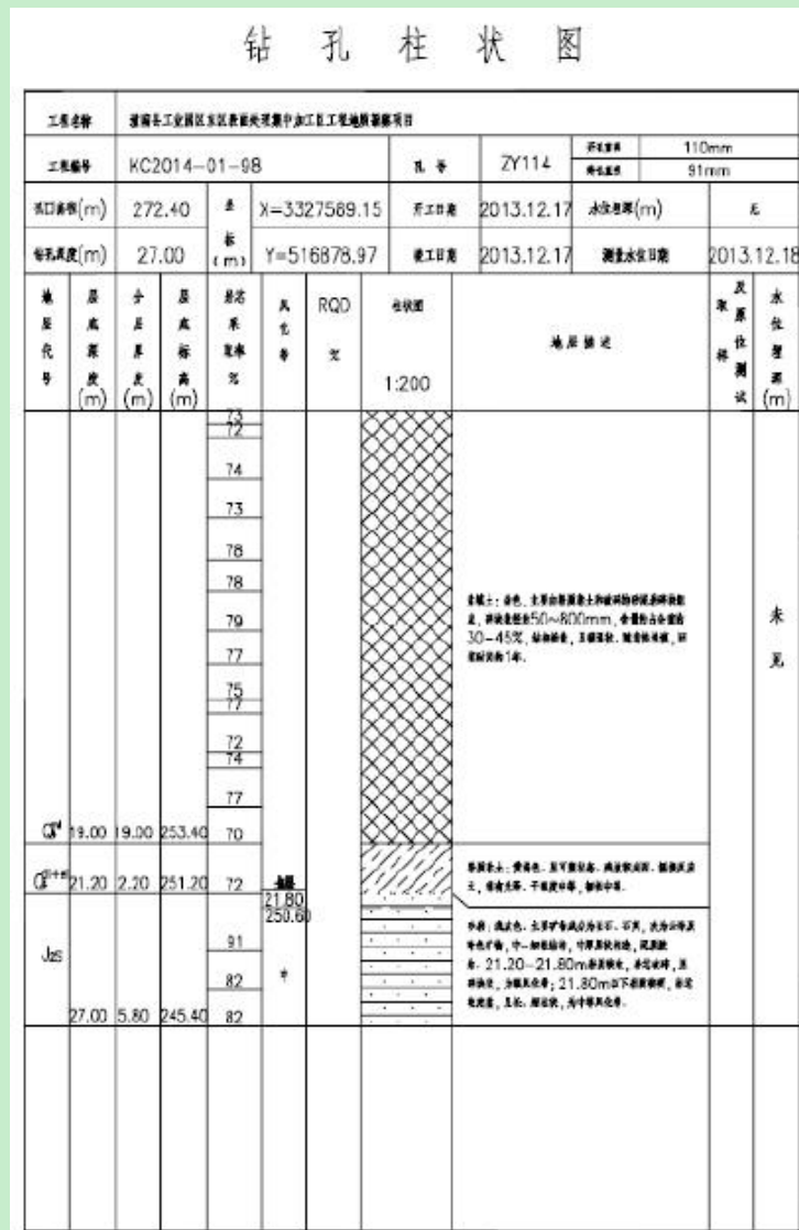
ZY 114 钻孔柱状图
