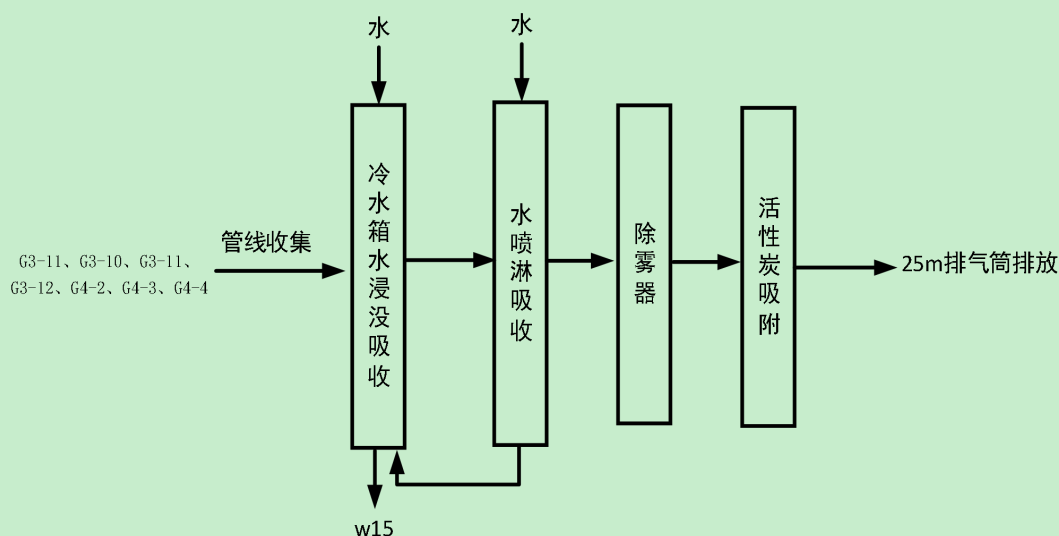
图6. 1. 2-5 含乙醇废气处理工艺流程图
