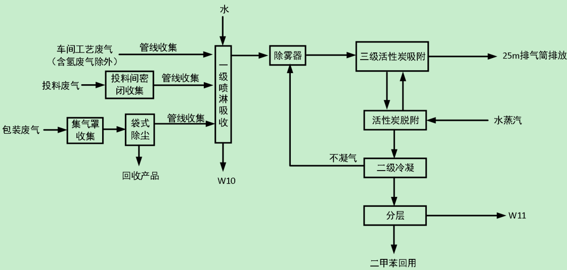
图6.1.1-2 车间不含氢、乙醇废气处理工艺
