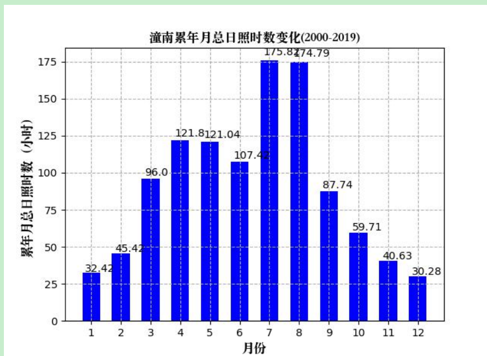
图 4.2.1-6 潼南月日照时数（单位：小时）
