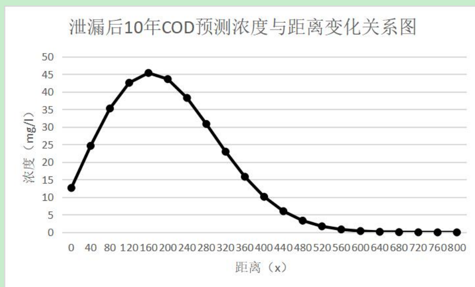
图4. 2. 3-1 COD浓度与距离变化关系图
