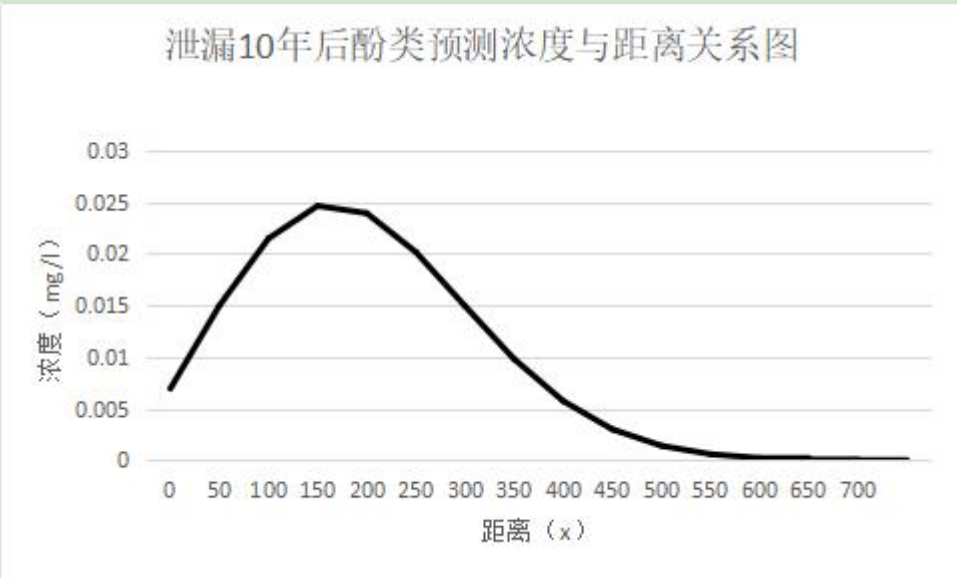
图4. 2. 3-3 挥发酚类浓度与距离变化关系图
