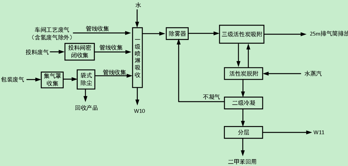
车间不含氢、乙醇废气处理工艺
