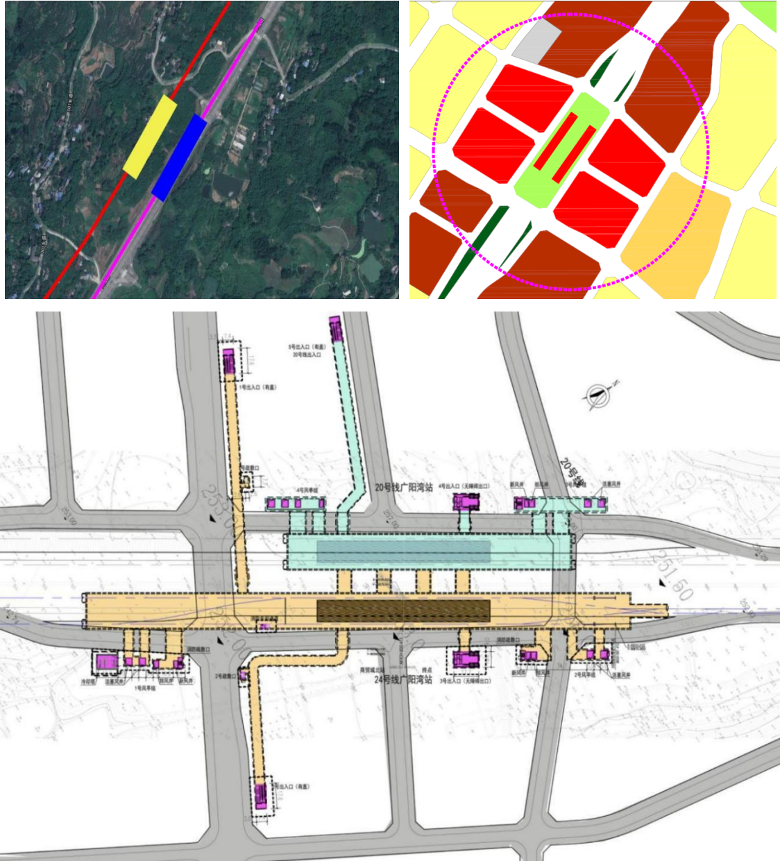
图 2.1-22 广阳湾站周边规划、平面布置图
