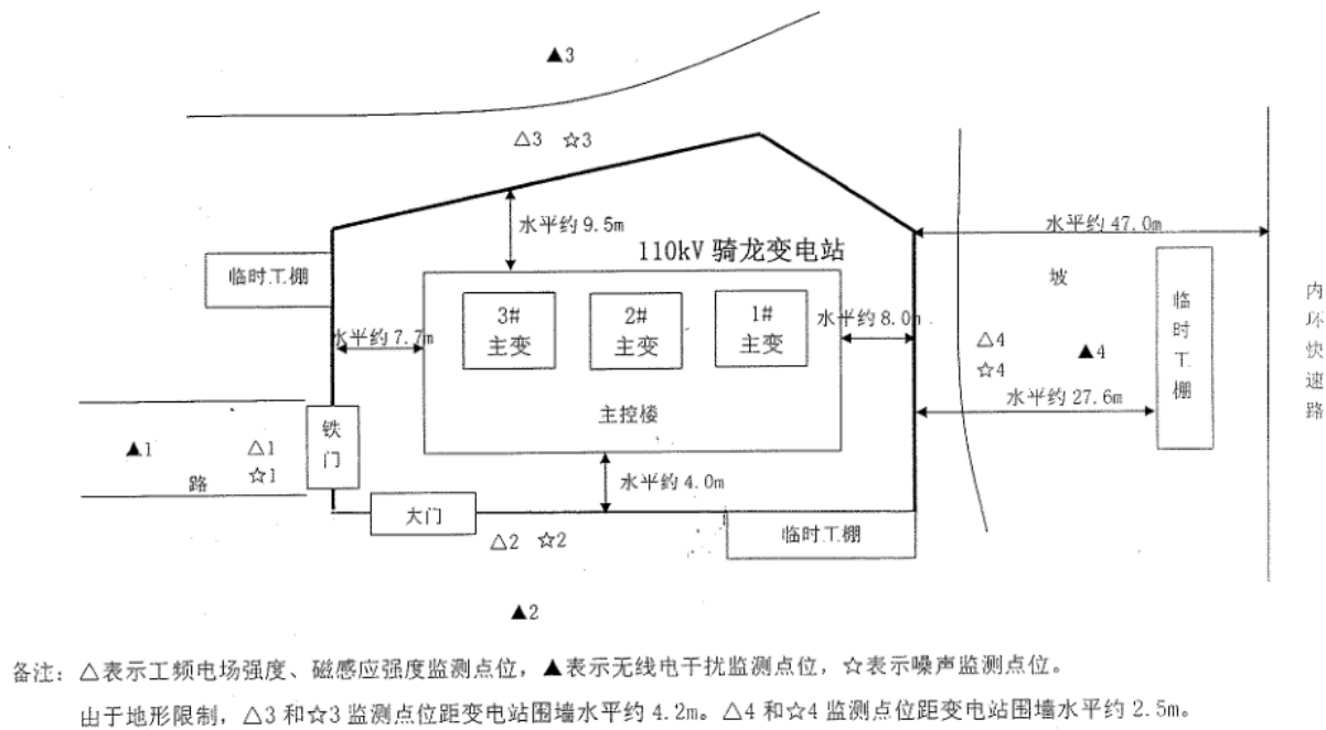
图 5.8-4 110kV 骑龙变电站电磁环境监测布点示意图
