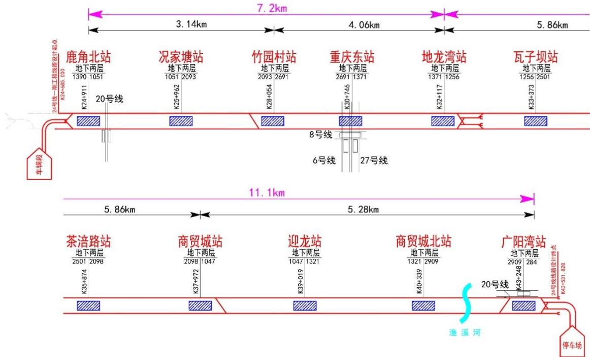
图 2.1-29 24 号线一期工程配线图
