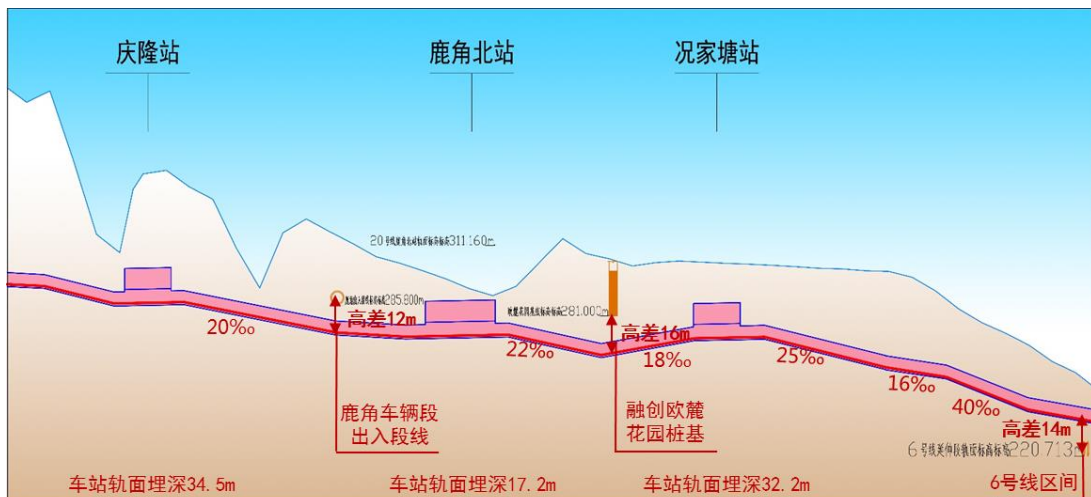
图 2.1-7 庆隆站～况家塘站段线路纵断面图
