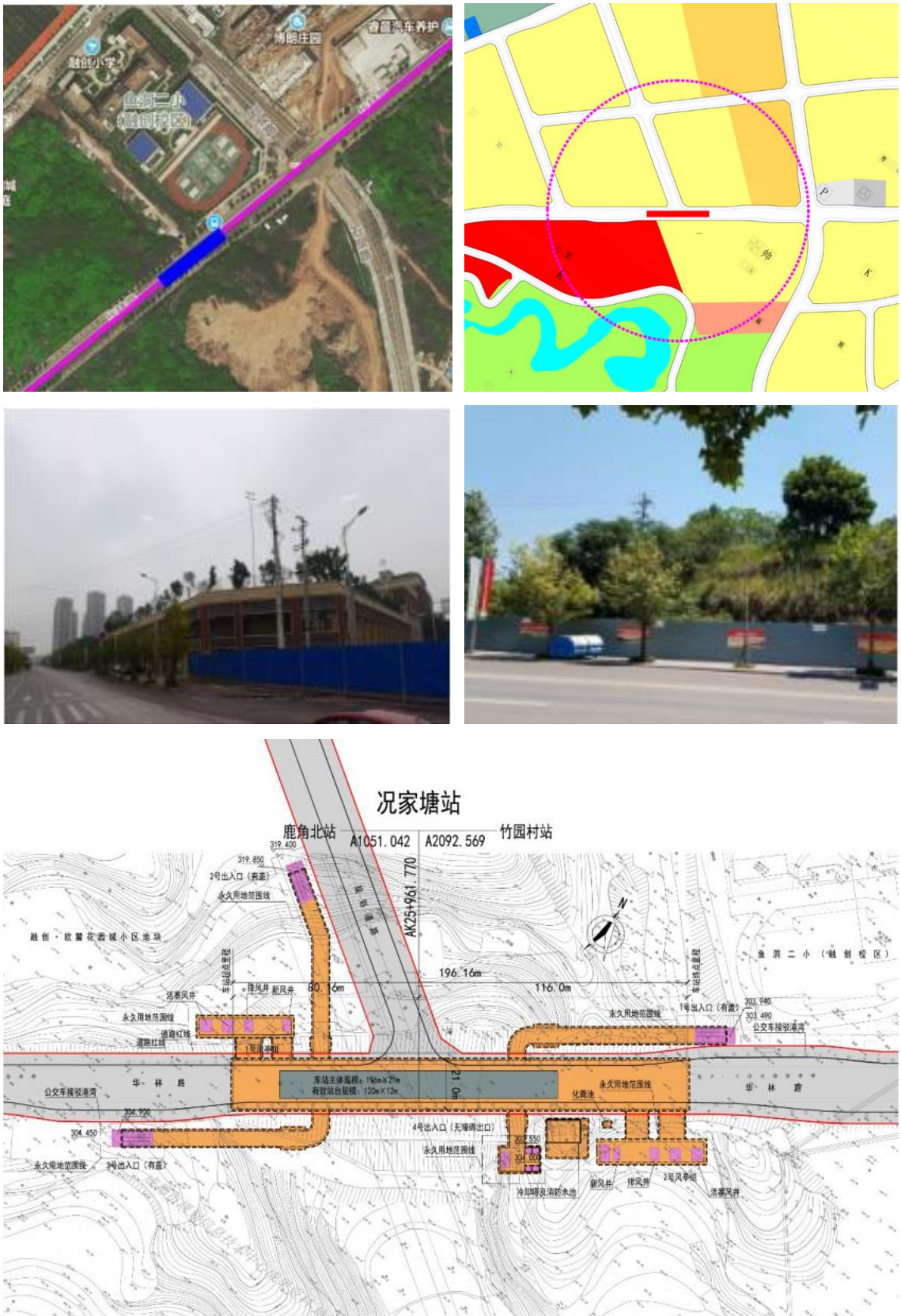
图 2.1-13 况家塘站周边规划、平面布置图
