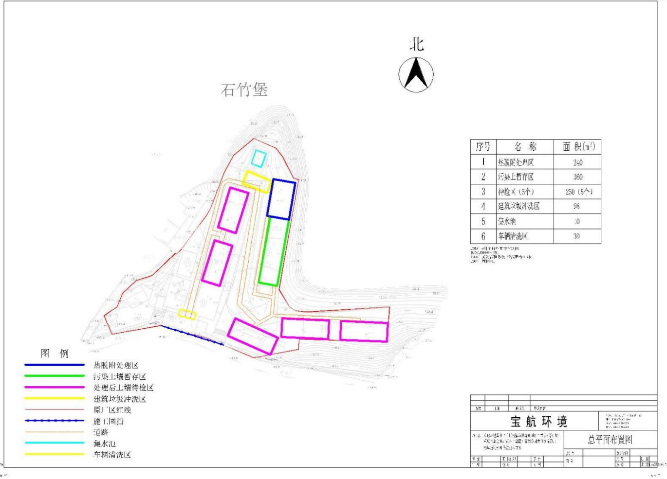
图 1.2-2 施工平面布置图
