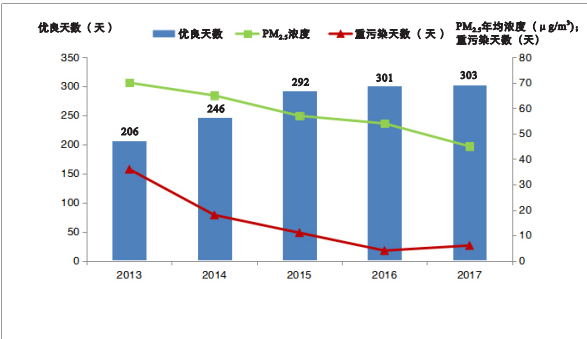
图2 2013~2017年重庆市空气质量状况变化趋势
