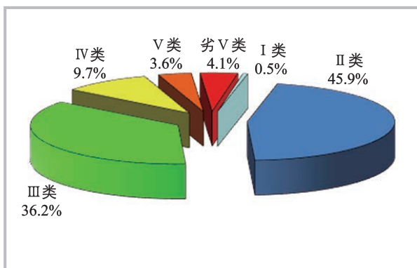
图1 2017年长江支流水质类别分布
